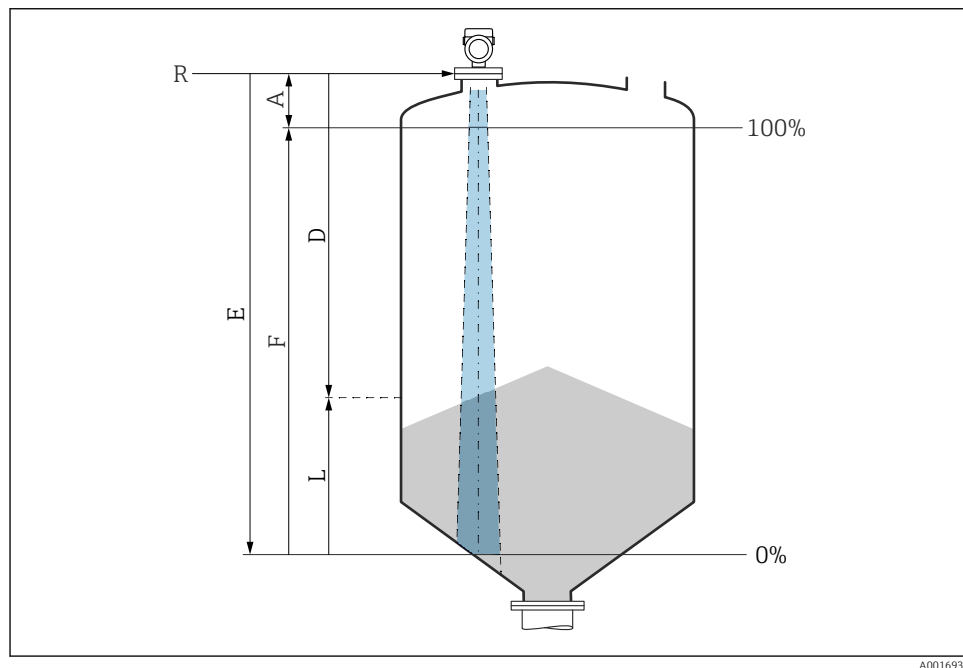
19 Konfigurasjonsparametere for nivåmåling i bulkfaststoffer
