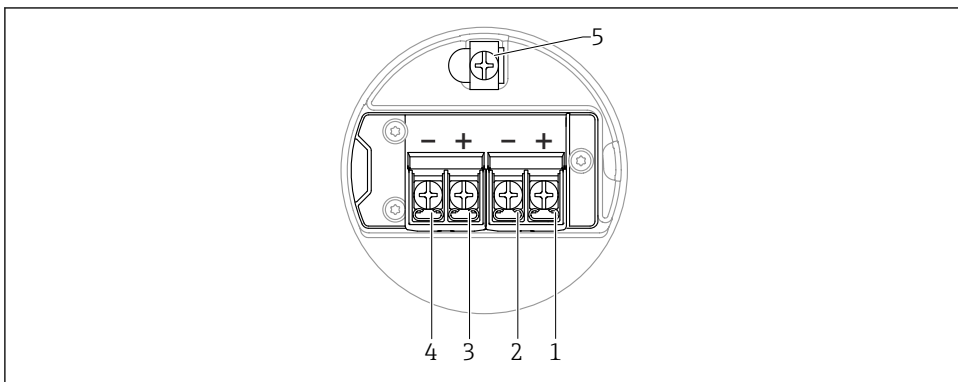
11 Klemmetilordning i tilkoblingsrom; 4 – 20 mA HART, bryterutgang, hus med dobbeltrom
