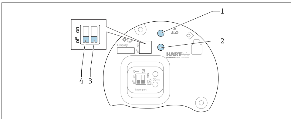
15 Betjeningstaster og DIP-brytere på HART-elektronikkinnsetsen
