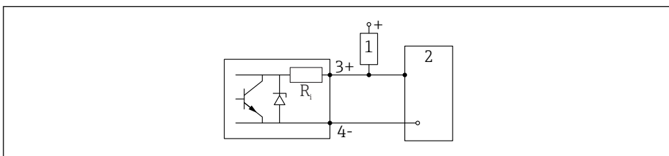
6 Tilkoblingseksempel for den digitale inngangen
