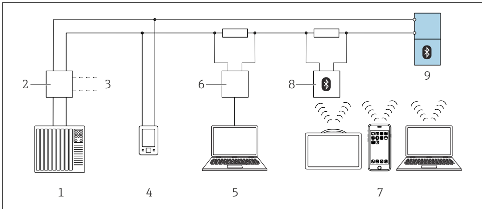
18 Alternativer for fjernbetjening via HART-protokollen
