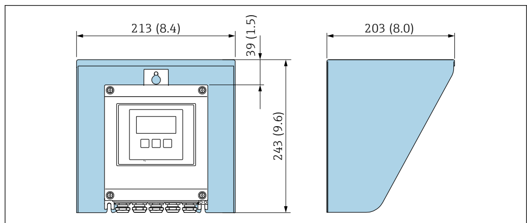
图 19 防护罩 (Proline 500 (数字式)) ; 单位: mm (in)
