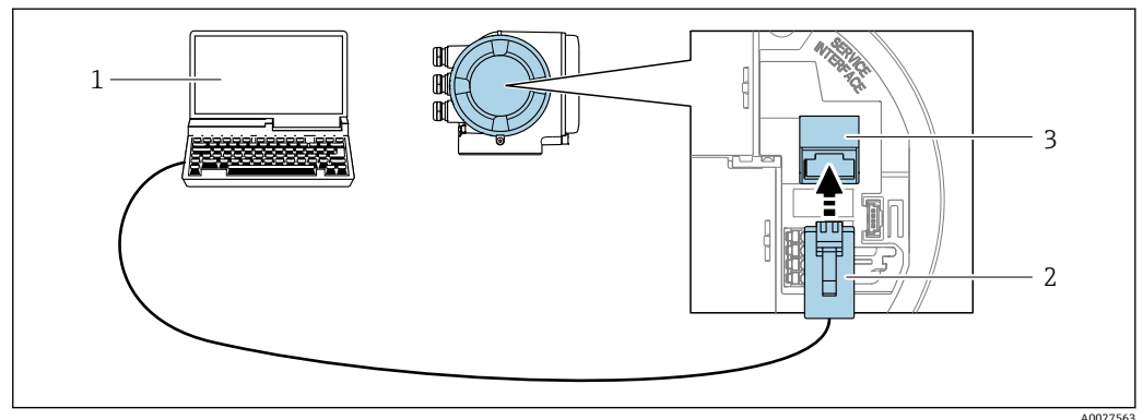
图 53 通过服务接口 (CDI-RJ45) 连接
