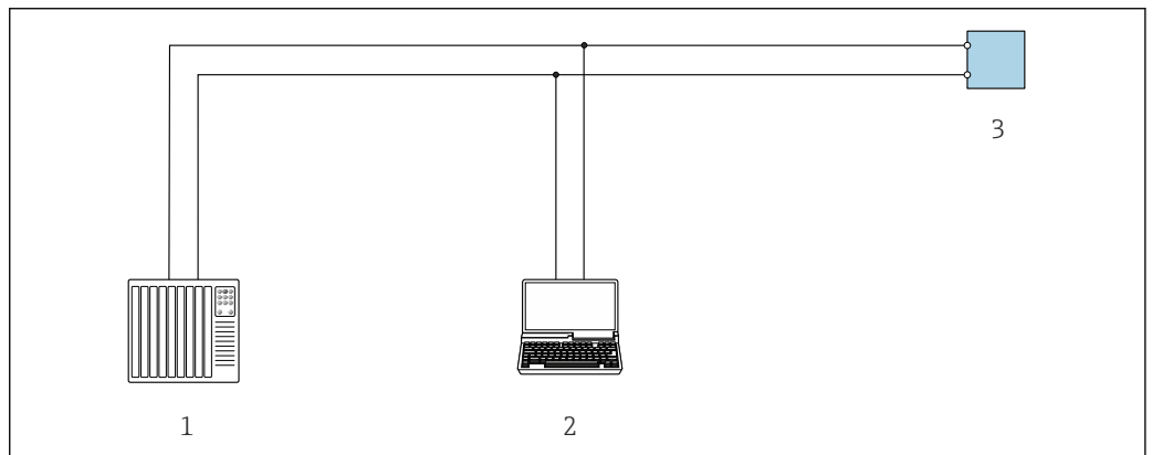
45 通过 Modbus RS485 通信进行远程操作（有源信号）
