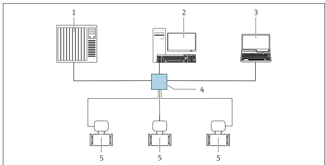
图 51 通过 Modbus TCP + Ethernet 进行远程操作 - 100 Mbit/s: 星形拓扑结构
