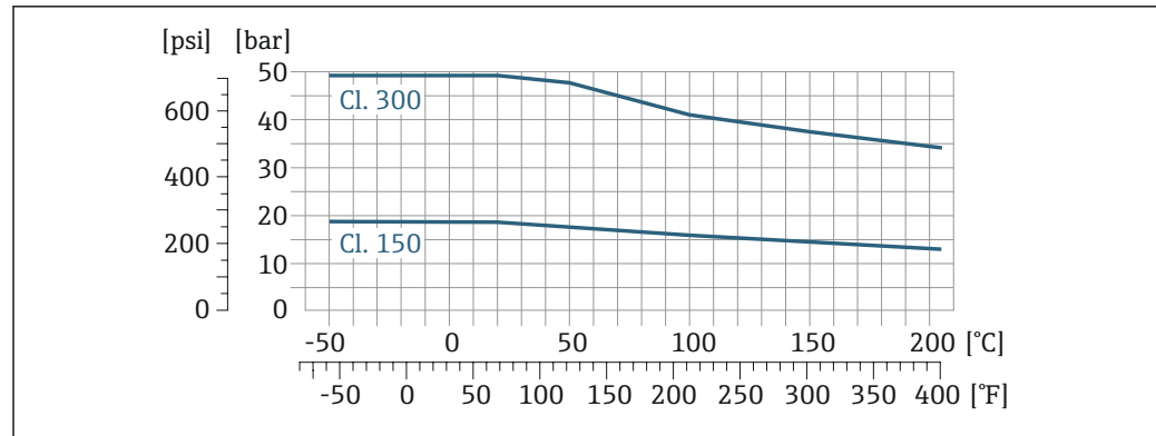
图 23 法兰材质: 1.4301 (304) ; 接液部件材质: 锆 702、钽
