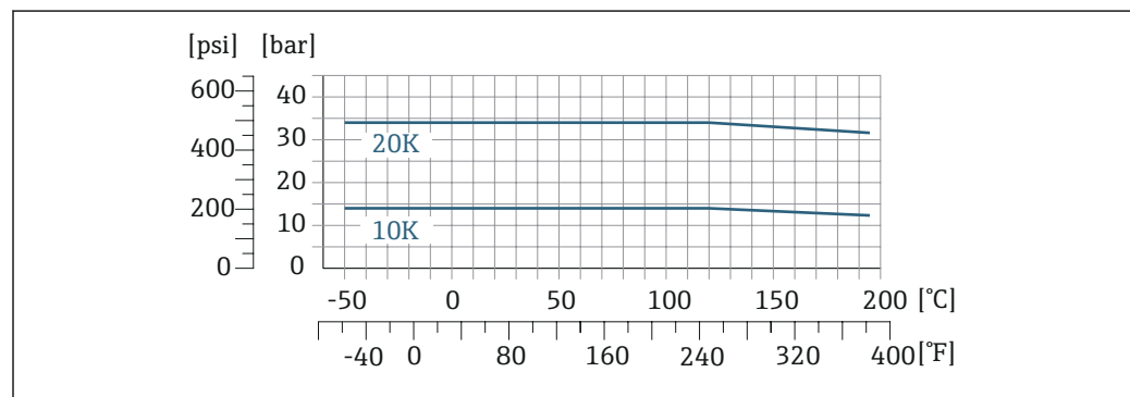
图 24 法兰材质: 1.4301 (304) ; 接液部件材质: 锆 702、钽
