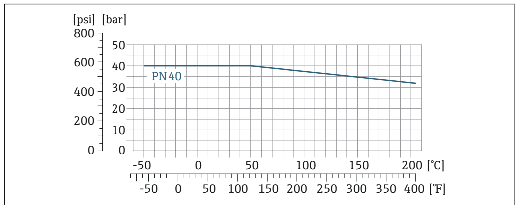
图 22 法兰材质: 1.4301 (304) ; 接液部件材质: 锆 702、钽
