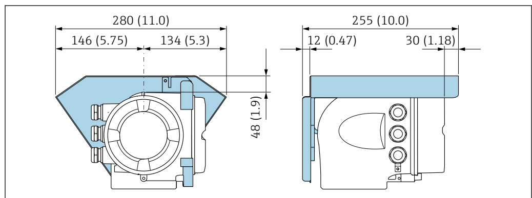
图 20 防护罩 (Proline 500) ; 单位: mm (in)
