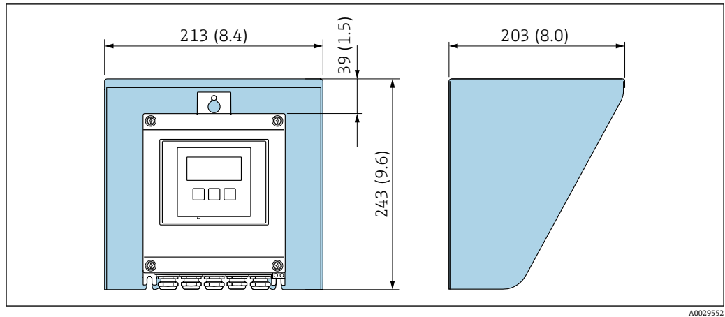
图 26 防护罩 (Proline 500 (数字式)) ; 单位: mm (in)
