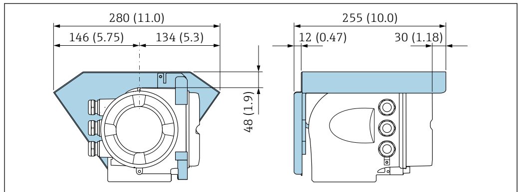
图 27 防护罩 (Proline 500) ; 单位: mm (in)
