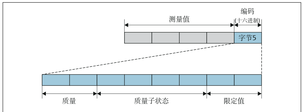
图 37 状态字节结构
