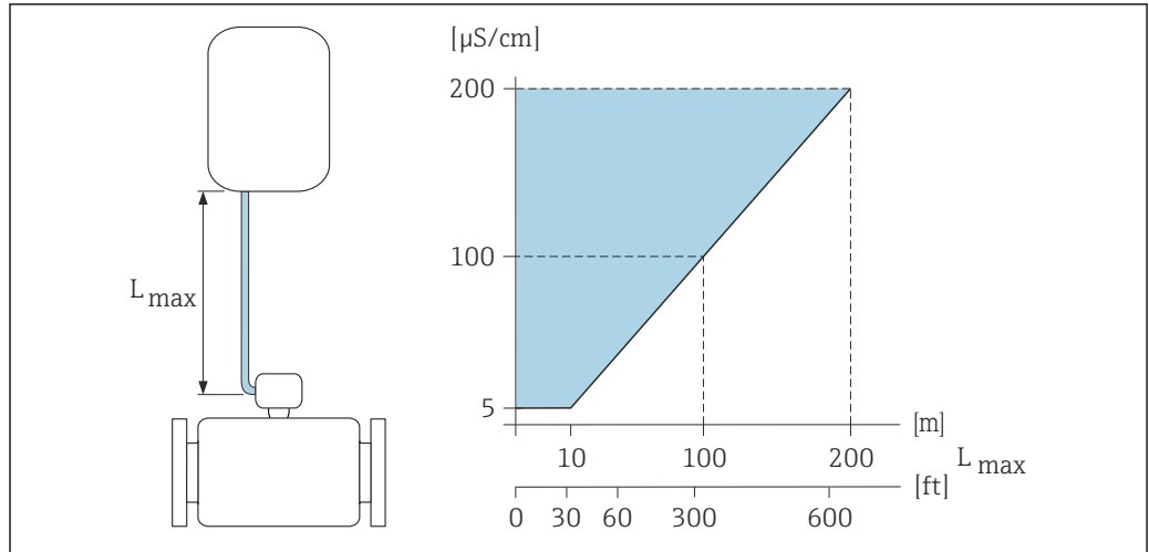
图 6 允许连接电缆长度 彩色区域 = 允许电缆长度范围 L_{max} = 连接电缆长度 ([m] ([ft]) ) [\mu S/cm] = 介质电导率
