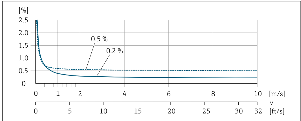
图 40 最大测量误差 (% o.r.)
