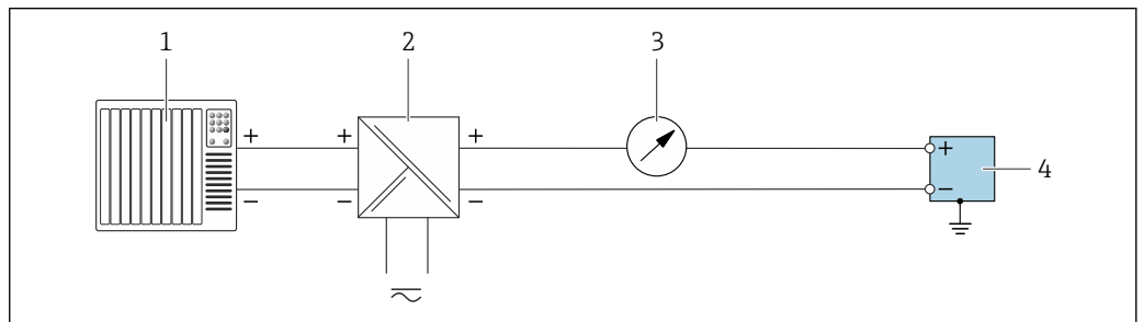
图 19 接线实例：4 ... 20 mA 电流输出 (无源)
