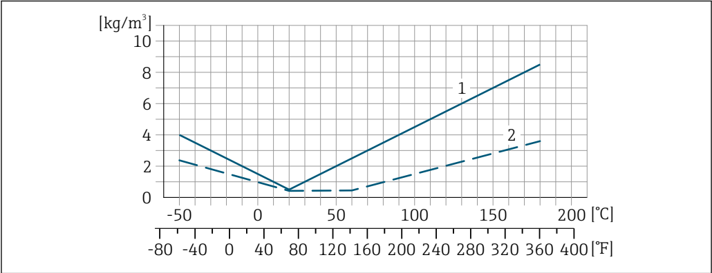
1 Ajuste en campo de la densidad, p. ej., a +20 °C (+68 °F) 2 Calibración de densidad ampliada
