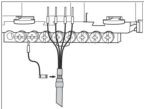
🔗 10 Podłączenie uziemienia funkcjonalnego
