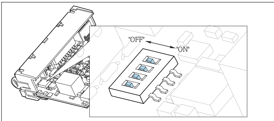
31 Mikroprzełączniki do wewnętrznej terminacji magistrali
