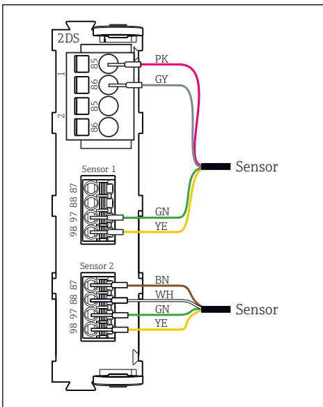
13 Podłączenie czujników z dodatkowym zasilaniem lub bez dodatkowego zasilania do modułu 2DS
