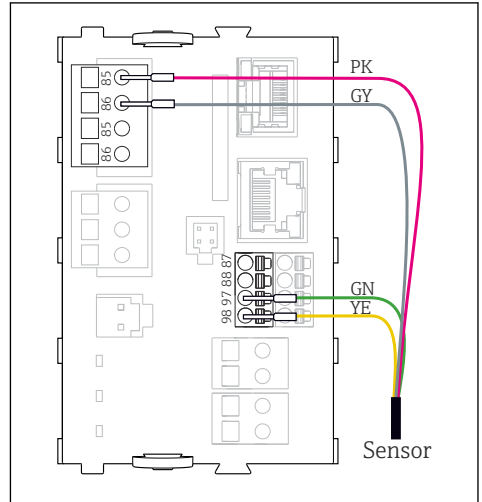
12 Czujniki z dodatkowym zasilaniem
