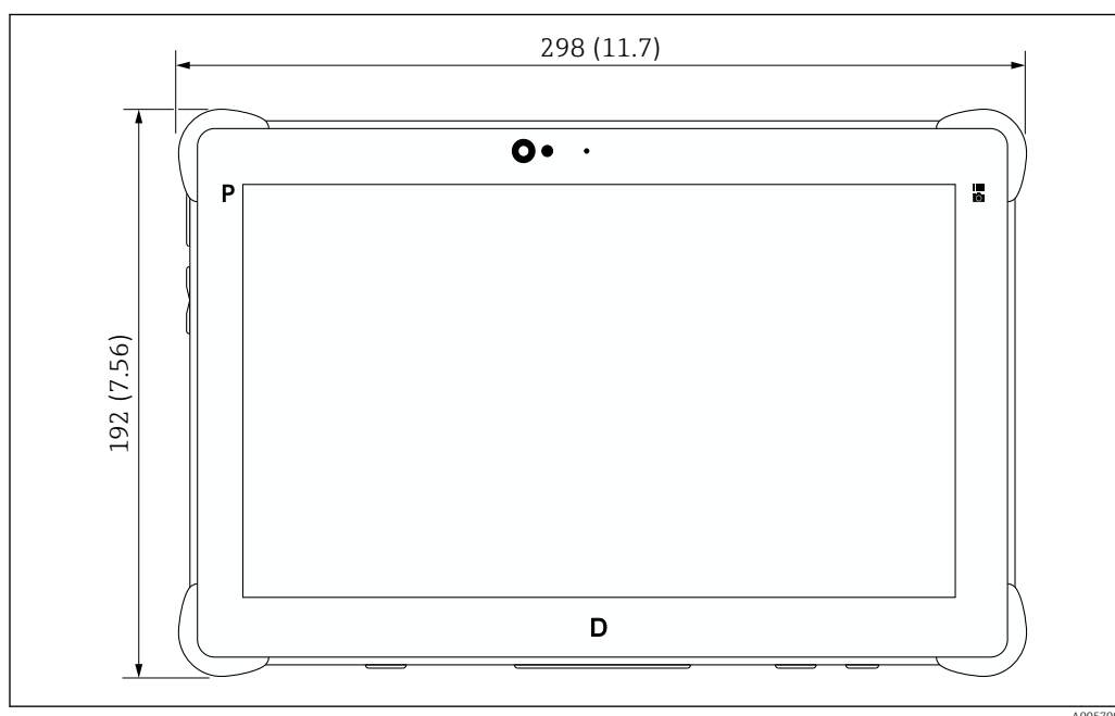
10 Vista frontal. Unidad de medida mm (in)
