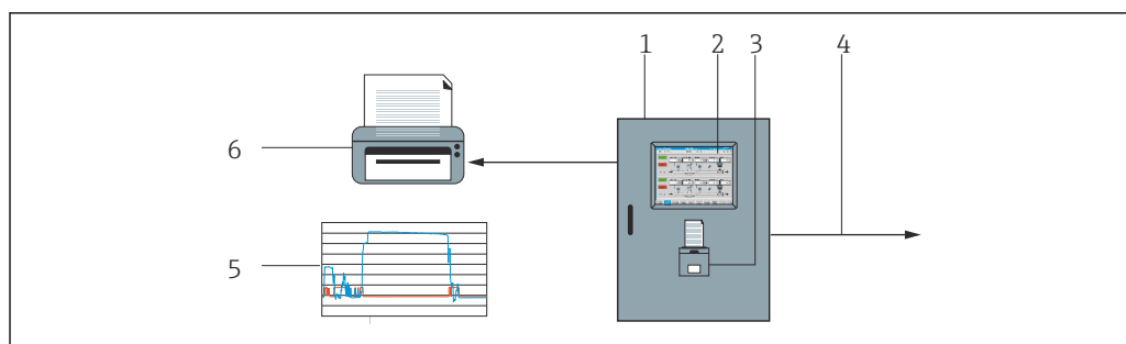
1 Übersicht Bunker-Computer
