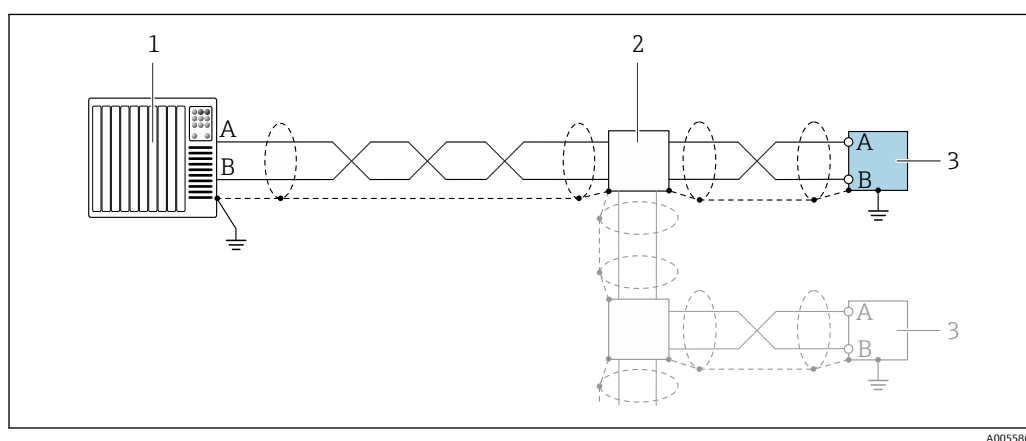
11 接线实例: Modbus RS485
