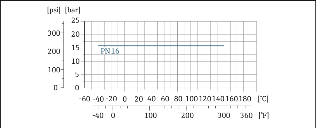
34 过程连接材质：不锈钢 1.4404 (F316L)
