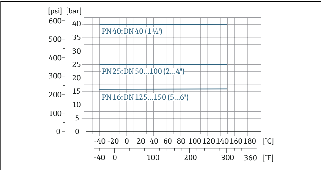
图 36 过程连接材质: 不锈钢 1.4404 (F316L)
