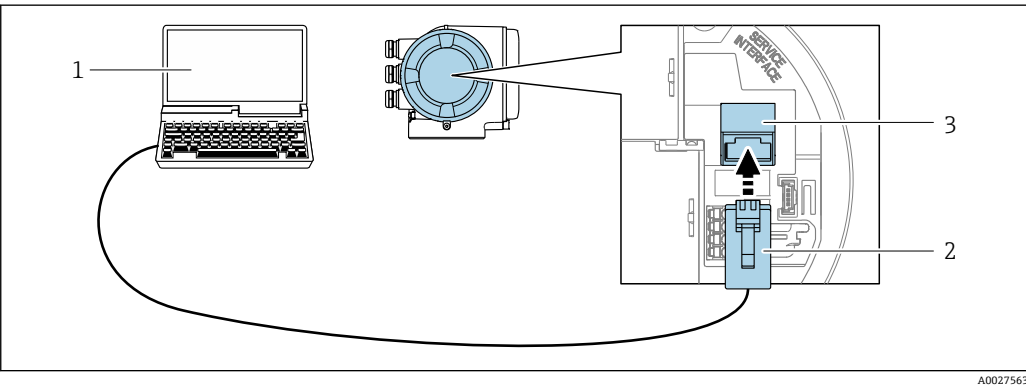
图 75 通过服务接口 (CDI-RJ45) 连接
