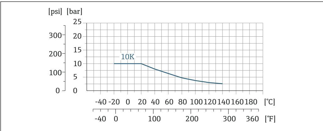
32 过程连接材质: PVDF
