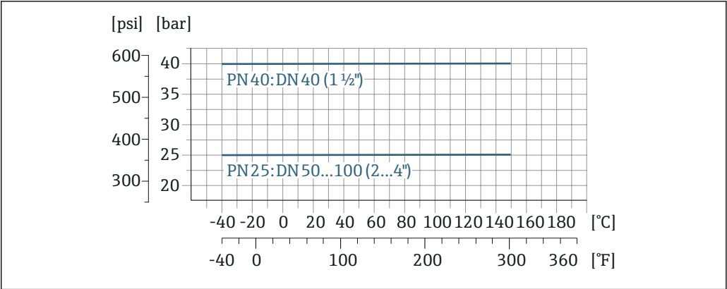
38 过程连接材质: 不锈钢 1.4404 (F316L)
