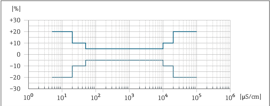
15 测量误差 (可选: 订购选项“电导率测量标定”，选型代号 CW)
