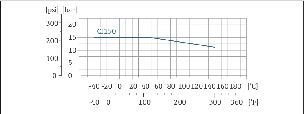
29 过程连接材质: 不锈钢 1.4404 (F316L)
