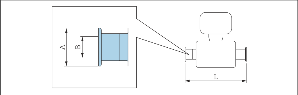
图 59 卫生型卡箍，适用带 ASME BPE 接头的管道（缩径）
