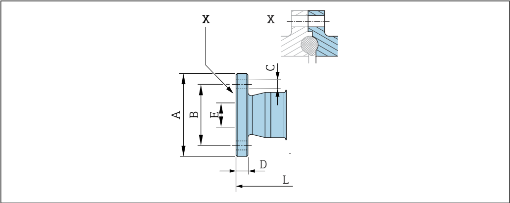
44 部件 X: 非对称过程连接; 蓝色部分由供应商提供。
