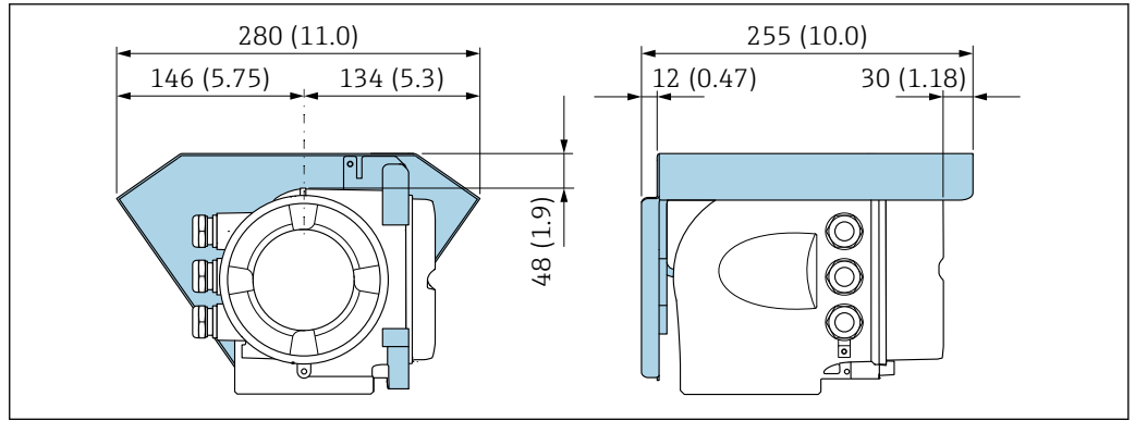
46 防护罩 (Proline 500) ; 单位: mm (in)
