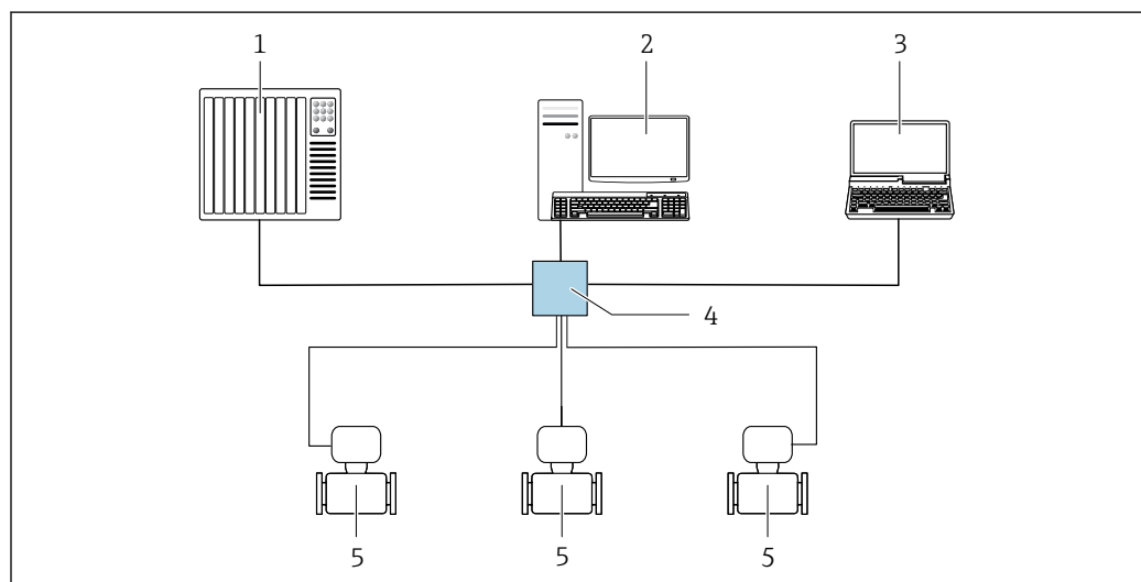
图 73 通过 Modbus TCP + Ethernet 进行远程操作 - 100 Mbit/s: 星形拓扑结构
