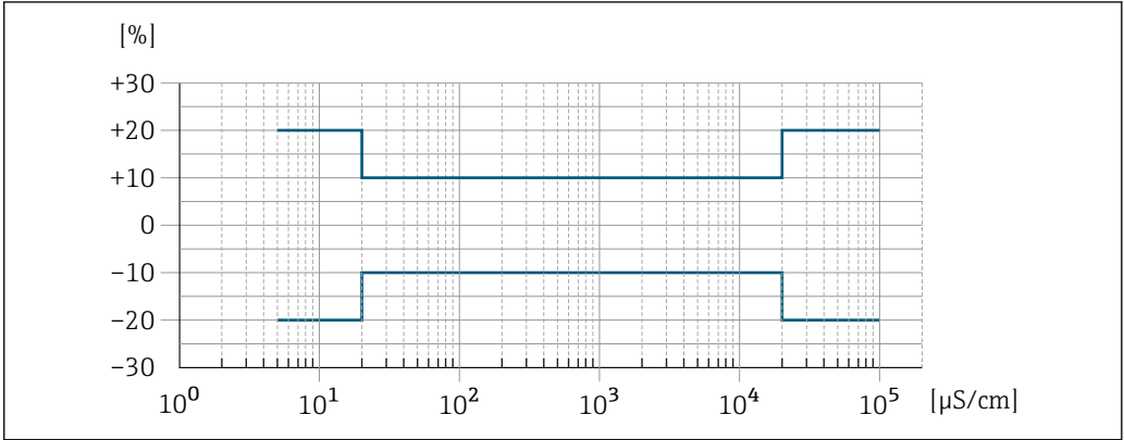
14 测量误差 (标准)
