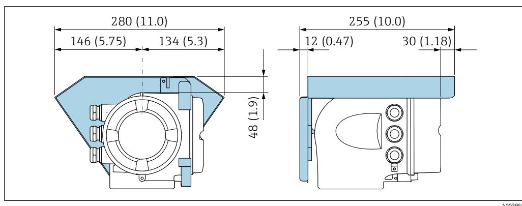
图 54 防护罩 (Proline 500) ; 单位: mm (in)
