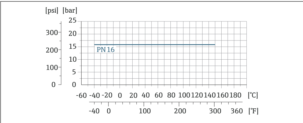
33 过程连接材质: 不锈钢 1.4404 (F316L)
