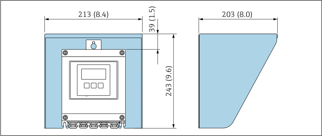
45 防护罩 (Proline 500 (数字式) ) ; 单位: mm (in)
