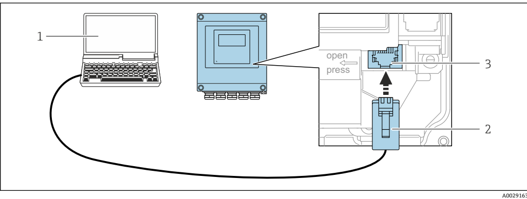
图 74 通过服务接口 (CDI-RJ45) 连接
