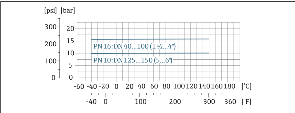
图 37 过程连接材质: 不锈钢 1.4404 (F316L)
