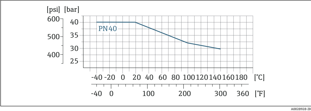
图 25 过程连接材质：不锈钢 1.4404 (F316L)
