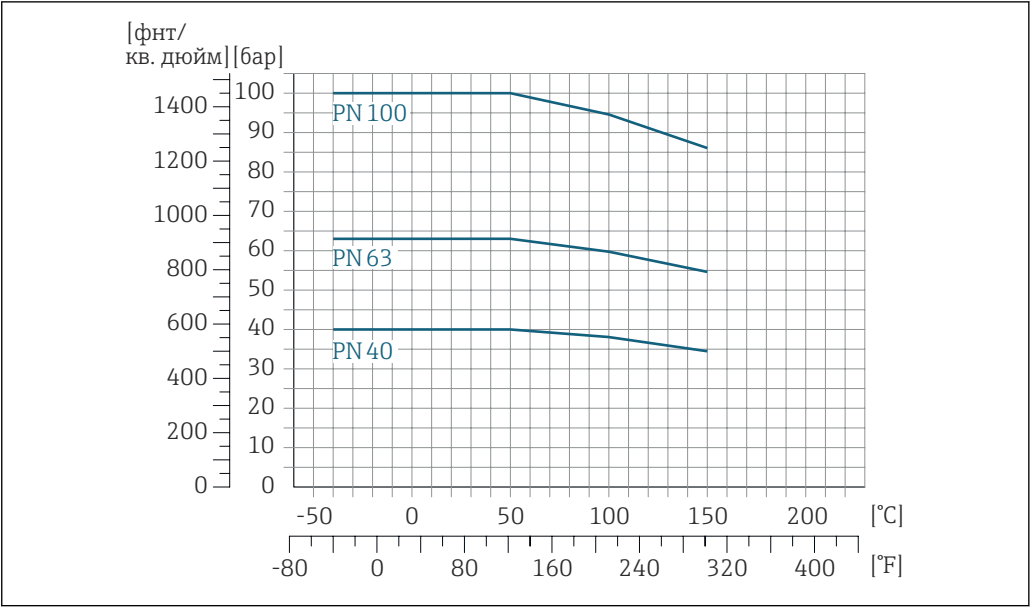
18 С материалом фланца 1.4404 (F316/F316L)
