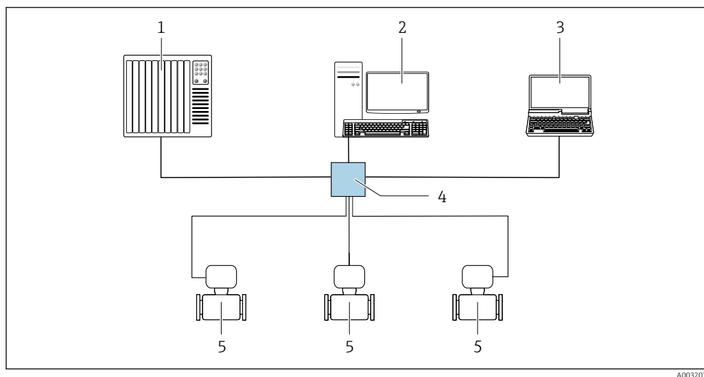
47 Варианты дистанционного управления по протоколу Modbus TCP посредством интерфейса Ethernet - 100 Мбит/с: топология «звезда»
