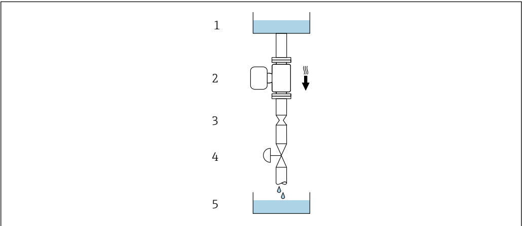
14 Монтаж в трубопроводе с нисходящим потоком (например, для дозирования)
