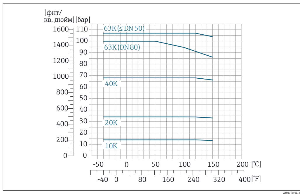
20 С материалом фланца 1.4404 (F316/F316L)
