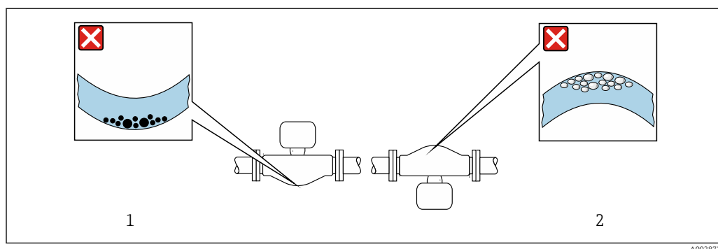
☒ 15 Монтажное положение датчика с изогнутой измерительной трубкой
