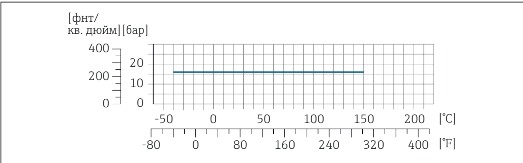
25 С материалом присоединения 1.4404 (316/316L)
