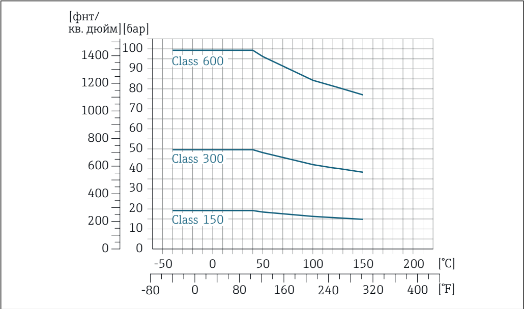
19 С материалом фланца 1.4404 (F316/F316L)
