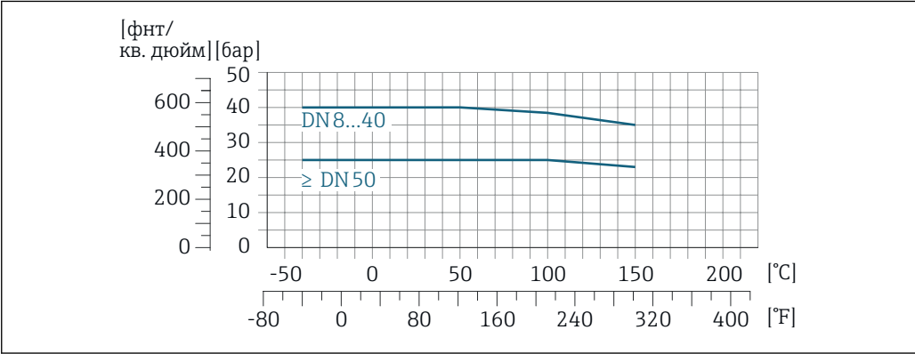
23 С материалом присоединения 1.4404 (316/316L)
