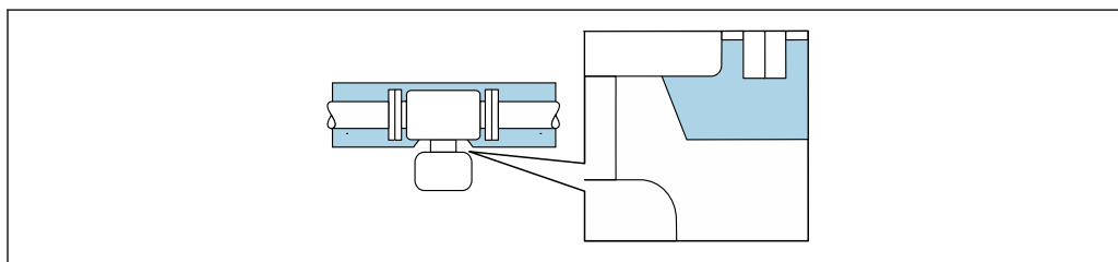
27 Теплоизоляция с открытой удлинительной шейкой
