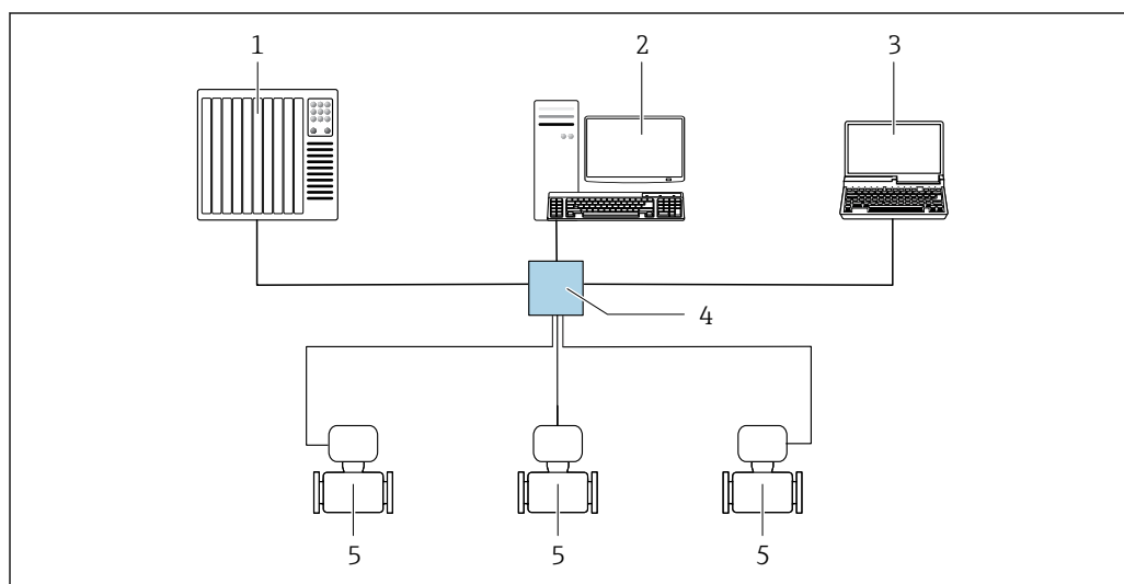
48 Варианты дистанционного управления через сеть EtherNet/IP: топология «звезда»
