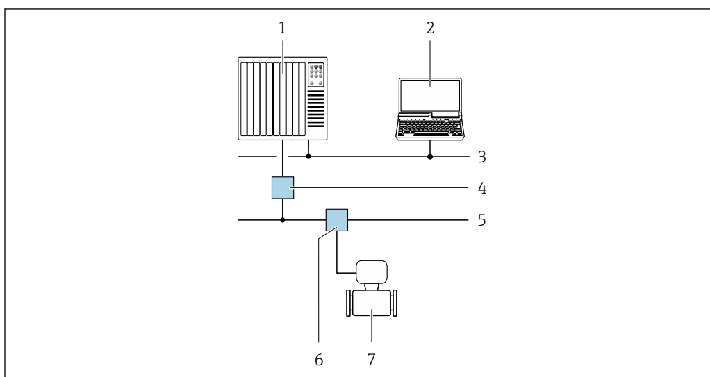
44 Варианты дистанционного управления по сети PROFIBUS PA
