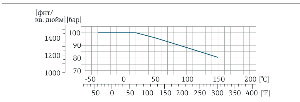
26 С материалом присоединения 1.4404 (316/316L)
