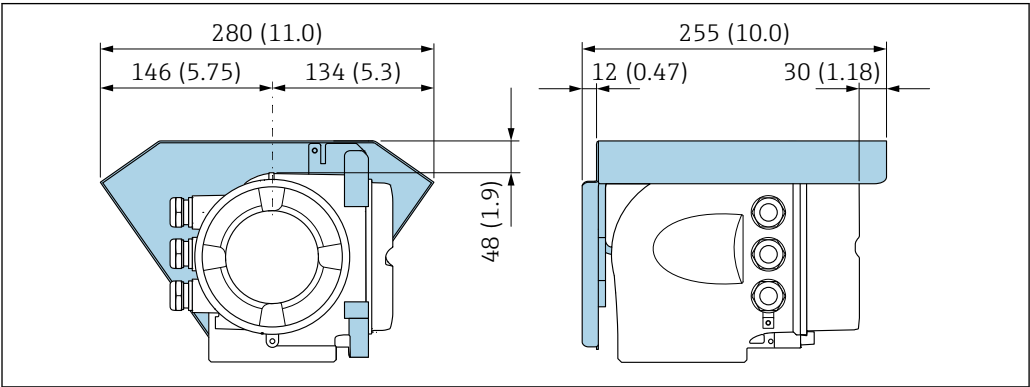
16 Ед. изм.: мм (дюймы)
