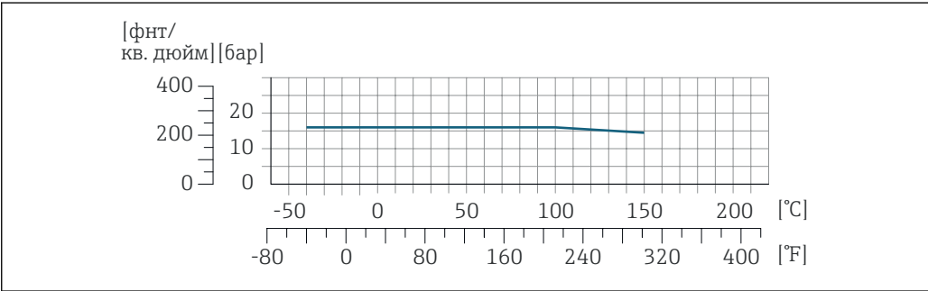
24 С материалом присоединения 1.4404 (316/316L)
