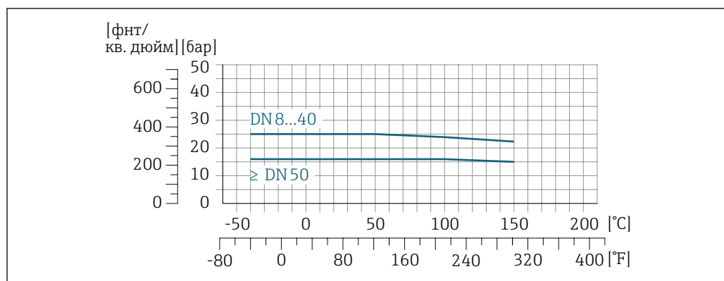
21 С материалом фланца 1.4404 (316/316L)
