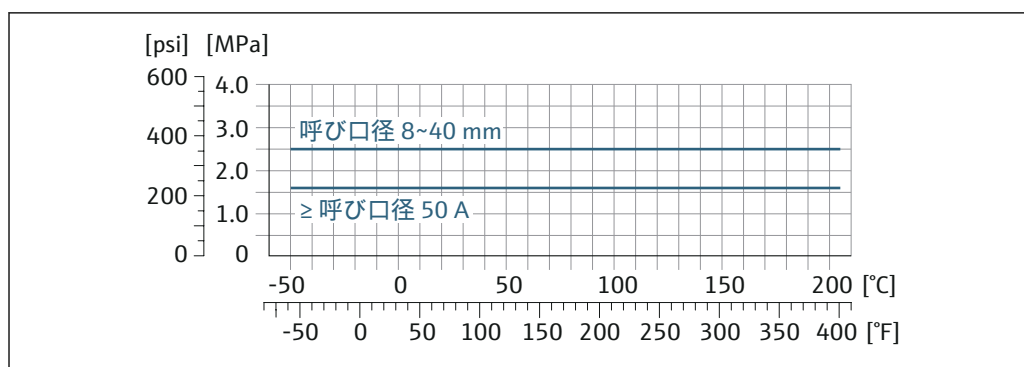
図 19 フランジ材質 1.4435 (SUS 316L 相当)
