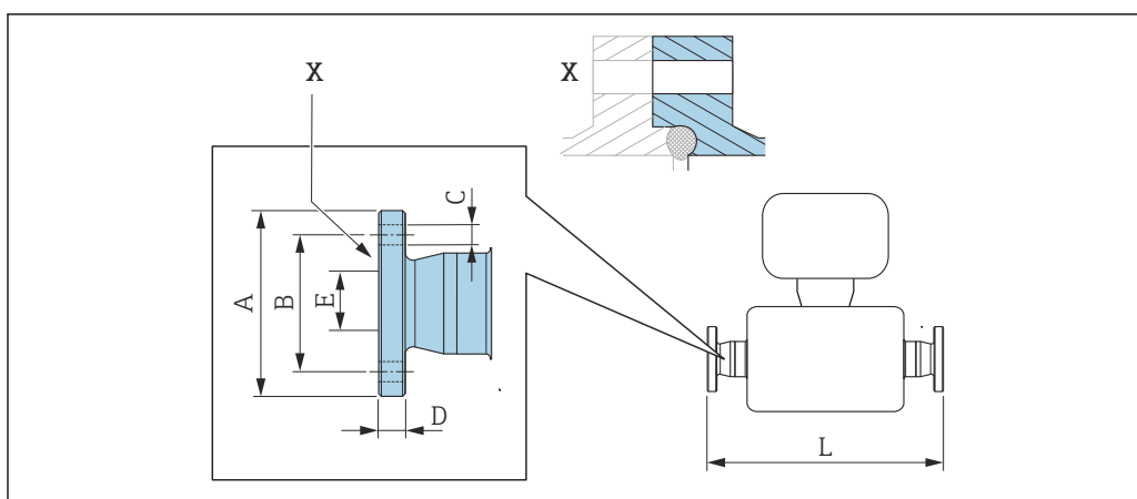
図 38 Xの詳細：非対称型プロセス接続；青色部分が供給されます。
