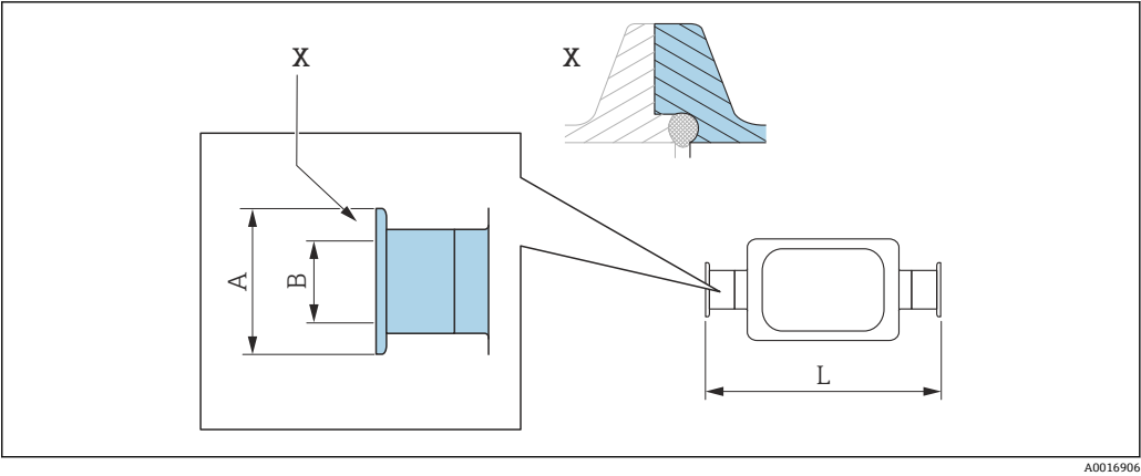
図 41 X の詳細：非対称型プロセス接続；着色部分が供給されます。
