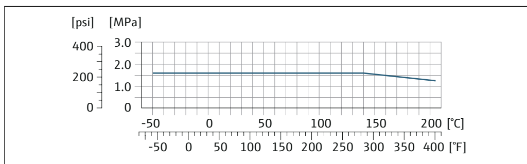
図 20 フランジ材質 1.4435 (SUS 316L 相当)
