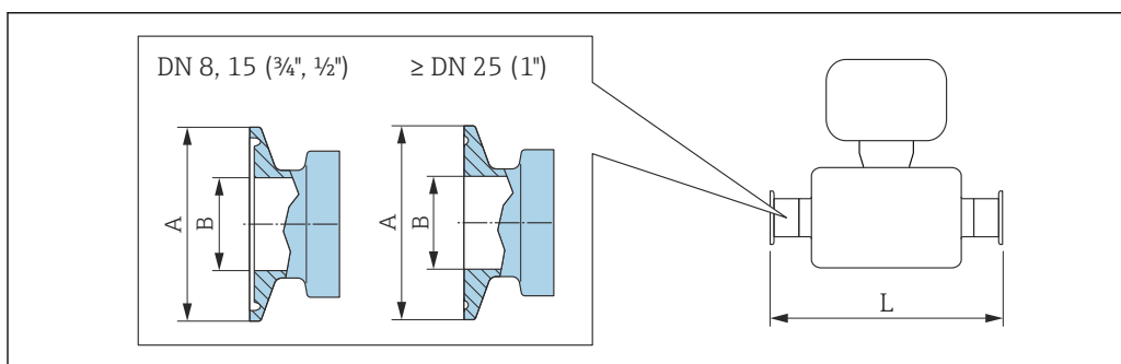
図 39 単位 mm (in)
