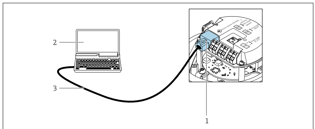
図 48 「出力」のオーダーコードの接続、オプション B：4～20 mA HART、パルス/周波数/スイッチ出力
