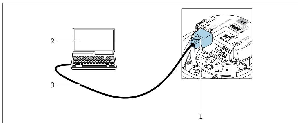
図 50 「出力」のオーダーコードの接続、オプション N : EtherNet/IP
