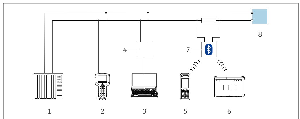
図 44 HART プロトコルを使用したリモート操作オプション
