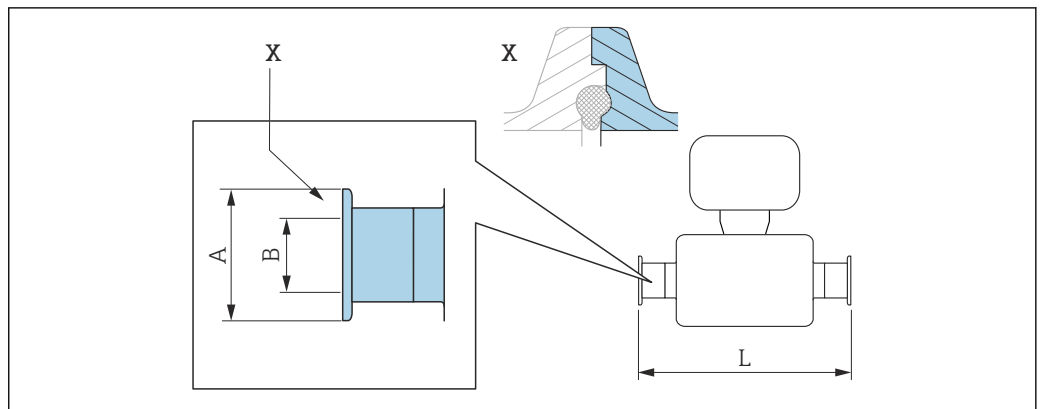
図 31 Xの詳細：非対称型プロセス接続；着色部分が供給されます。
