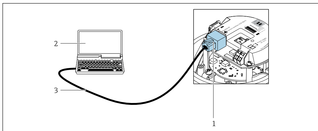
図 51 「出力」のオーダーコード、オプション R : PROFINET の接続
