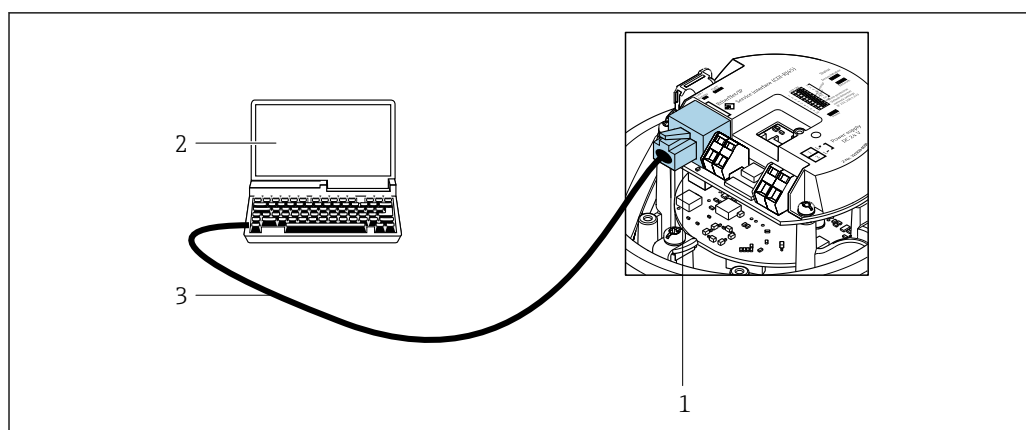
図 49 「出力」のオーダーコードの接続、オプション L : PROFIBUS DP
