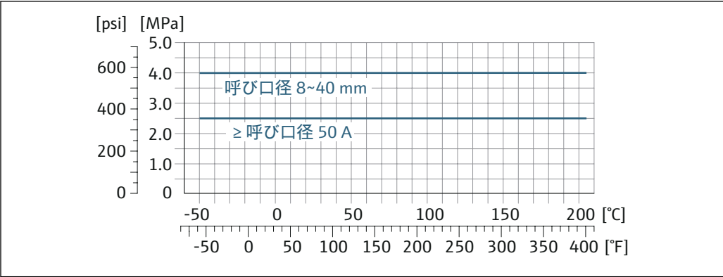
図 25 接続部の材質 1.4435 (SUS 316L 相当)
