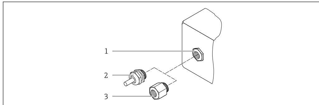
図 43 可能な電線口/ケーブルグランド
