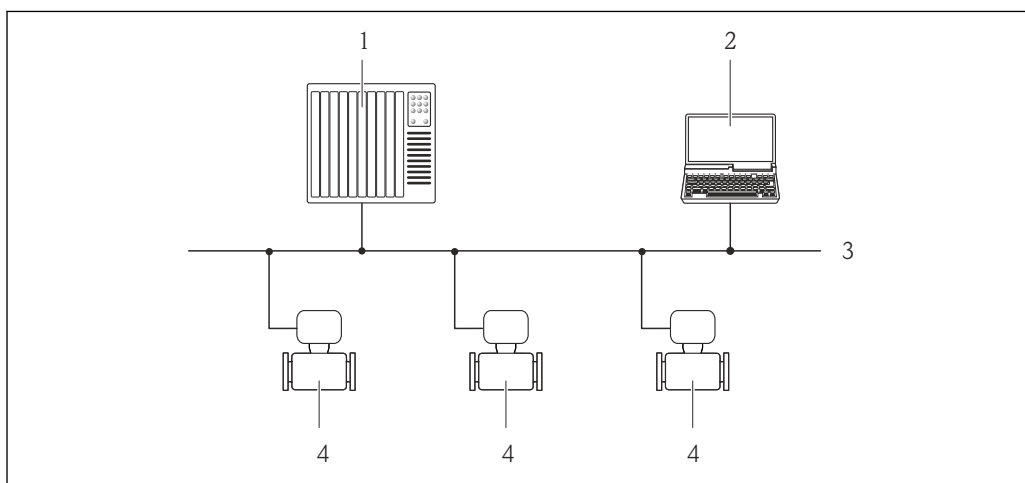
15 Opções para operação remota através da rede PROFIBUS DP
