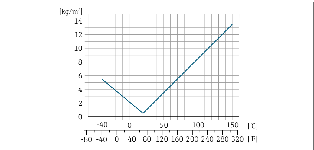
18 Ajuste da densidade de campo, por exemplo, a +20 °C (+68 °F)
