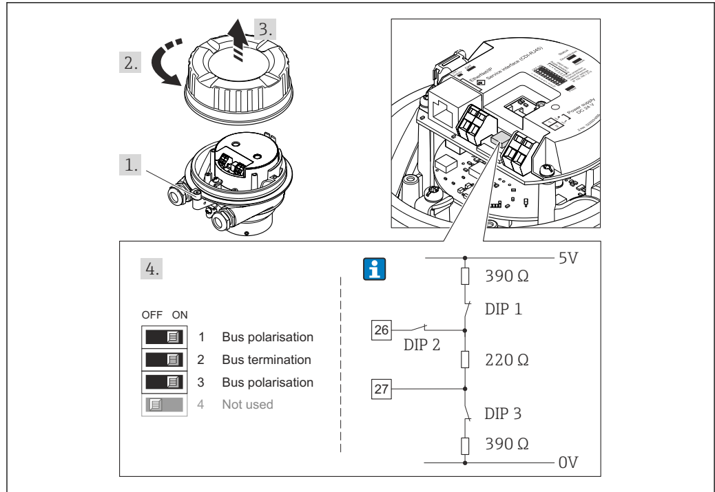
13 Finalização usando minisseletoras no módulo para componentes eletrônicos de E/S (para taxas de transferência < 1.5 MBaud)
