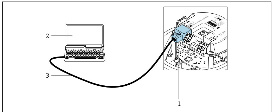
16 Conexão para o código de pedido para "Saida", opção L: PROFIBUS DP
