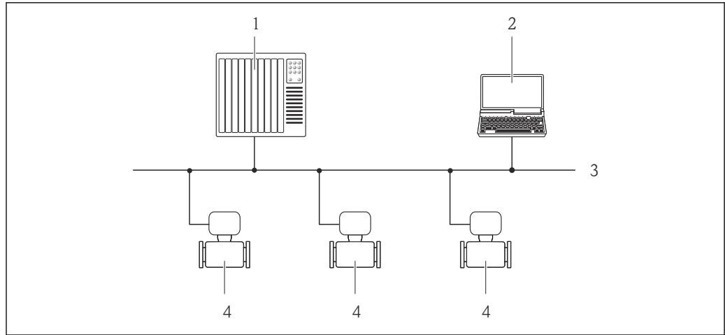
21 Opções para operação remota através da rede PROFIBUS DP
