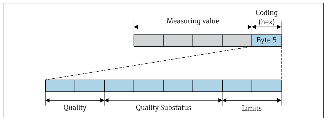
Fig. 17 Estrutura do byte de codificação
