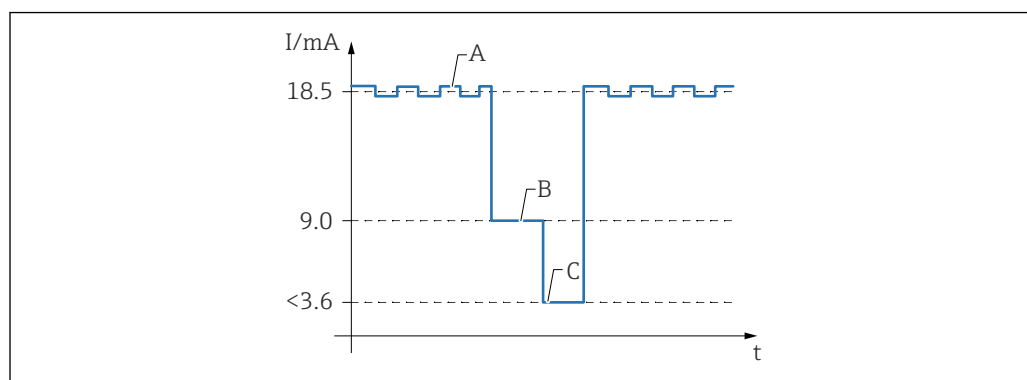
35 Процедура проведения функционального испытания для обнаружения минимального уровня
