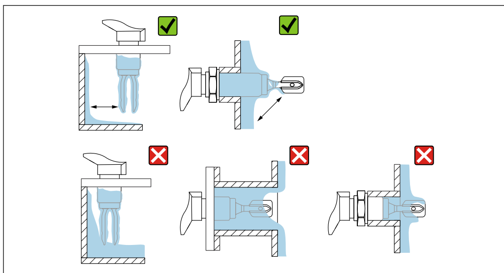
9 Примеры монтажа для технологической среды с высокой вязкостью
