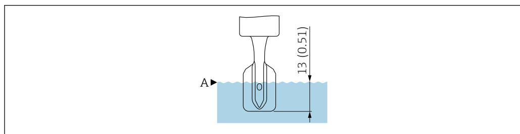
5 Точка переключения при стандартных рабочих условиях, вибрирующая вилка с пластиковым покрытием (ECTFE, PFA), размеры без учета толщины покрытия. Единица измерения мм (дюйм)
