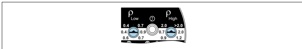
27 Недопустимое положение переключателя диапазона плотности в состоянии поставки
