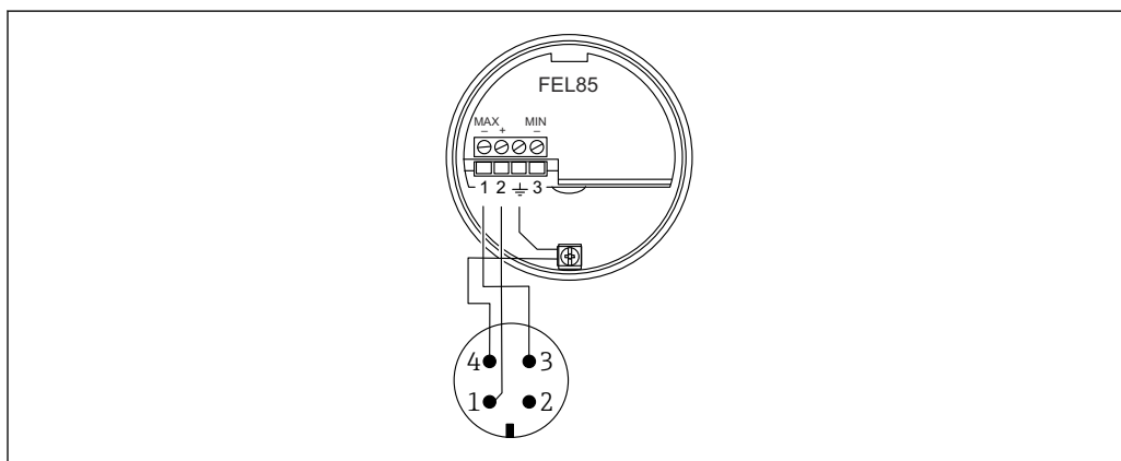
18 Назначение выводов с разъемом M12, режим работы с обнаружением максимального уровня
