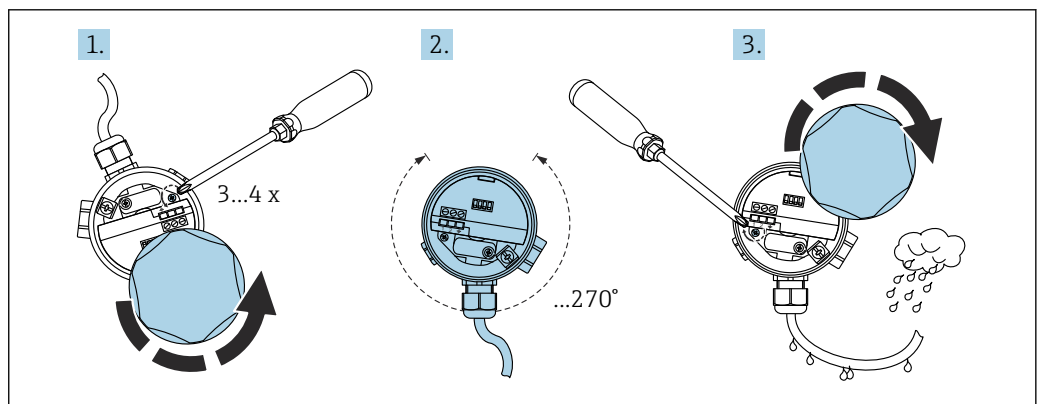
15 Корпус со стопорным винтом; образует ниспадающую каплеуловительную кабельную петлю
