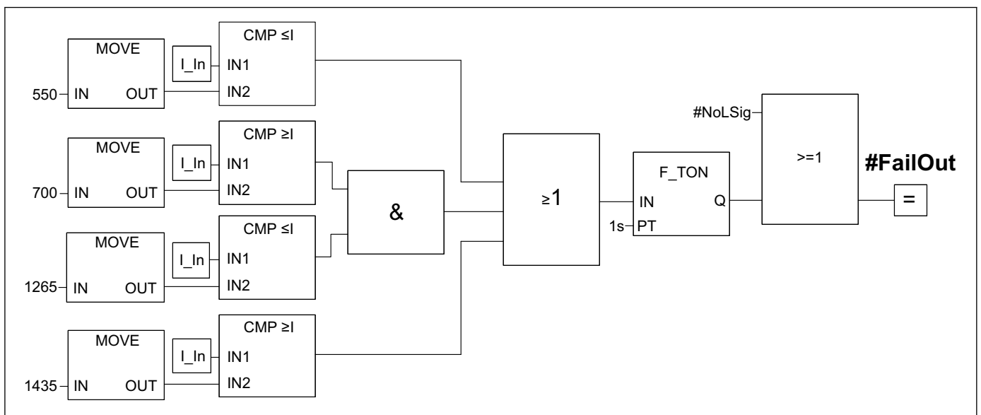
25 Функциональный модуль, анализ тока ошибки
