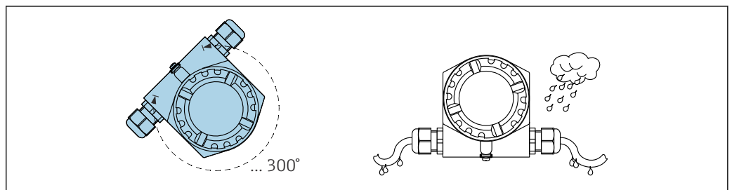
16 Корпус без установочного винта; образуйте ниспадающую каплеуловительную кабельную петлю
