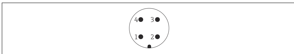
17 Назначение контактов разъема M12
