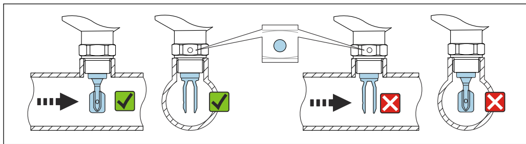
13 Монтаж в трубопроводах (следует учитывать положение вилки и отметку)
