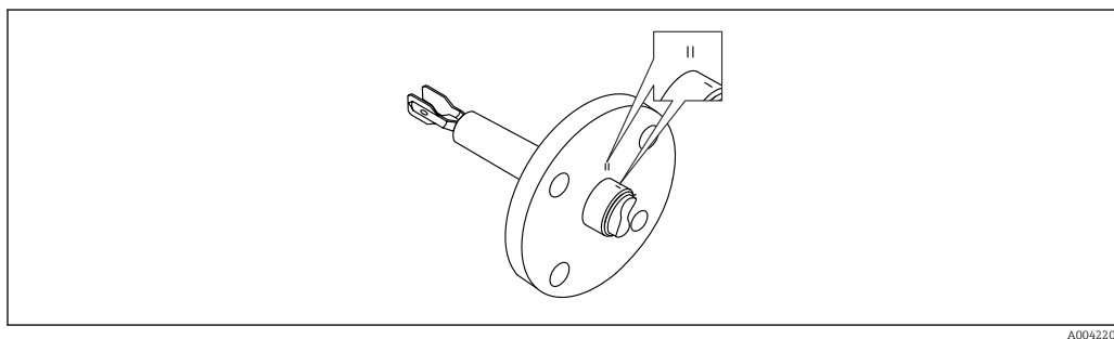
12 Положение вибрационной вилки при горизонтальном монтаже в резервуаре с использованием маркировки
