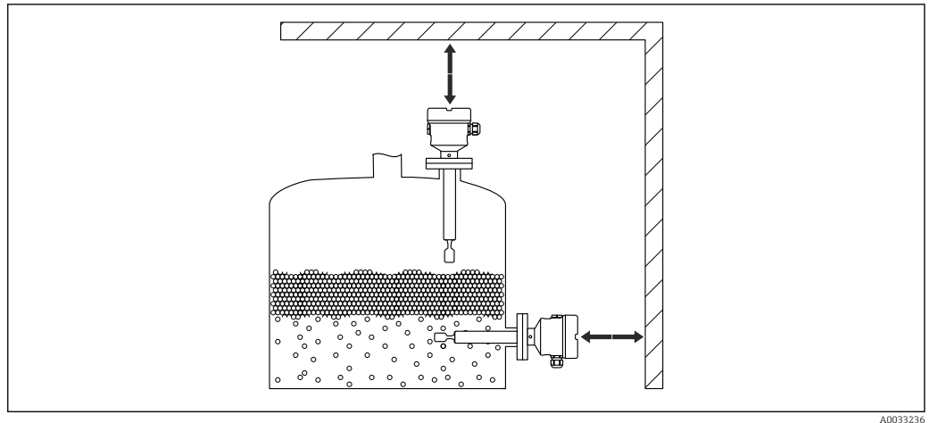
10 Учитывайте необходимое свободное пространство снаружи резервуара
