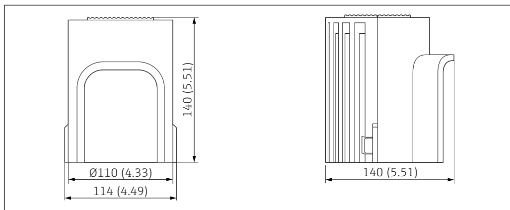
46 Размеры защитного козырька PBT. Единица измерения мм (дюйм)
