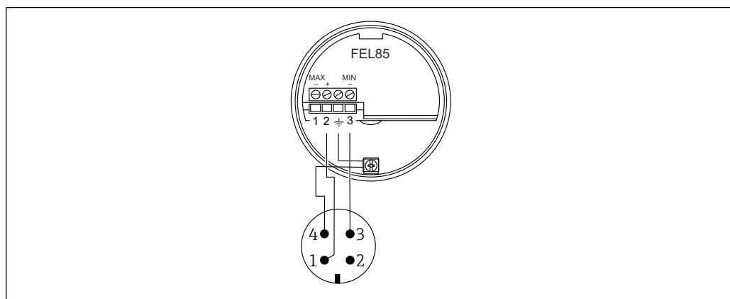
19 Назначение выводов с разъемом M12, режим работы с обнаружением минимального уровня
