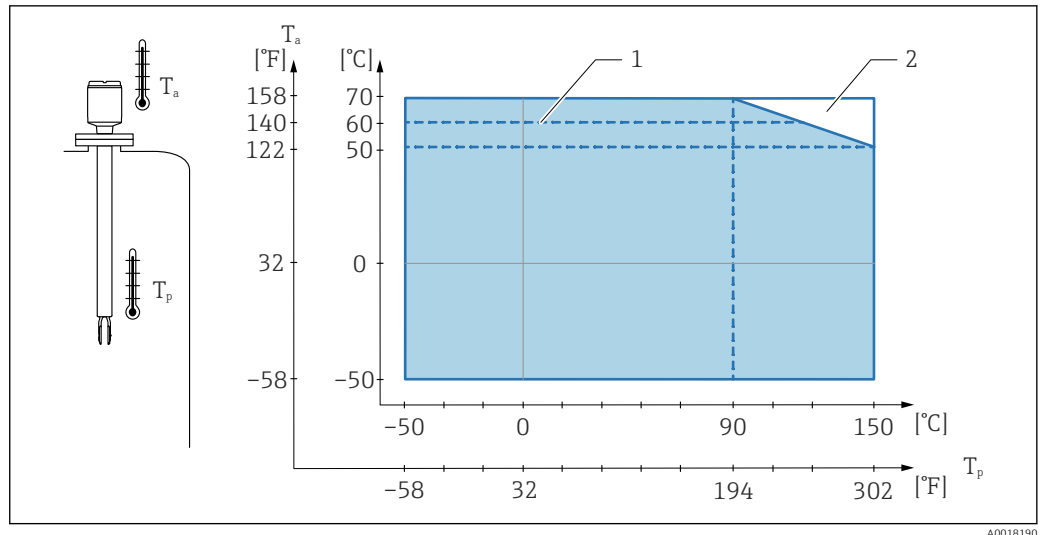
47 Зависимость допустимой температуры окружающей среды T_a в зоне корпуса от рабочей температуры T_p в резервуаре; максимальная температура технологического процесса 150\text{ }^{\circ}\text{C} ( 302\text{ }^{\circ}\text{F} )
