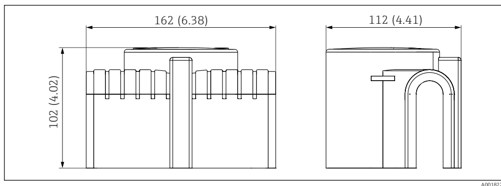
45 Размеры защитного козырька от погодных условий PA6. Единица измерения мм (дюйм)
