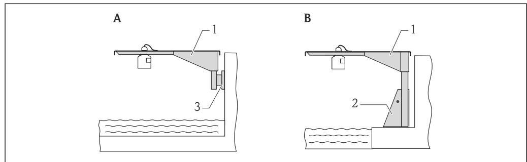
13 Montage du capteur avec bras de montage
