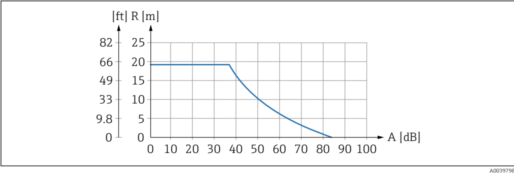
2 Diagramme de portée pour les capteurs à ultrasons
