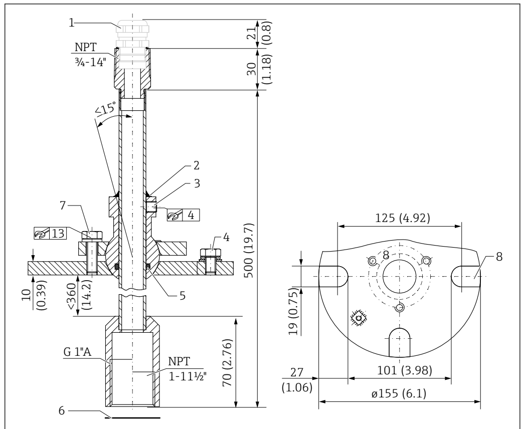
20 Dispositif d'orientation FAU40. Unité de mesure mm (in)
