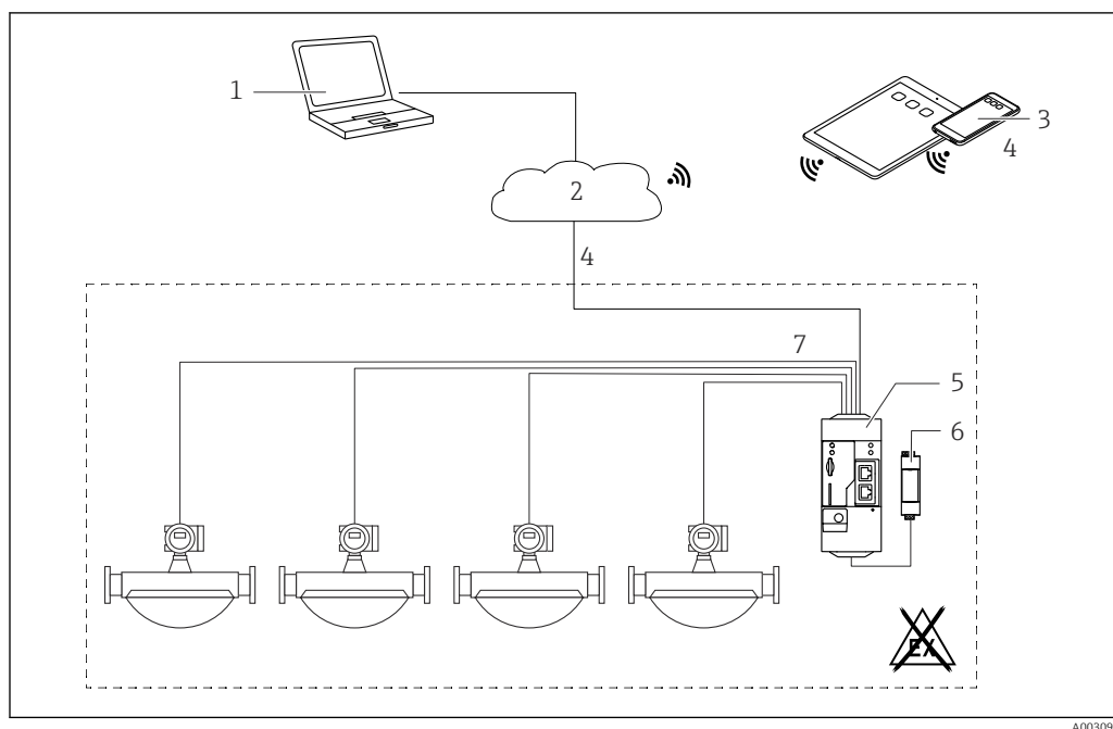
5 Arquitectura de sistema de un FXA42 Fieldgate con un contador de pulsos
