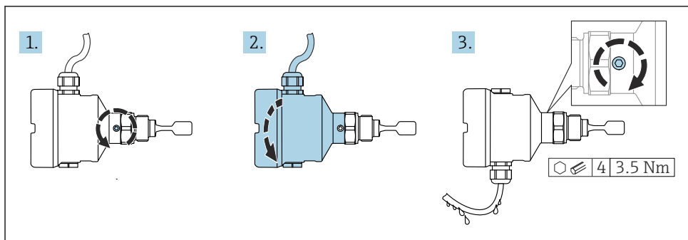
17 Gehäuse mit außenliegender Feststellschraube und Abtropfschlaufe
