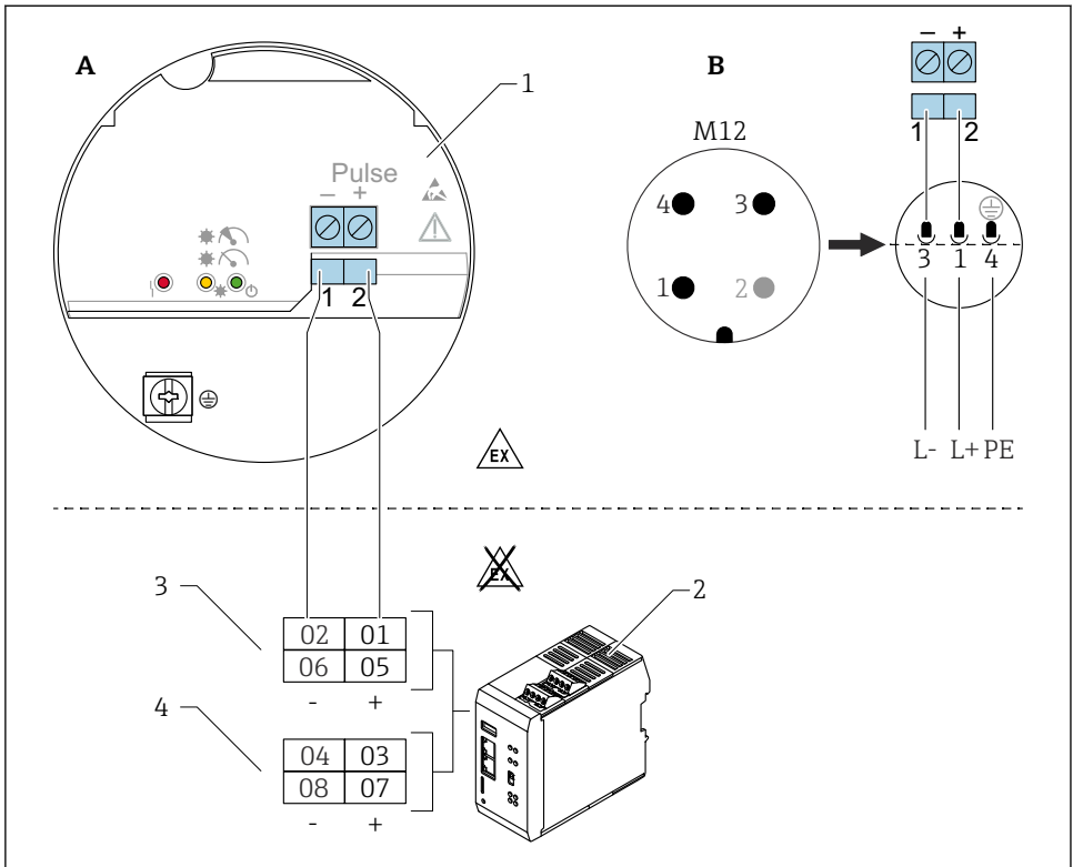
19 Anschlusschema: Anschluss Elektronikeinsatz FEL60D an den Dichterechner QML51
