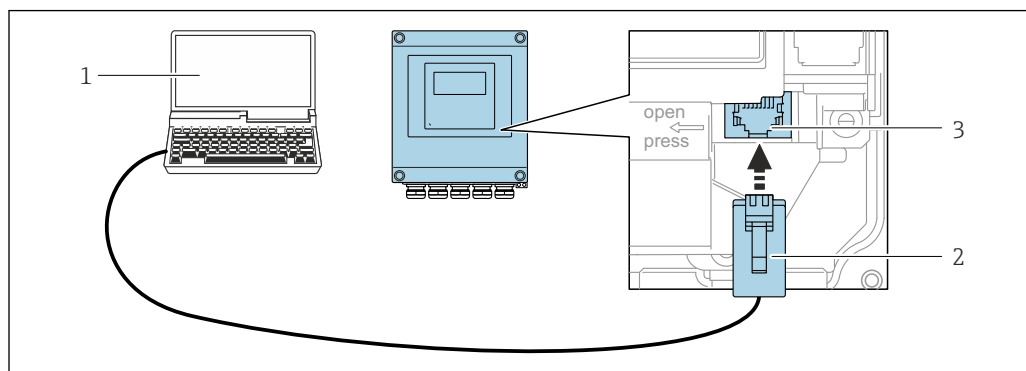
62 Conexión mediante la interfaz de servicio (CDI-RJ45)
