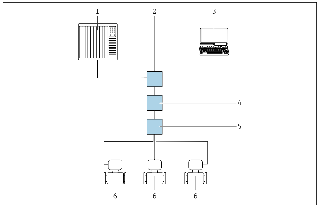
60 Opciones de configuración a distancia mediante el protocolo Modbus TCP a través de Ethernet-APL (activo)
