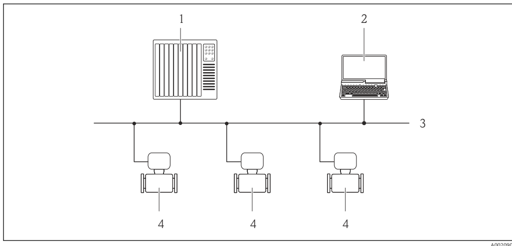
23 Варианты дистанционного управления через сеть PROFIBUS DP
