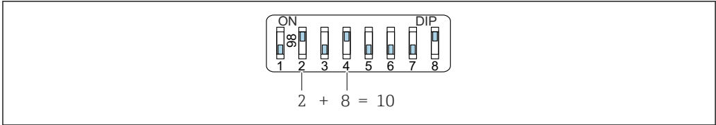
11 Ejemplo de direccionamiento por hardware; el interruptor 8 está en la posición "ON"; los interruptores 1 a 7 definen la dirección.
