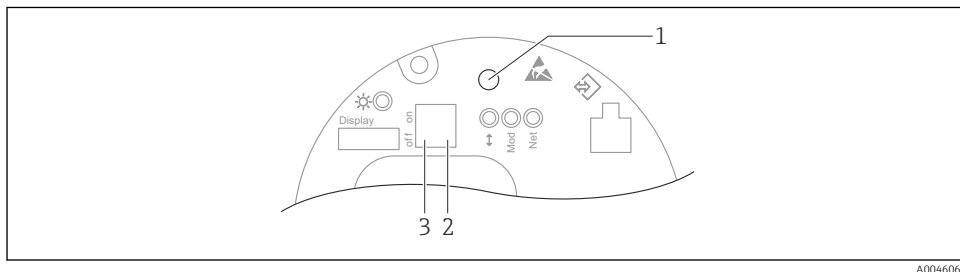
6 Tastele de acționare și comutatoarele tip DIP switch de pe inserția electronică Ethernet-APL
