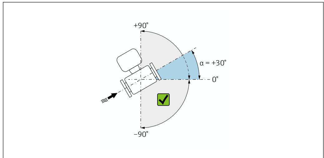
15 Visão lateral com direção da vazão da esquerda para a direita.
