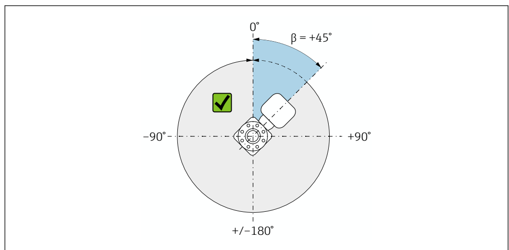
16 Visão de cima na direção da vazão
