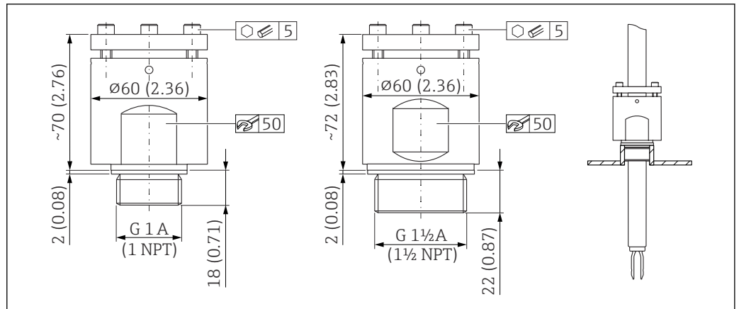
图 34 高压滑动套管。测量单位 mm (in)
