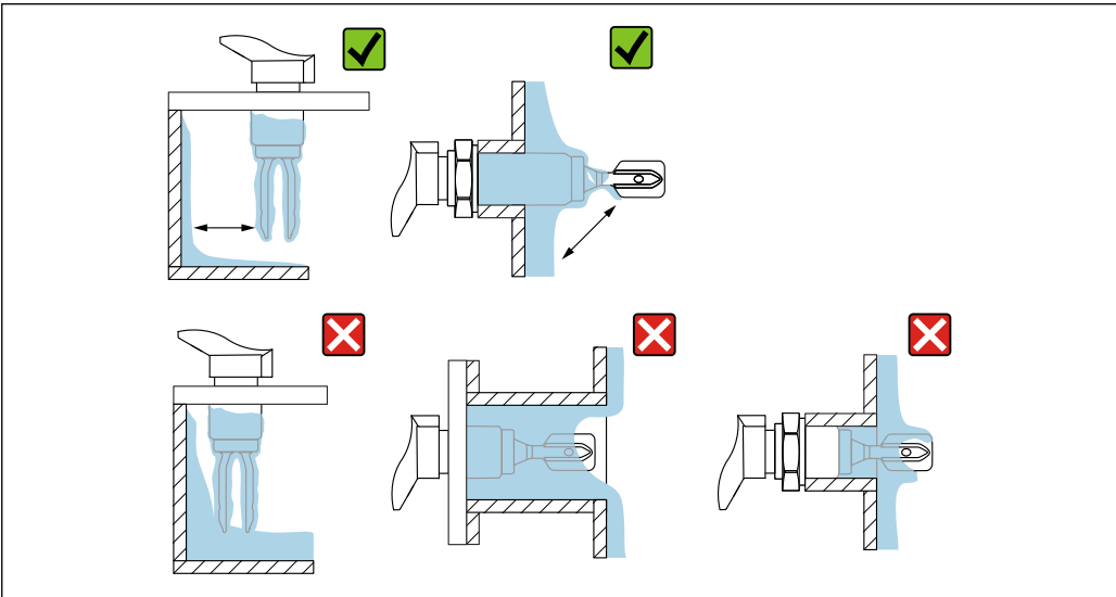
7 安装实例：测量高粘度过程介质
