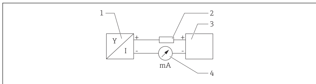
图 17 HART 信号回路连接框图
