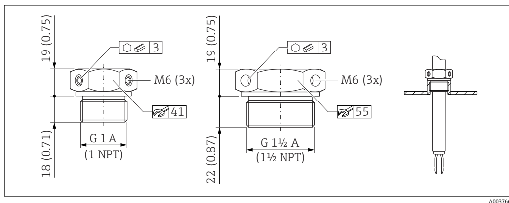
图 33 常压滑动套管 p_e = 0 \text{ bar} (0 psi)。测量单位 mm (in)
