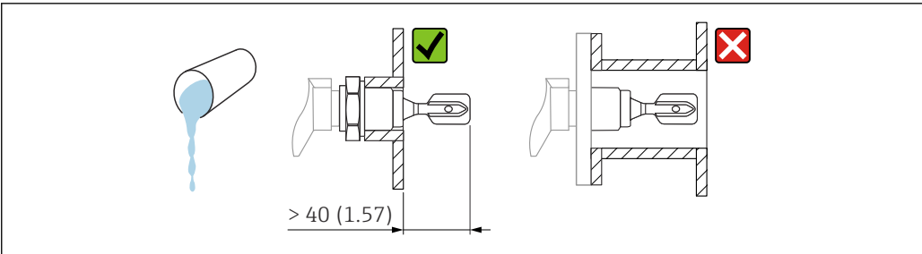
6 安装实例：测量高粘度液体。测量单位 mm (in)
