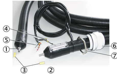
Abbildung 4: Beheizte Messgasleitung
