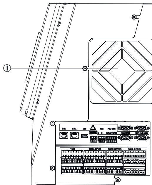
Abbildung 13: Elektronikgehäuse (rechte Seite)
