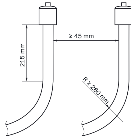
Abbildung 5: Leitungen – Abstand und Biegeradius
