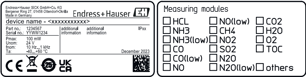
Abbildung 1: Typenschild Gesamtgerät, schematische Darstellung
