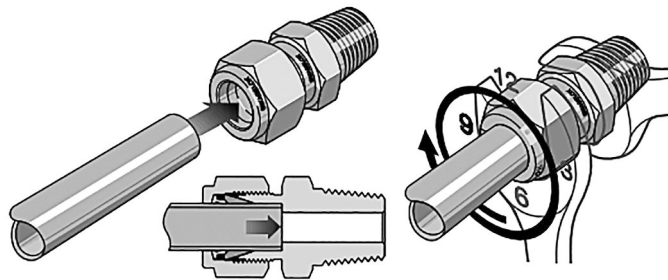
Abbildung 6: Edelstahlverschraubung
