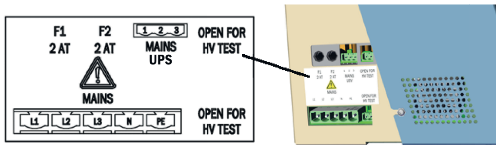
Abbildung 10: Anschluss Spannungsversorgung
