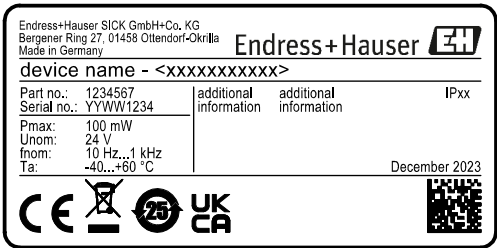
Abbildung 2: Typenschild Analysator, schematische Darstellung
