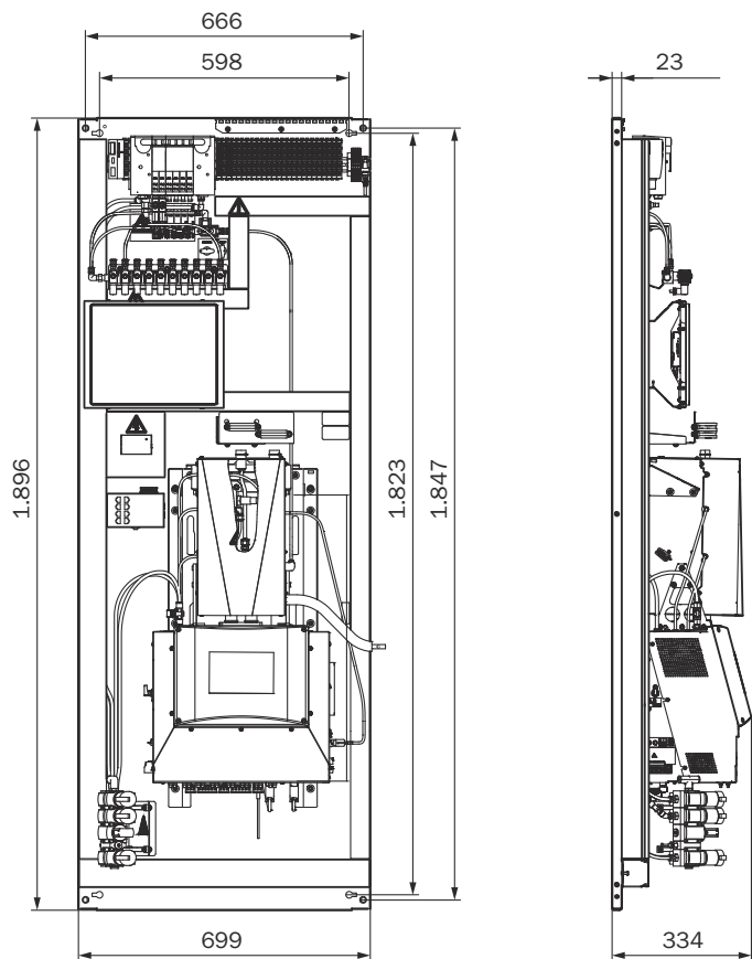
Abbildung 14: MCS200HW-MP (Maße in mm)
