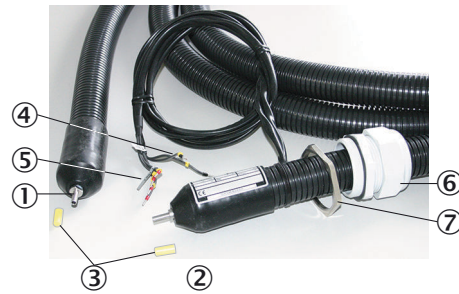
Abbildung 3: Beheizte Messgasleitung
