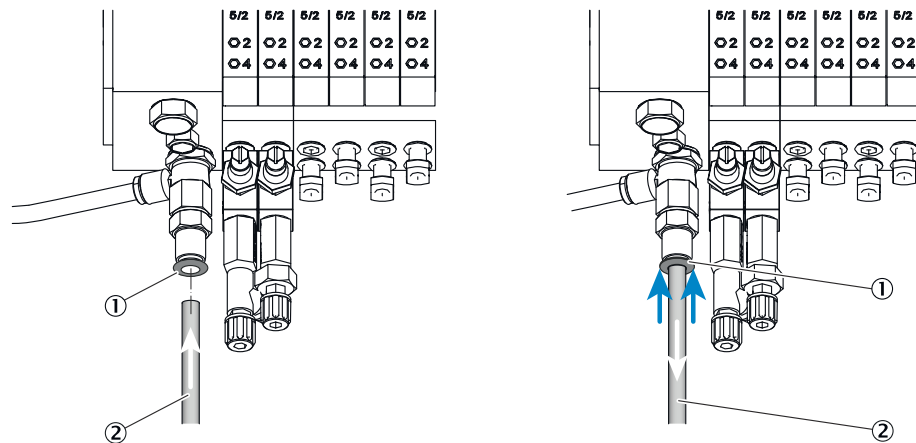
Abbildung 7: Steckverschraubung mit Sicherungsring (beispielhafte Abbildung)
