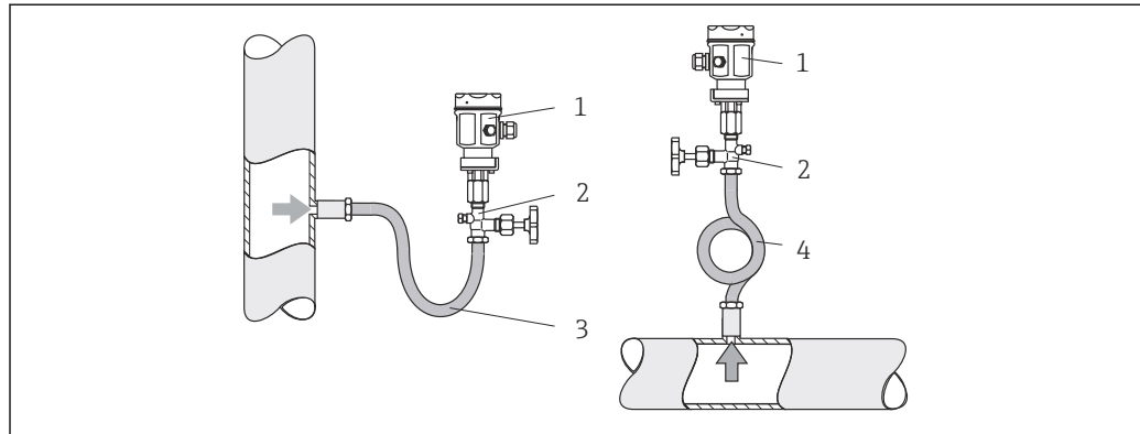
14 Montaje para medición de presión en vapores
