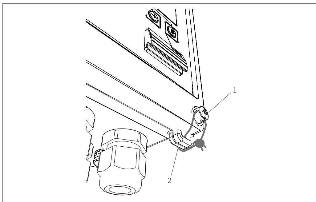
31 Precintado de plomo del equipo
