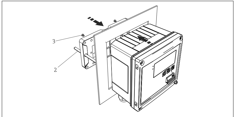
8 Montaje en panel
