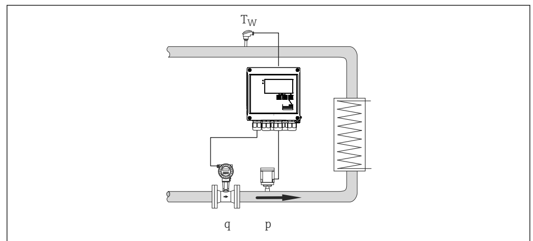
34 Diferencial de calor/p
