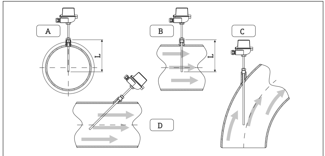
13 Tipos de instalación para sensores de temperatura
