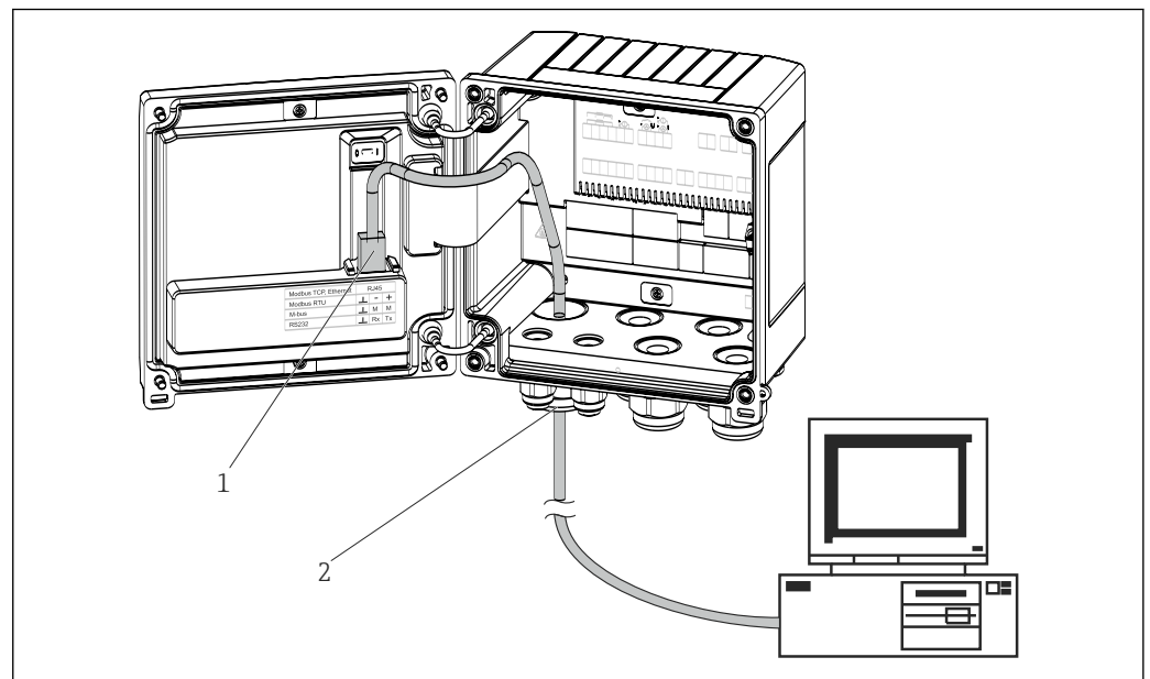
19 Conexión de Ethernet TCP/IP, Modbus TCP
