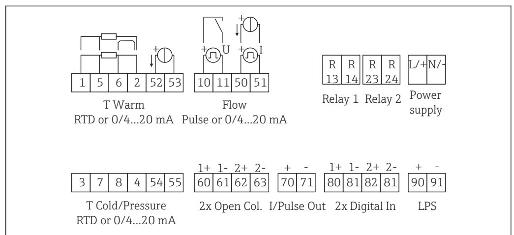
15 Diagrama de conexión del equipo
