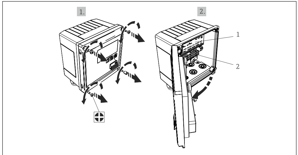
16 Abertura de la caja del equipo
