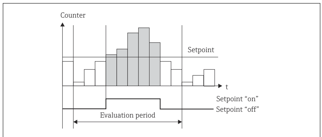
30 Valor de alarma para contadores
