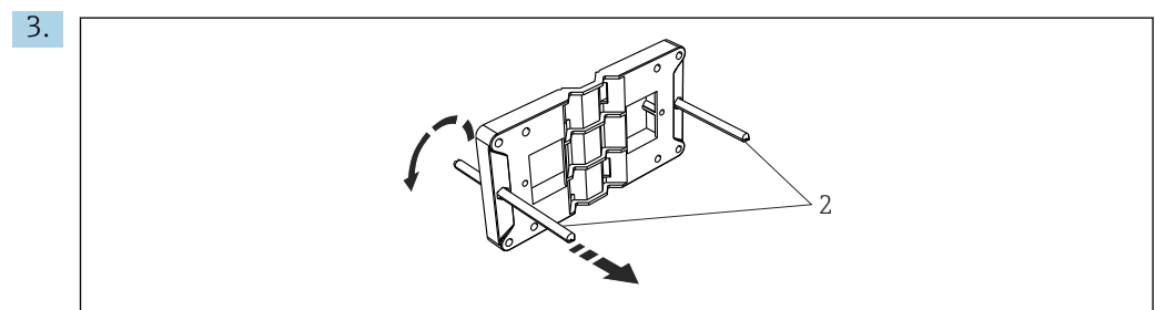
7 Preparación de la placa de montaje para montaje en armario
