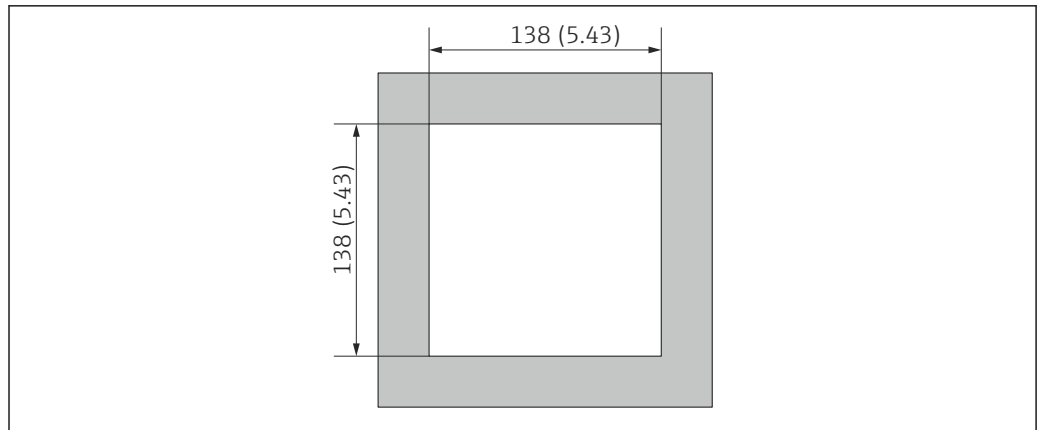
40 Apertura en el cuadro en mm (pulgadas)
