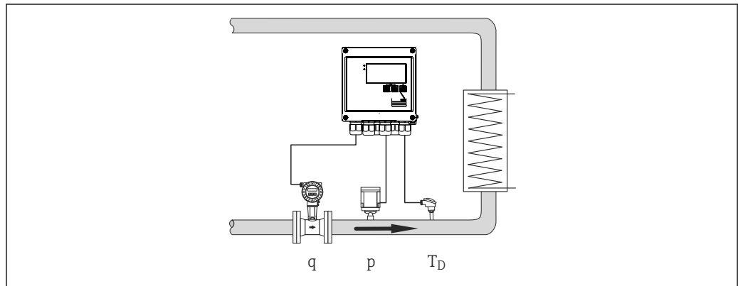
36 Cantidad de calor o diferencial de calor/p+T
