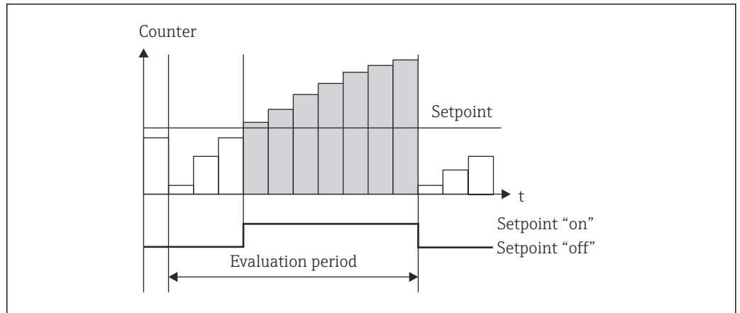
29 Valor de alarma para contadores
