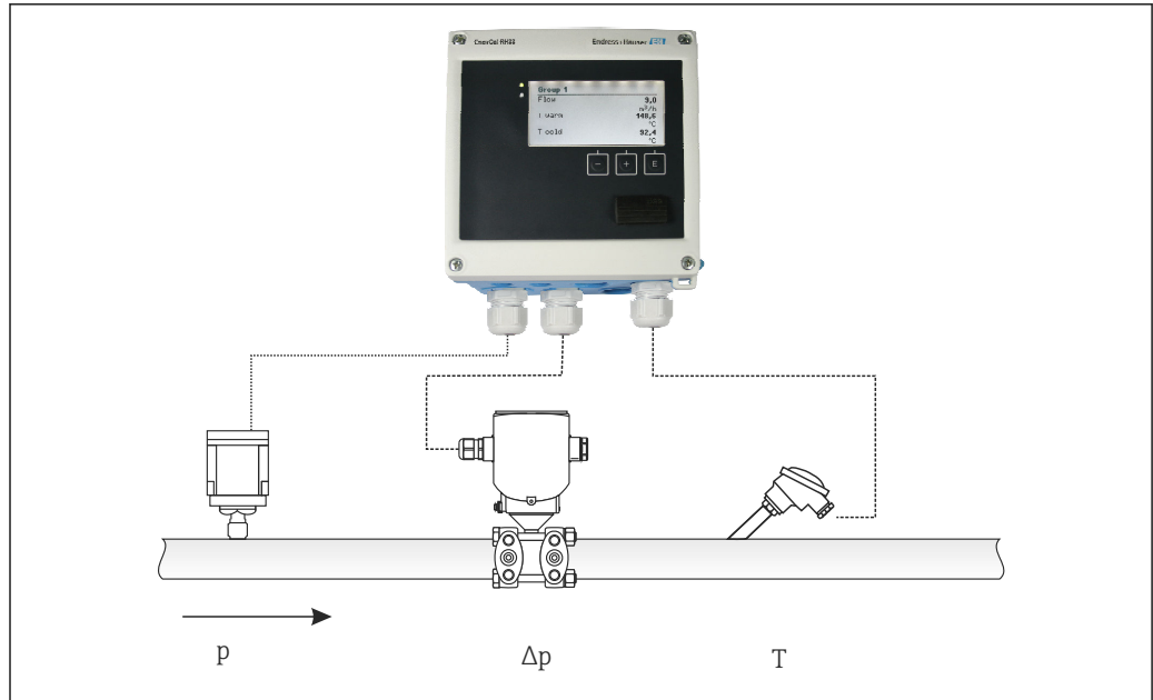
33 Determinación del caudal por presión diferencial
