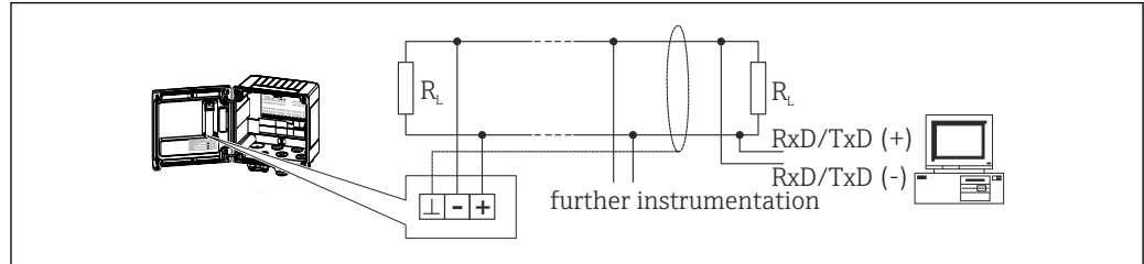
20 Conexión de Modbus RTU
