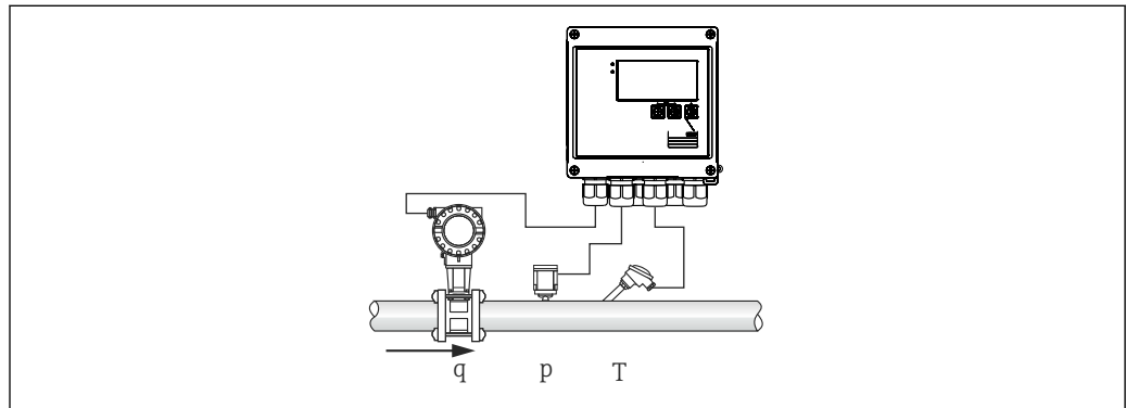
26 Uso de la tarificación para masa de vapor y flujo energético (opción)
