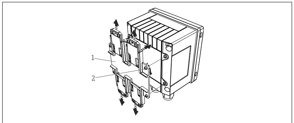
9 Preparación para el montaje en raíl DIN
