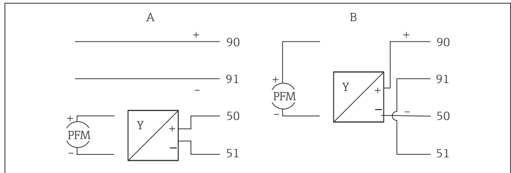
18 Conexión de los sensores de caudal activos
