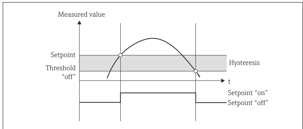
28 Modo de funcionamiento "SP upper"
