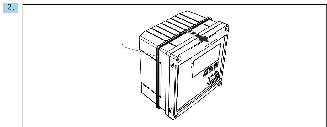
6 Montaje en panel
