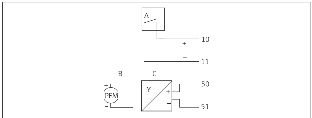
17 Conexión a un sensor de caudal
