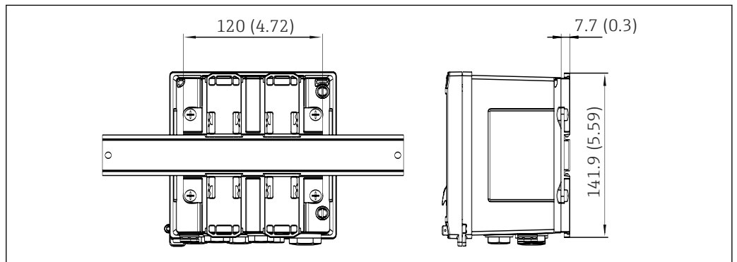
4 Dimensiones del adaptador para rail DIN en mm (in)
