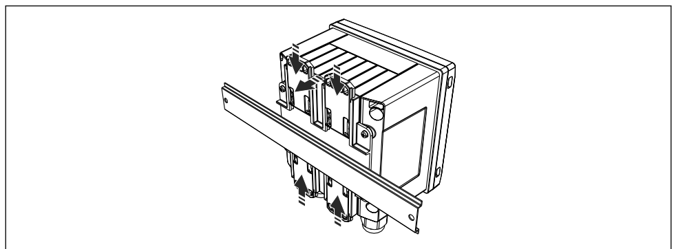
10 Montaje en raíl DIN
