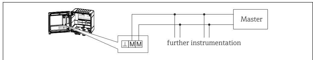
21 Conexión de M-Bus
