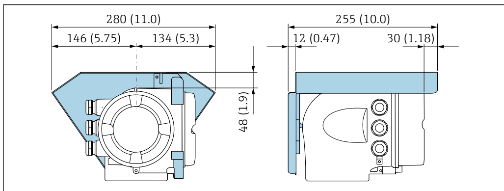
10 Copertura protettiva per Proline 500; unità mm (in)
