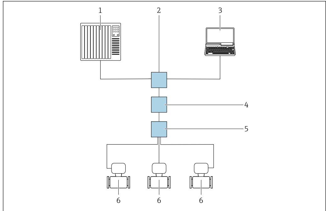
▣ 28 Opzioni per il funzionamento a distanza tramite il protocollo Modbus TCP su Ethernet-APL (attivo)
