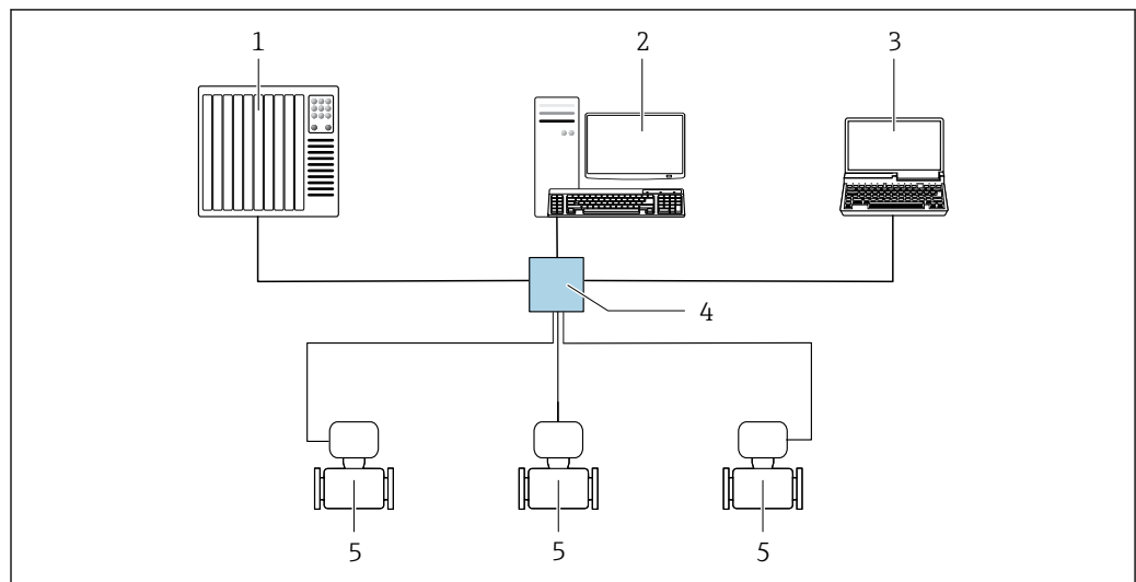
▣ 29 Opzioni per il funzionamento a distanza tramite Modbus TCP su Ethernet - 100 Mbit/s: topologia a stella
