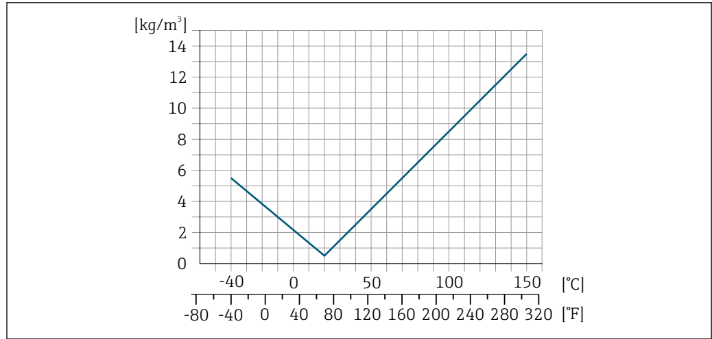
33 Ajustage sur site de la masse volumique, par exemple à +20 °C (+68 °F)
