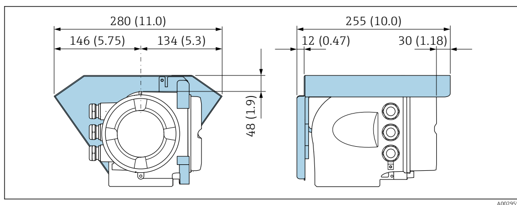
35 Tapa de protección ambiental para Proline 500; unidad mm (in)
