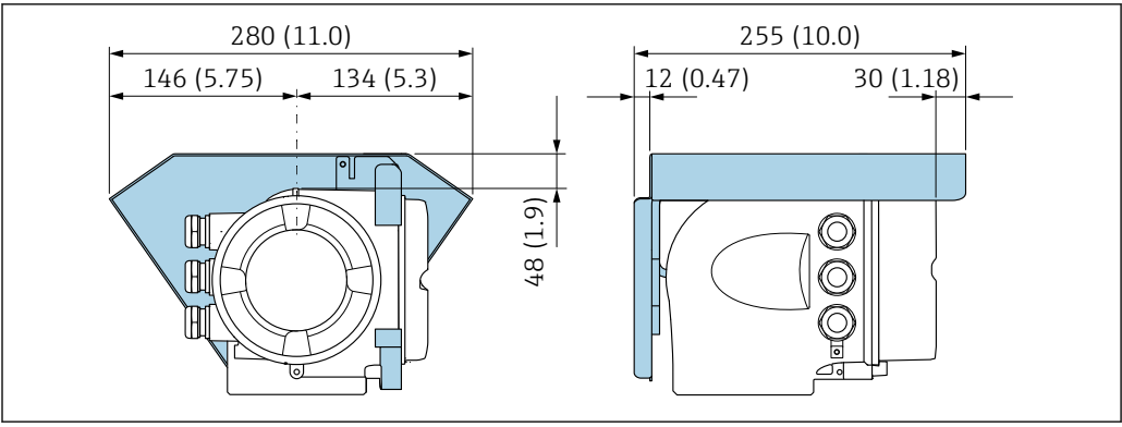
21 Tapa de protección ambiental para Proline 500; unidad mm (in)
