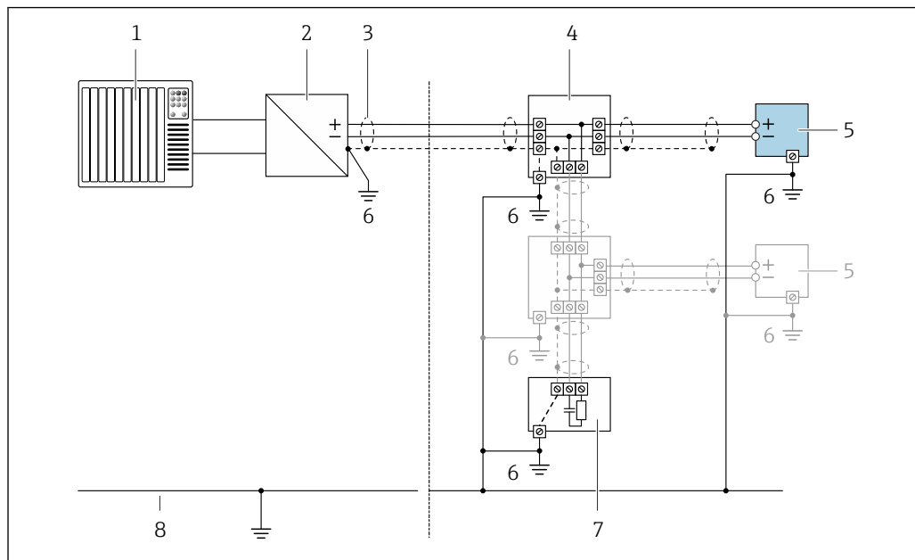
28 Пример подключения для интерфейса FOUNDATION Fieldbus
