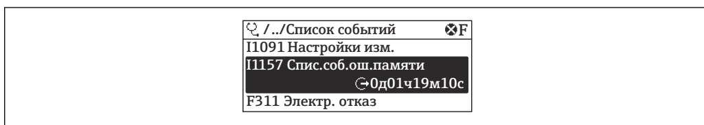
44 Использование на примере локального дисплея
