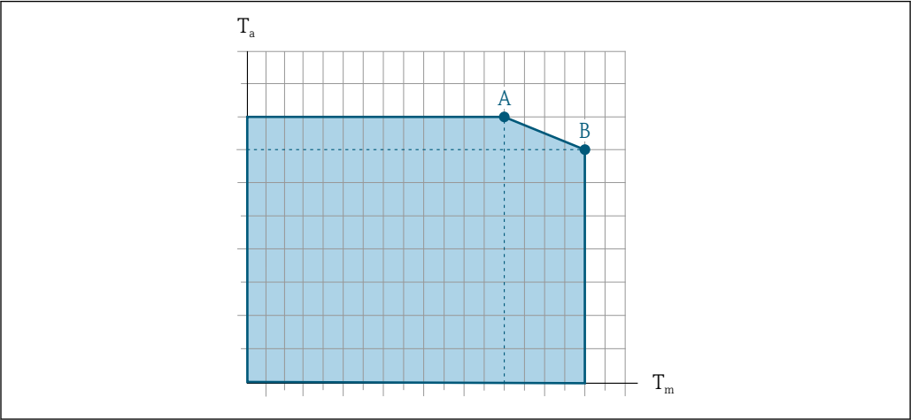
45 Пример зависимости, значения приведены в таблице. T a Температура окружающей среды T m Температура технологической среды A Максимально допустимая температура среды T m при T a max = 60 °C (140 °F); более высокие значения температуры технологической среды T m требуют снижения температуры окружающей среды T a B Максимально допустимая температура окружающей среды T a при максимальной установленной температуре среды T m для сенсора
