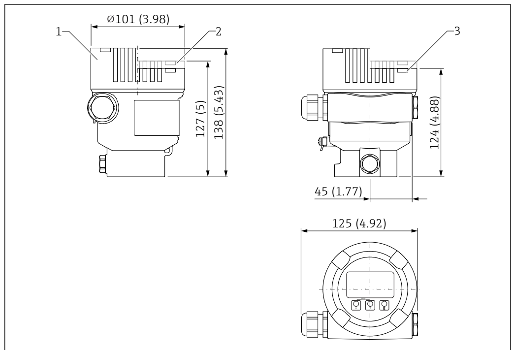
24 Dimensioni della custodia a vano unico, in alluminio, rivestita. Unità di misura mm (in)
