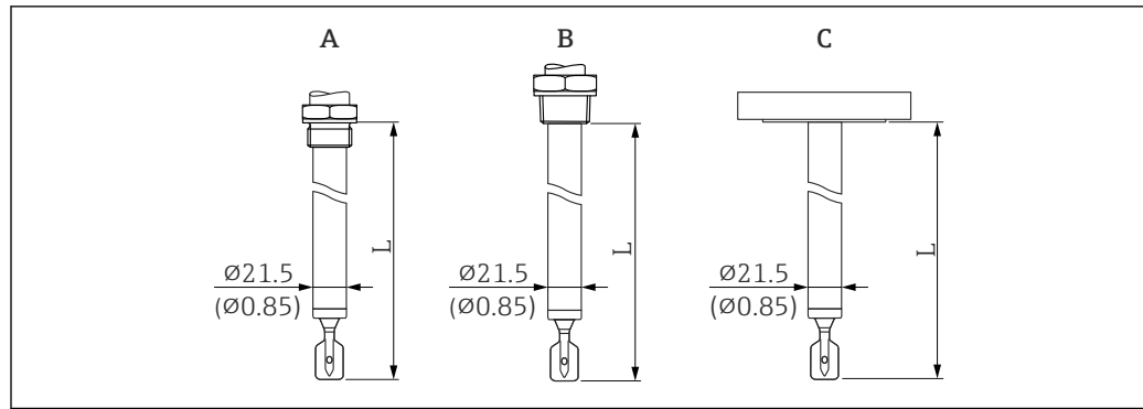
30 Design della sonda: tubo di estensione, versione con tubo corto (lunghezza dei sensori L). Unità di misura mm (in)
