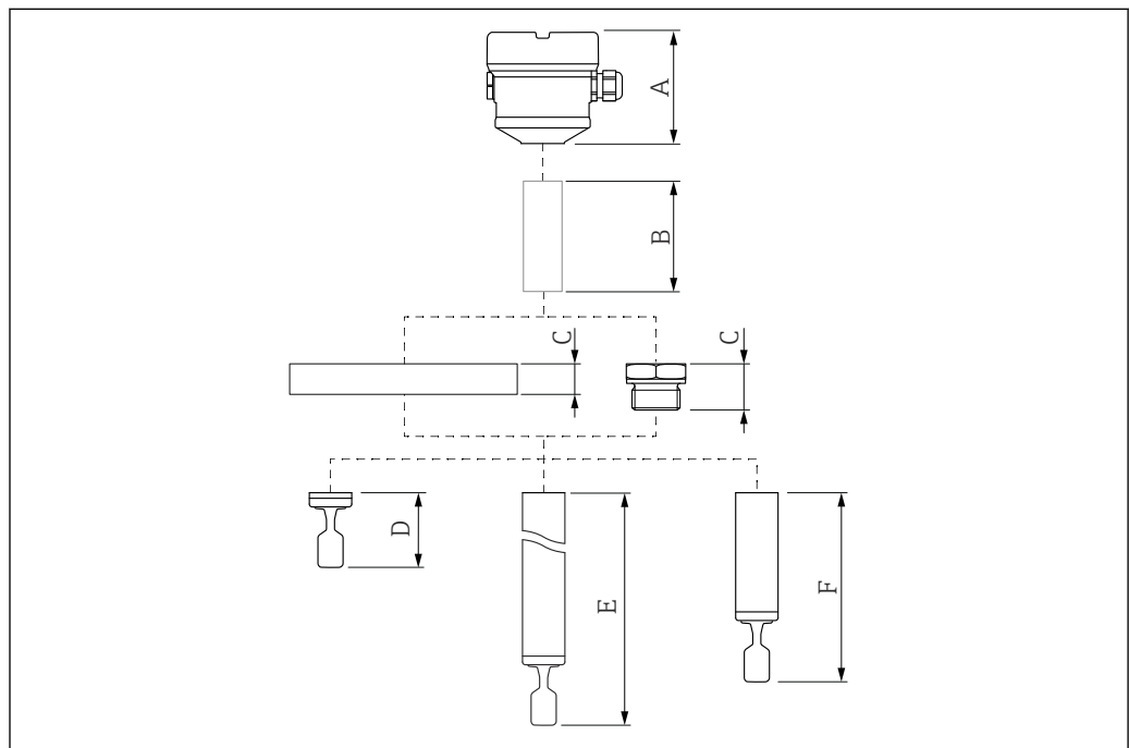
22 Componenti per determinare l'altezza del dispositivo
