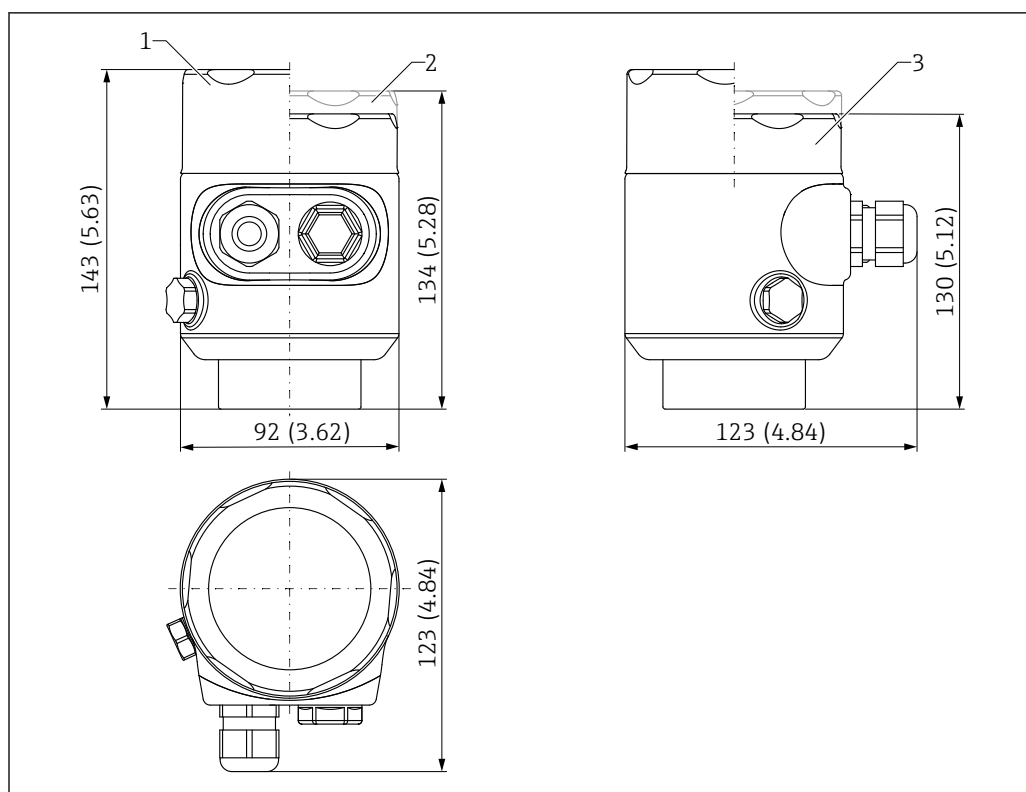
■ 25 Dimensioni della custodia a vano unico, in 316L, igienica. Unità di misura mm (in)
