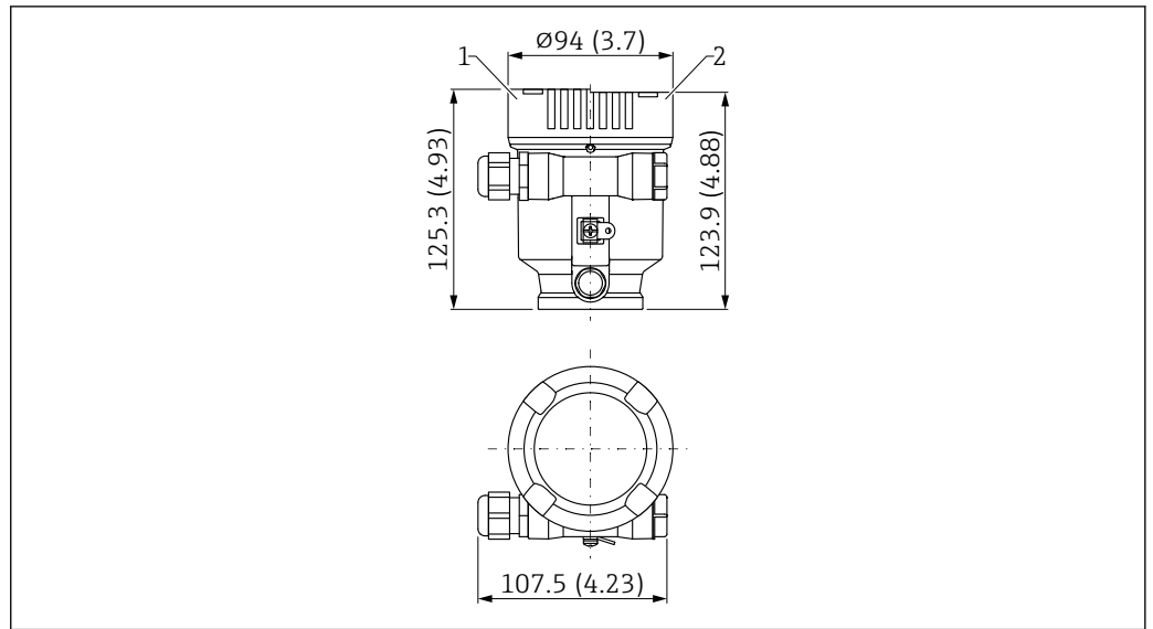
23 Dimensioni; custodia a vano unico, in plastica; completa di raccordo M20 e tappo in plastica. Unità di misura mm (in)
