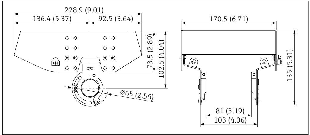
46 Tettuccio di protezione dalle intemperie per custodia a doppio scomparto. Unità di misura mm (in)
