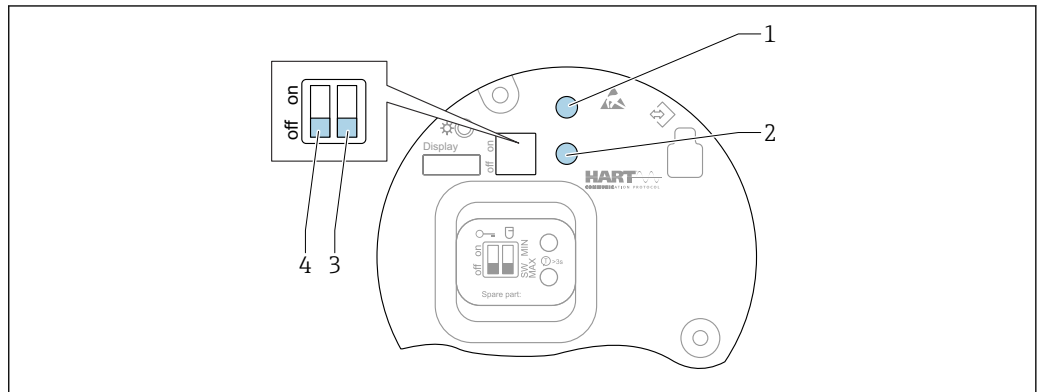
■ 44 Tasti operativi e microinterruttori sull'inserto elettronico FEL60H
