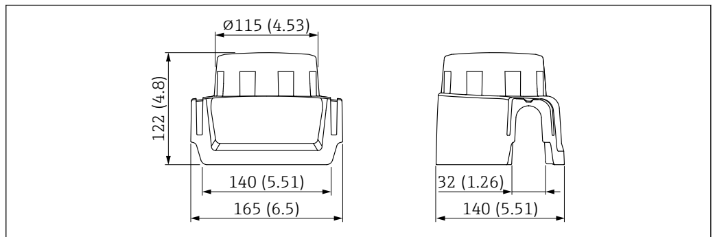
47 Coperchio di protezione per custodia a vano unico in alluminio. Unità di misura mm (in)
