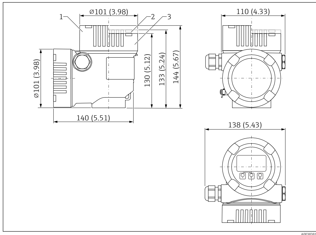
27 Dimensioni; custodia a vano doppio, a L, 316 L; completa di raccordo M20 e tappo in plastica. Unità di misura mm (in)
