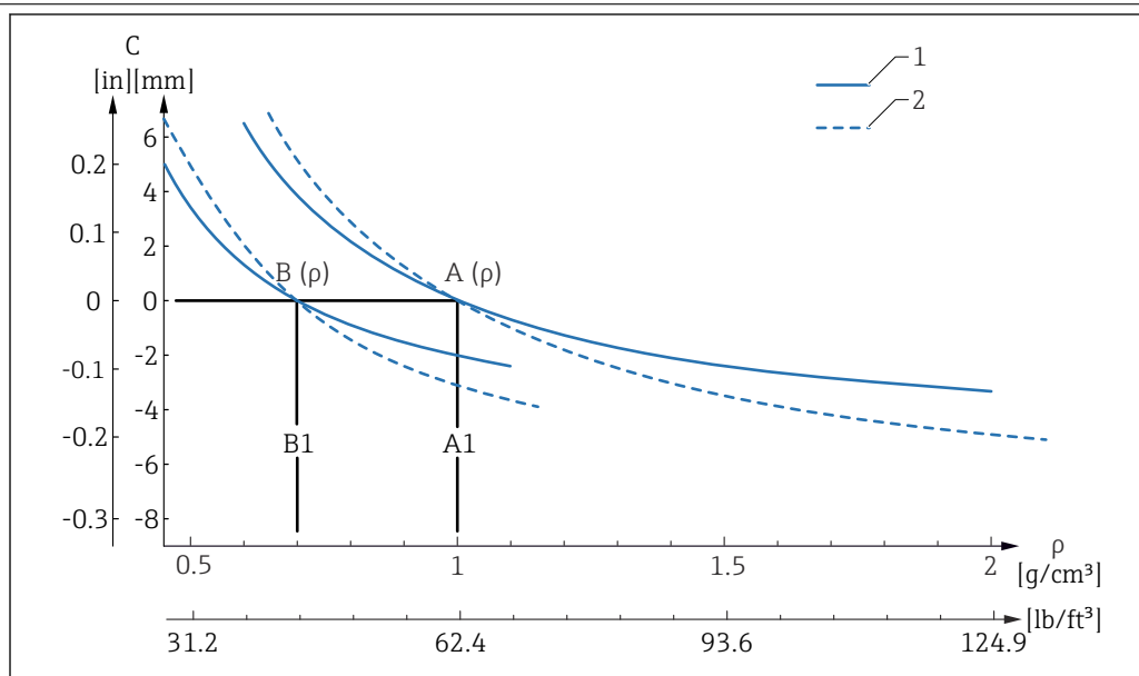
6 Deviazione del punto di commutazione in base alla densità
