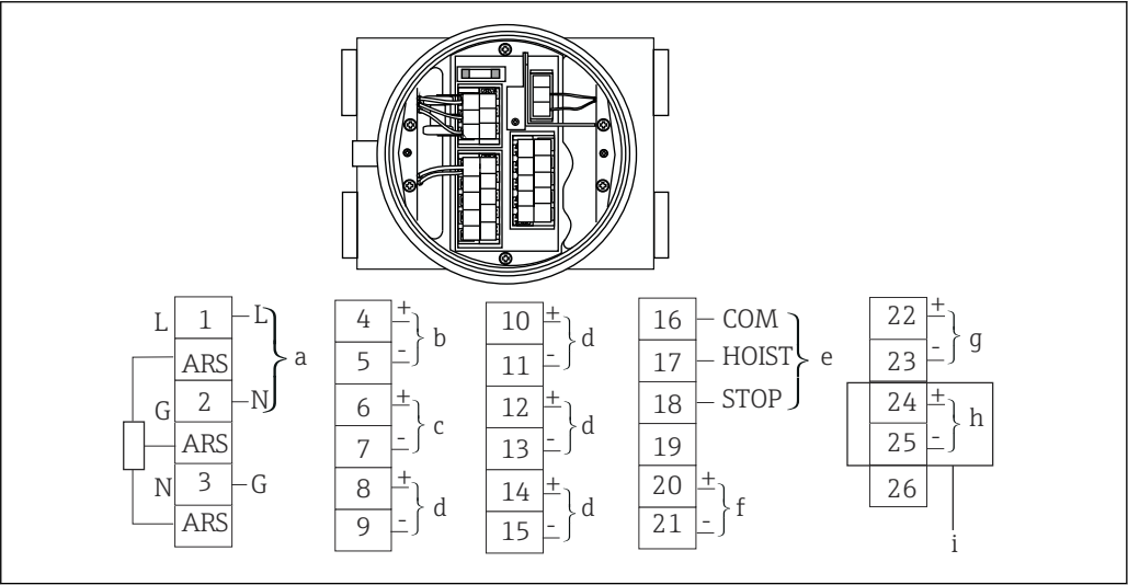
8 NMS5 的接线端子
