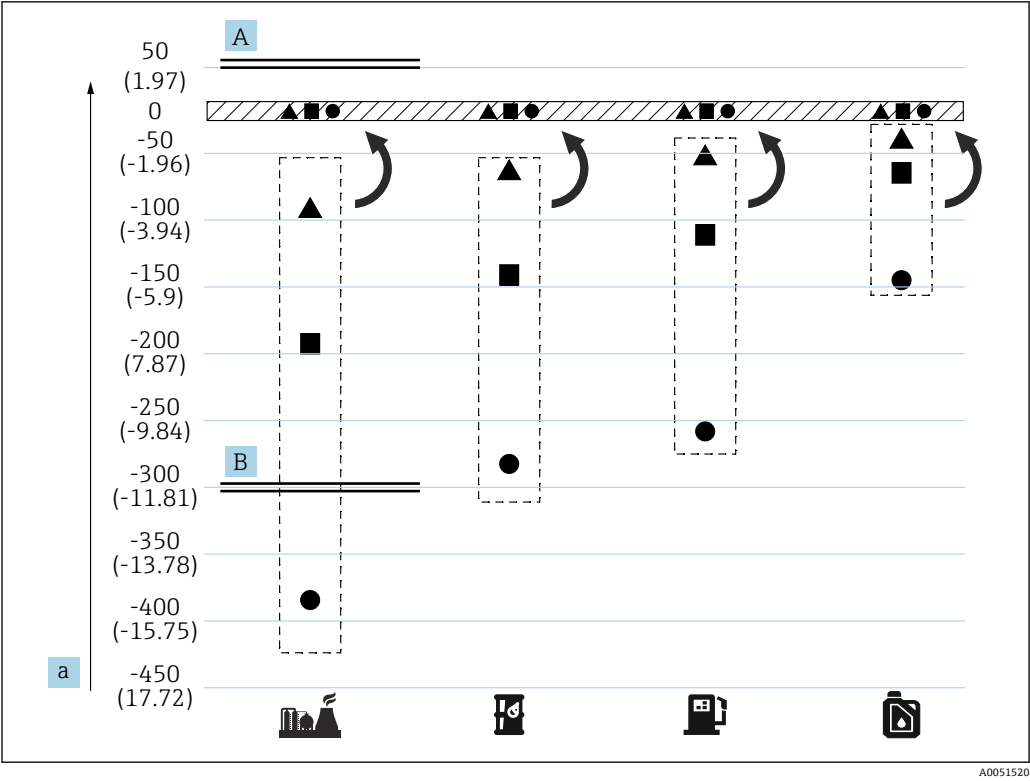
35 针对三层介质工况的补偿功能
