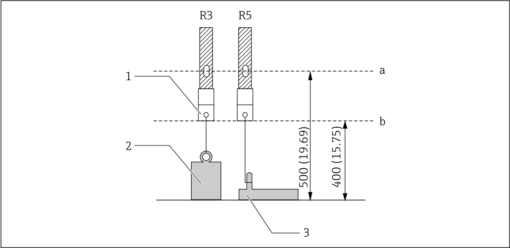
16 安装附件 1 (“转换器+平均温度探头”型仪表)。测量单位 mm (in)
