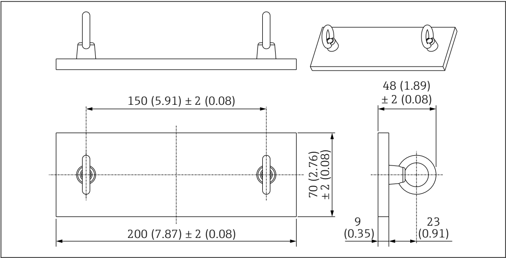
42 绞线连接孔。测量单位 mm (in)
