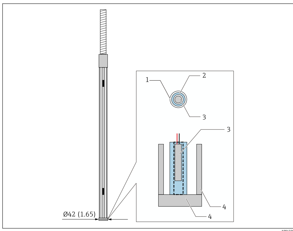
图 33 油水界面测量探头结构。测量单位 mm (in)
