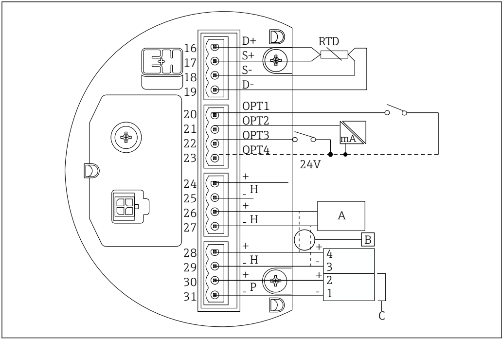
图 9 NRF590 的本安接线端子 A HART 型传感器（作为独立 HART 现场总线回路在内部相互连接） B 现场总线回路 C 仅适用 Micropilot S 系列
