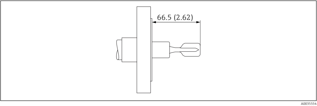
43 Exemplo com flange. Unidade de medida mm (in)
