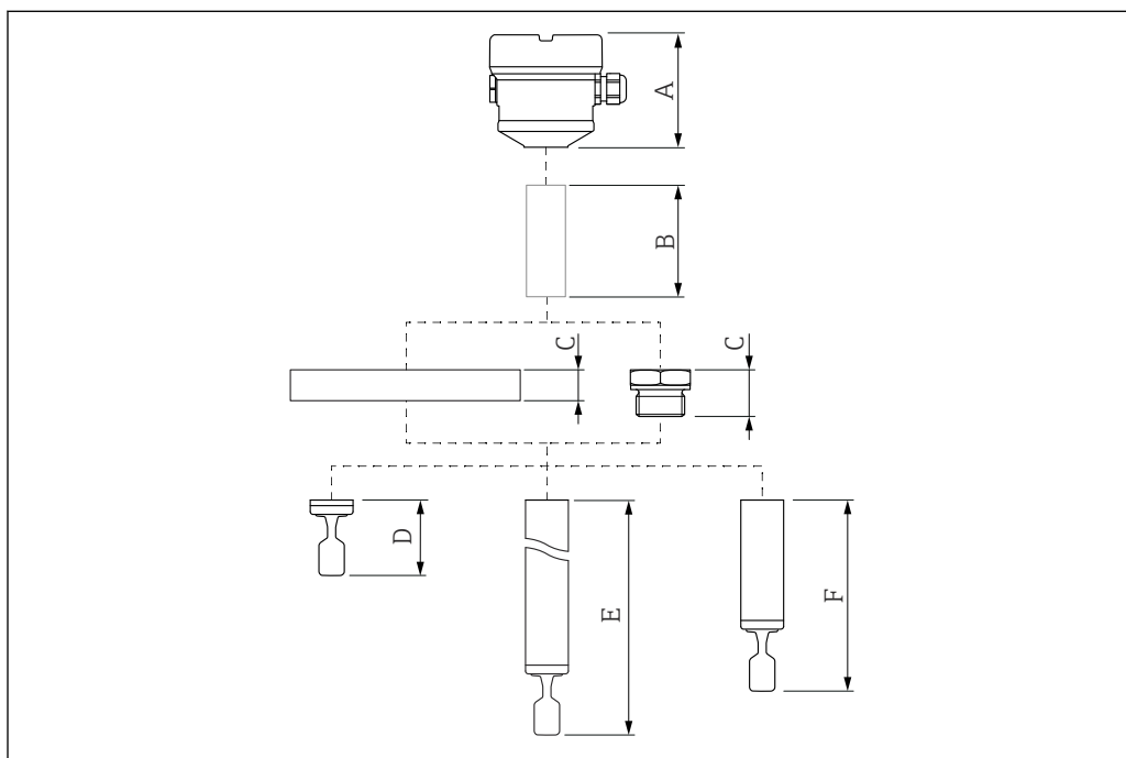
Fig. 22 Componentes para determinar a altura do equipamento
