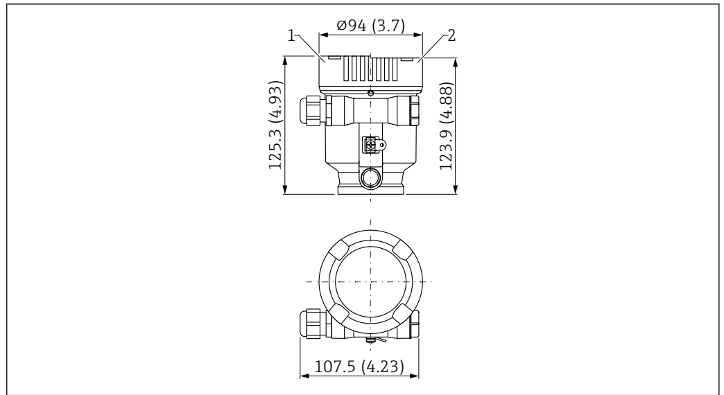
23 Dimensões; invólucro de compartimento único, plástico; incl. acoplamento e conector M20, plástico. Unidade de medida mm (in)
