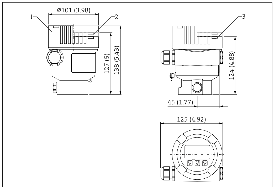
24 Dimensões de compartimento único, alumínio, revestido. Unidade de medida mm (in)
