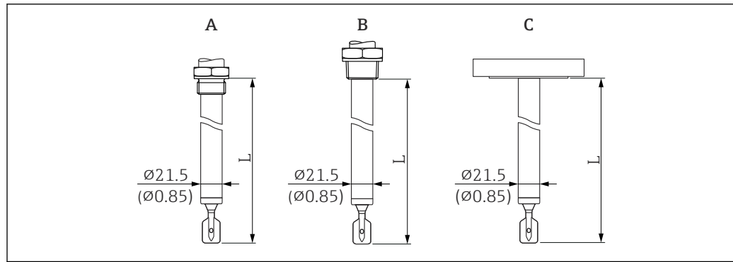
30 Projetos das sondas: tubo de extensão, versão de tubo curto (comprimento do sensor L). Unidade de medida mm (in)
