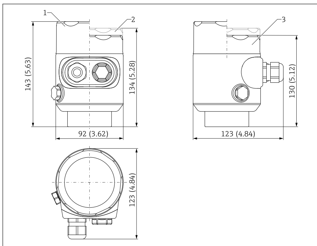
25 Dimensões do invólucro de compartimento único, 316L, higiênico. Unidade de medida mm (in)
