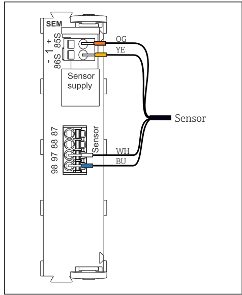
31 SEM 모듈에 분광기 연결
