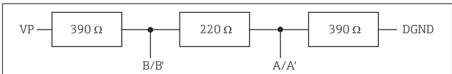
60 내부 중단의 구조
