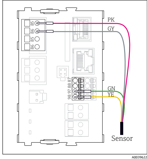
29 추가 공급 전압이 있는 Memosens 센서
