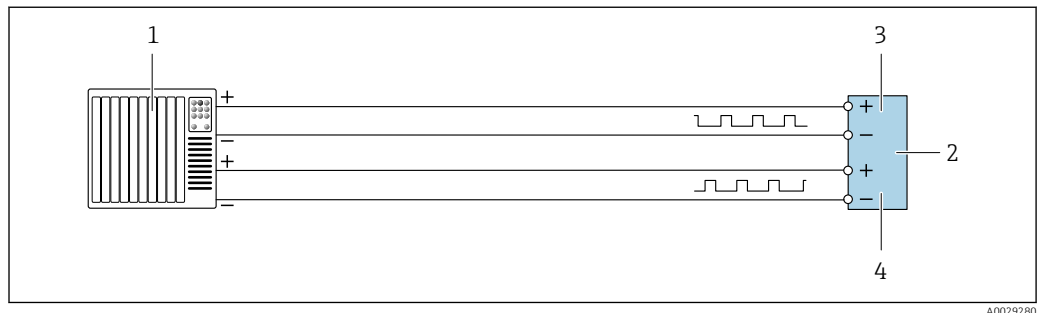
10 Пример подключения двойного импульсного выхода (активного)
