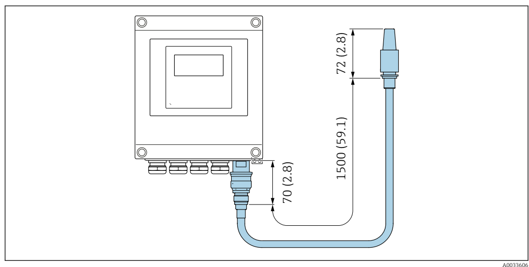
27 Единицы измерения – мм (дюймы)
