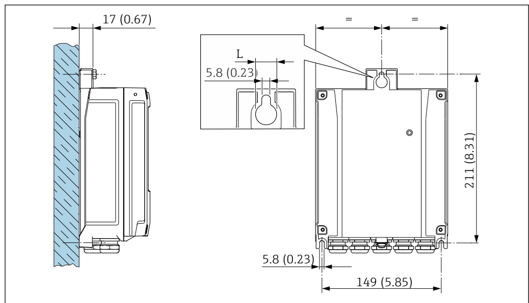
20 Единицы измерения – мм (дюймы)
