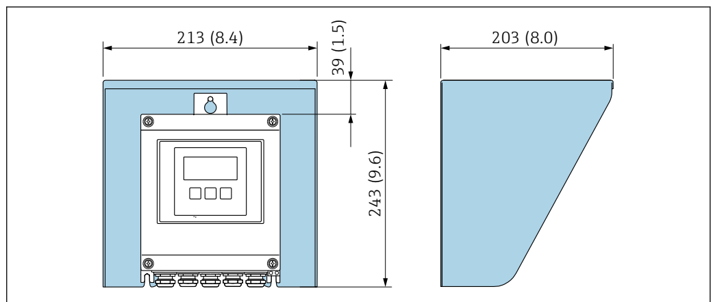
25 Защитный козырек от погодных явлений для Proline 500 – цифровое исполнение; мм (дюймы)
