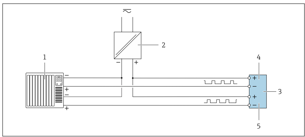
11 Пример подключения двойного импульсного выхода (пассивного)
