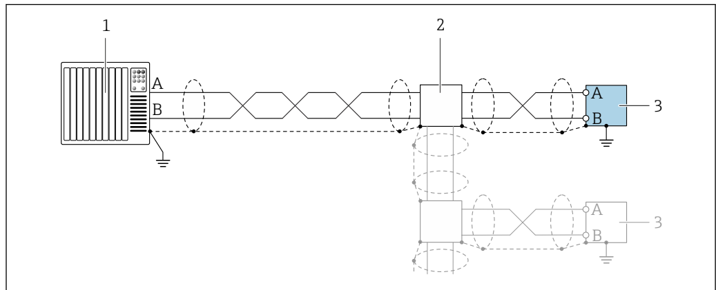
24 Anschlussbeispiel für Modbus RS485
