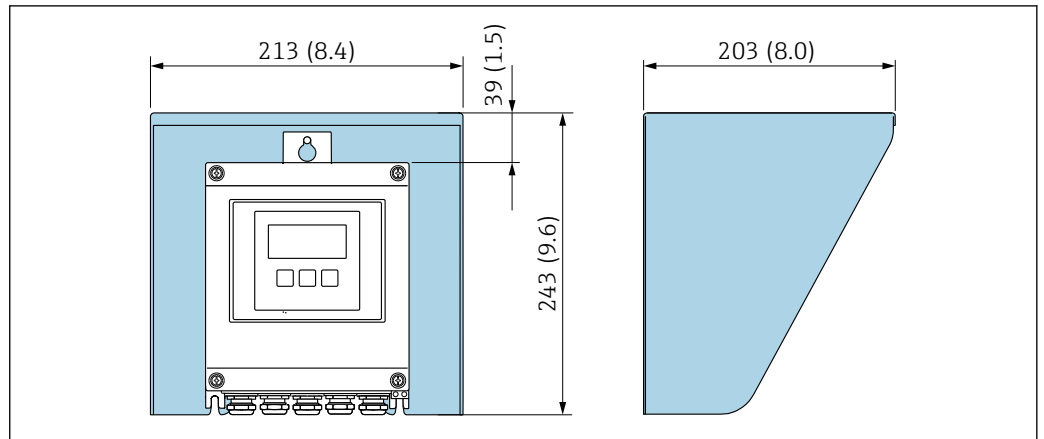
32 Tapa de protección ambiental para Proline 500, digital; unidad mm (in)
