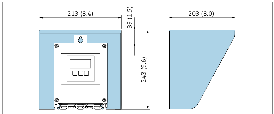
39 Tapa de protección ambiental para Proline 500, digital; unidad mm (in)
