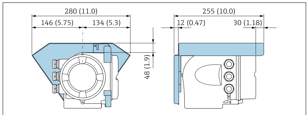
33 Tapa de protección ambiental para Proline 500; unidad mm (in)
