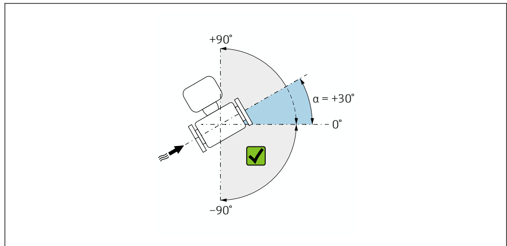
19 Vista lateral con sentido de flujo de izquierda a derecha.
