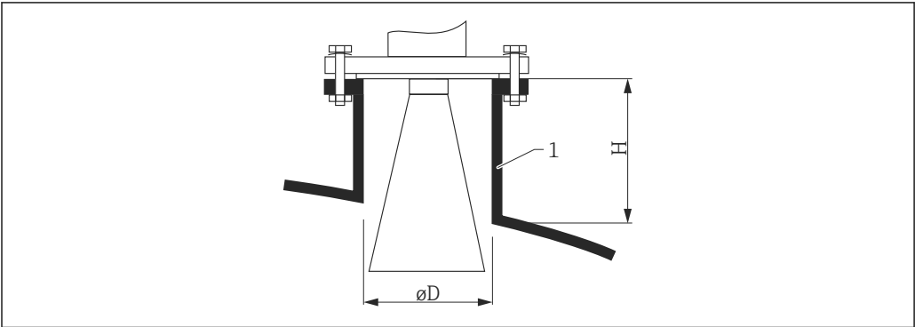
図 20 ホーンアンテナのノズル高と直径
