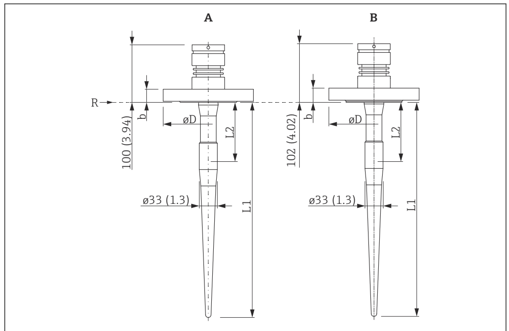
図 27 フランジ付き機器の寸法。測定単位 mm (in)
