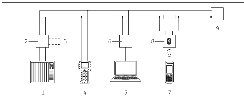
図 33 HART 経由のリモート操作用オプション
