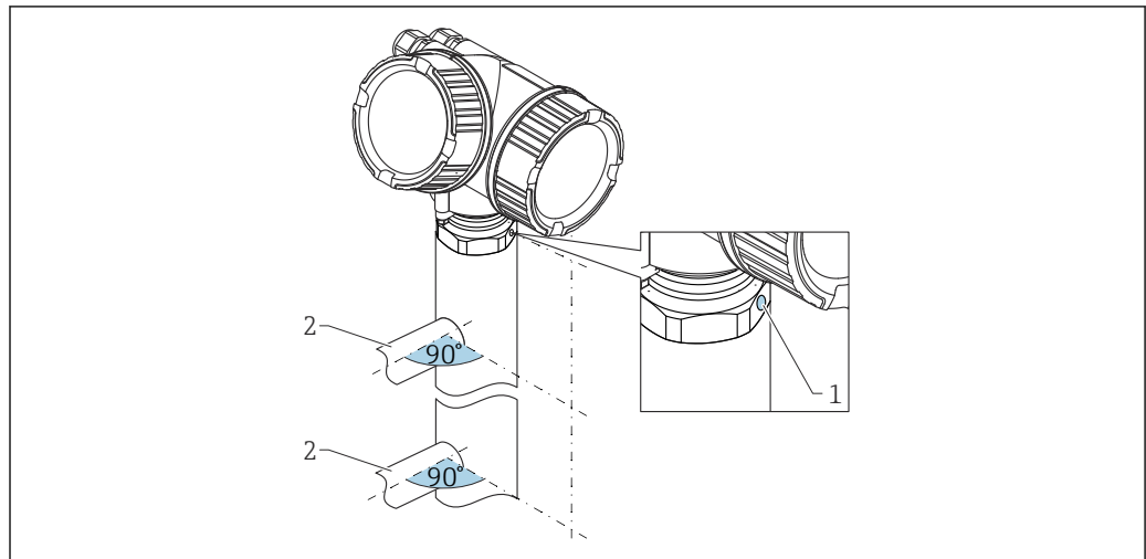
図 22 外筒管への設置
