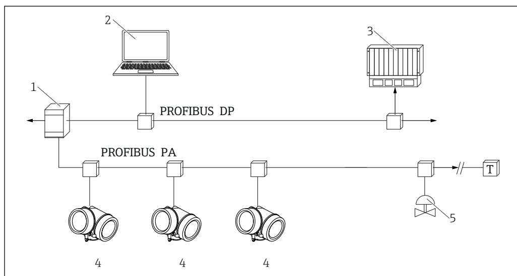
図 34 PROFIBUS PA プロトコルを介したリモート操作用のオプション
