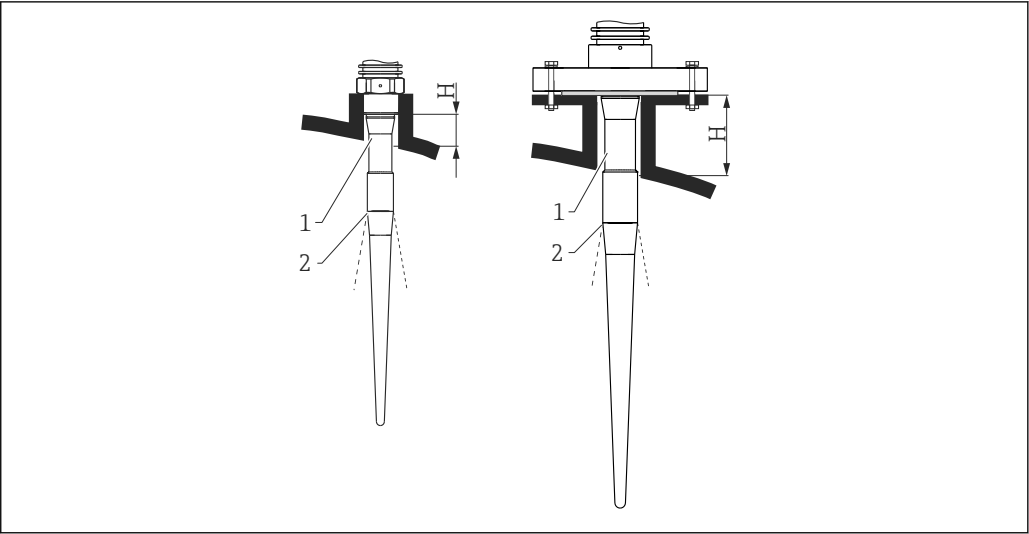
図 19 ロッドアンテナのノズル高 (FMR53)
