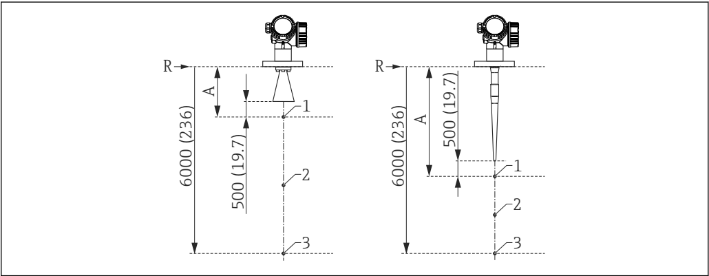
図 40 3 点リニアリティプロトコルの各点、使用単位：mm (in)
