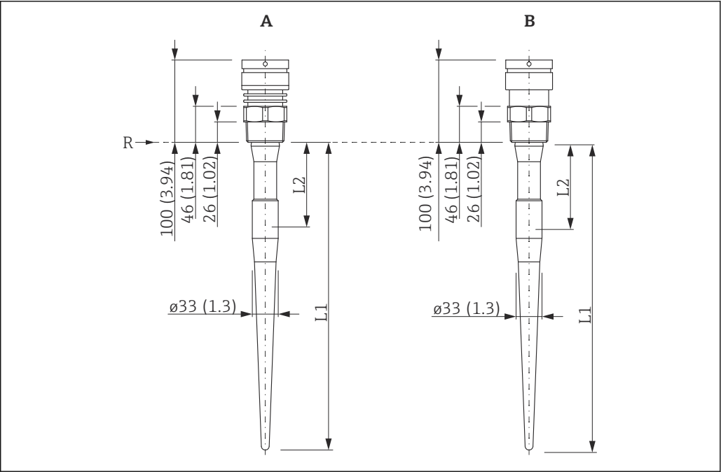
図 28 ネジ接続付き機器の寸法。測定単位 mm (in)
