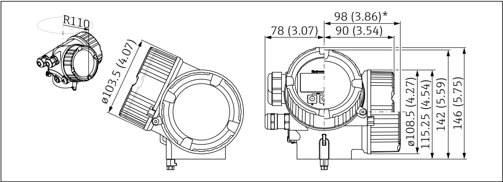
図 24 ハウジング GT18 (SUS 316L 相当)。測定単位 mm (in)
