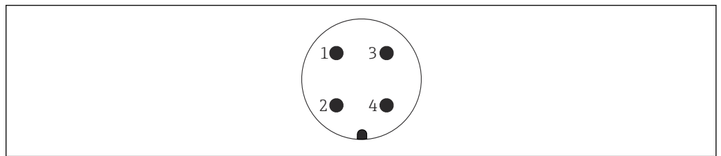
図 17 7/8" プラグのピン割当て
