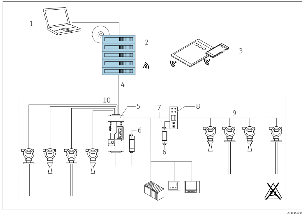
38 SupplyCare Enterprise SCE30B を使用した在槽管理プラットフォームの例
