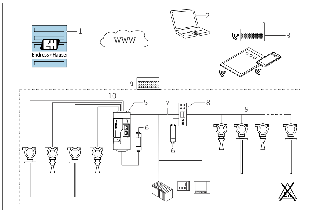
図 39 SupplyCare Hosting SCH30 を使用した在槽管理プラットフォームの例
