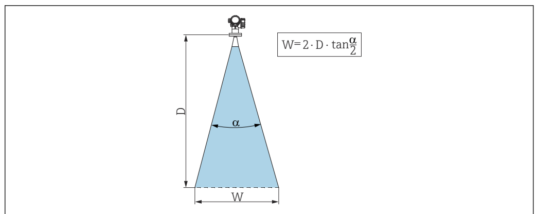
図 18 放射角 \alpha 、距離 D 、ビーム幅 W の関係
