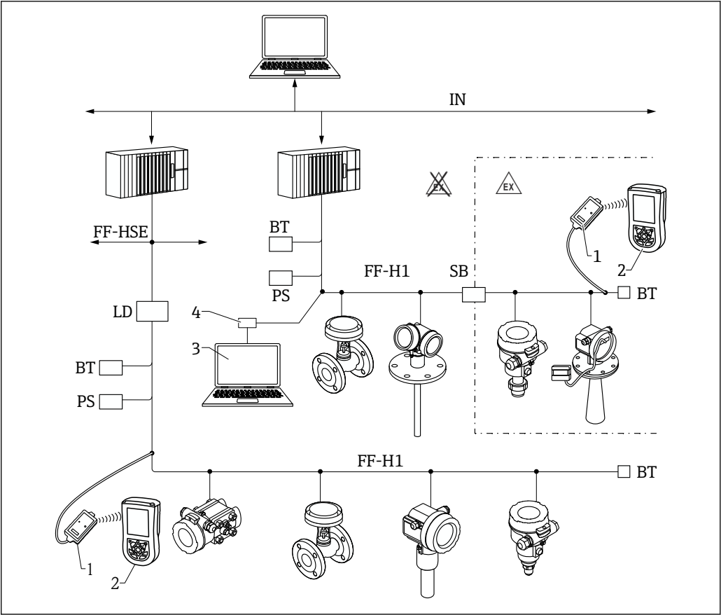
35 FOUNDATION フィールドバスシステム構成および関連するコンポーネント
