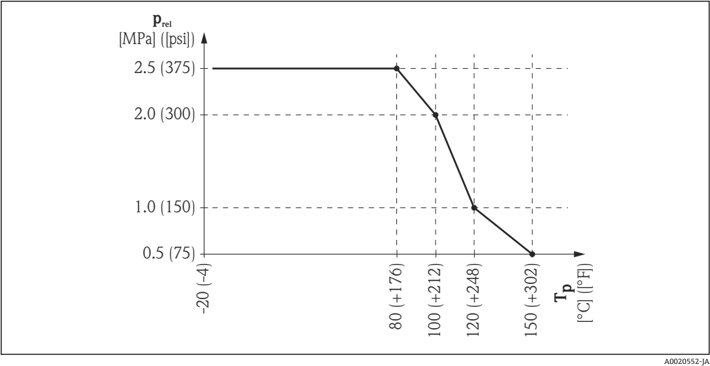
23 プレーナアンテナ付き FMR54 : プロセス温度およびプロセス圧力の許容範囲
