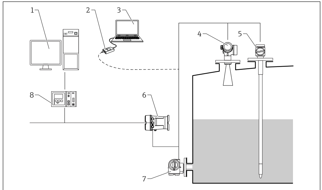
図 37 以下のコンポーネントで構成される計測システム
