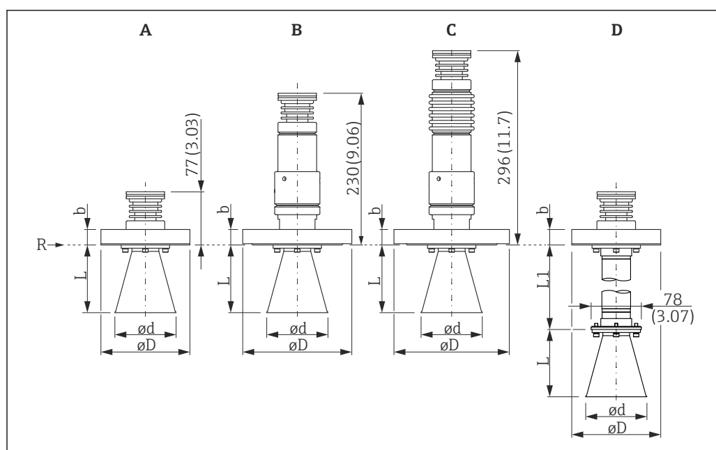
図 29 ホーンアンテナ付き FMR54 の寸法。測定単位 mm (in)
