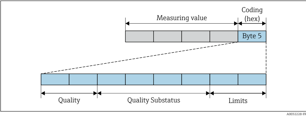
33 Structure de l'octet de codage
