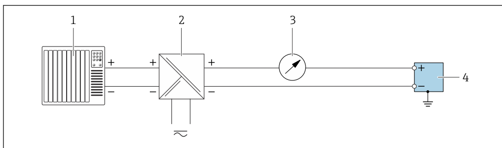
15 Exemple de raccordement pour sortie courant 4 ... 20 mA (passive)
