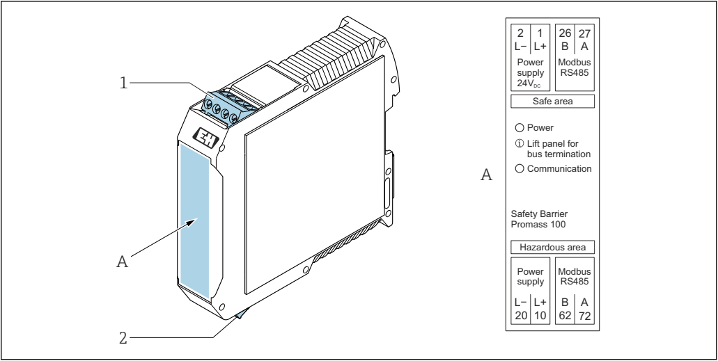
8 Promass 100 安全バリア、端子付き 1 非危険場所：ゾーン 2、Class I、Division 2 2 本質安全区域
