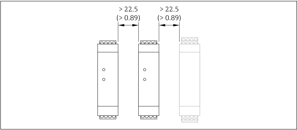
図 14 追加の Promass 100 安全バリアまたはその他のモジュールとの最小距離。単位 mm (in)
