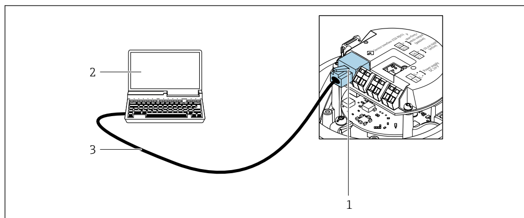
図 32 「出力」のオーダーコードの接続、オプション B : 4~20 mA HART、パルス/周波数/スイッチ出力
