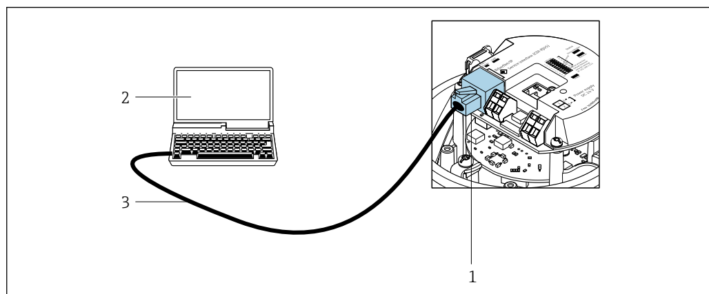
図 33 「出力」のオーダーコードの接続、オプション L : PROFIBUS DP
