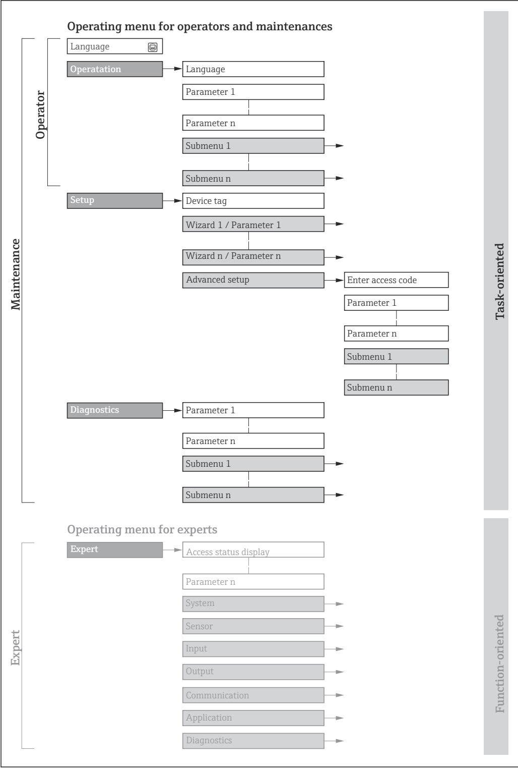
図 9 操作メニューの概要構成
