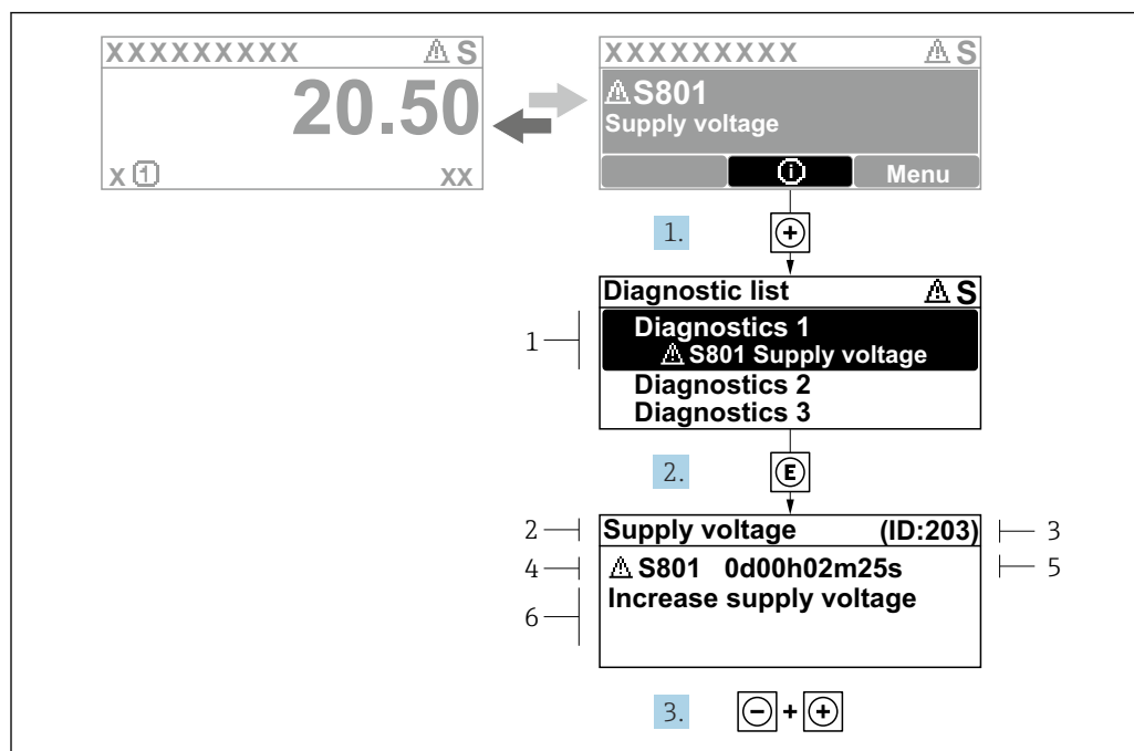
図 16 対処法のメッセージ
