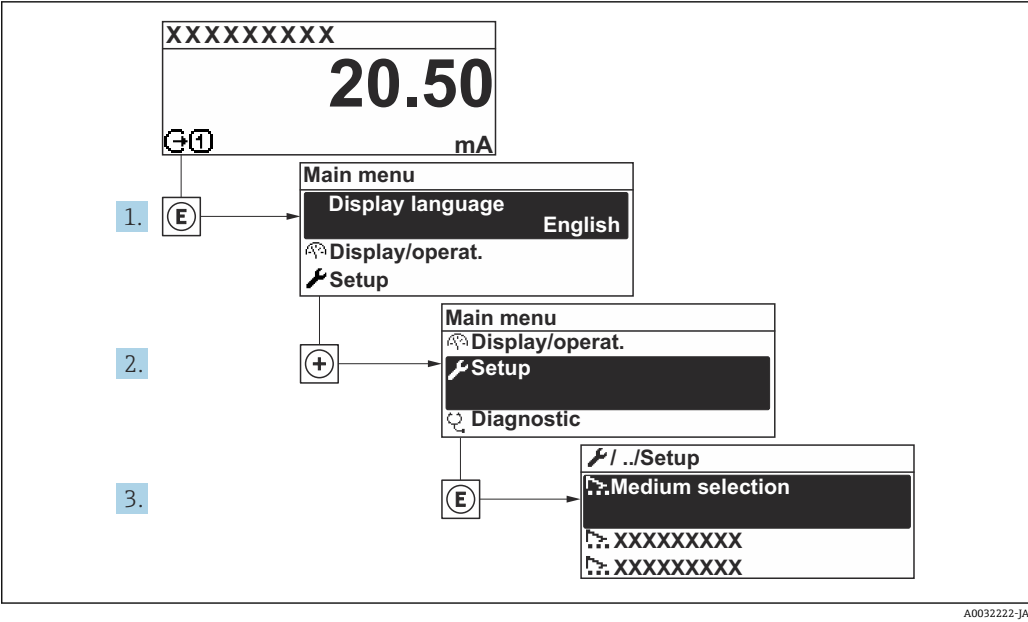
図 13 「設定」メニューへのナビゲーション（現場表示器の表示例）
