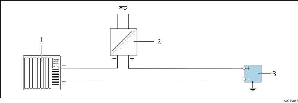
図 7 パルス出力/周波数出力/スイッチ出力（パッシブ）の接続例
