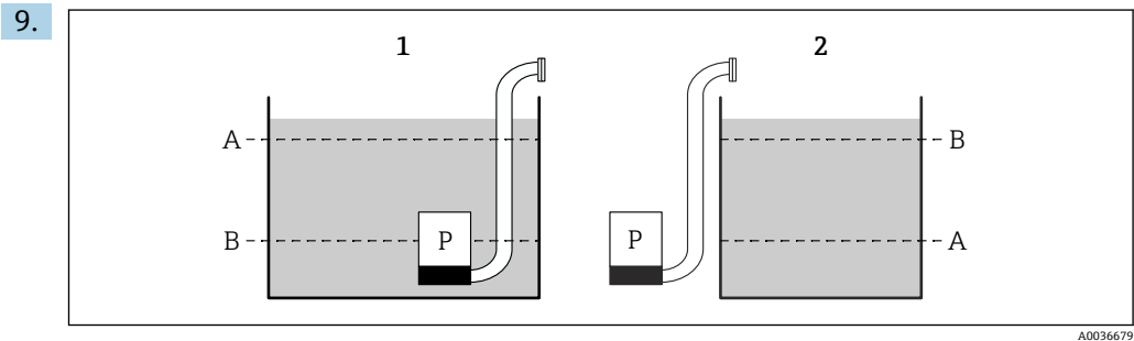
图 61 限位控制的开启点和关闭点
