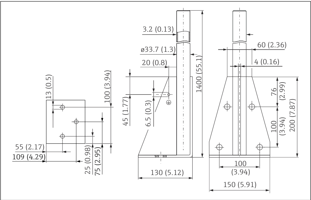
71 外形尺寸。测量单位 mm (in)
