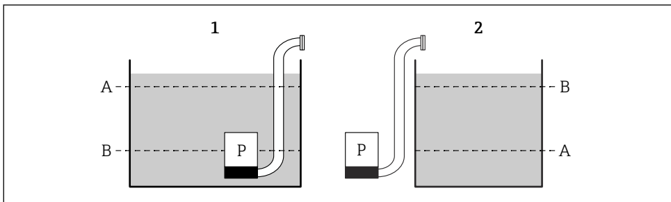
57 限位控制的开启点和关闭点
