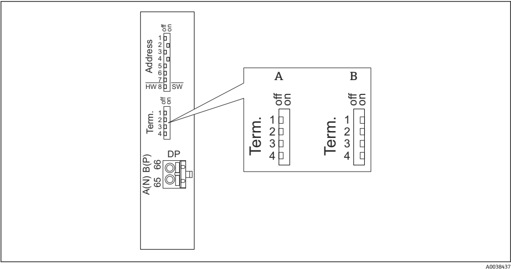
图 45 设备上的总线端接
