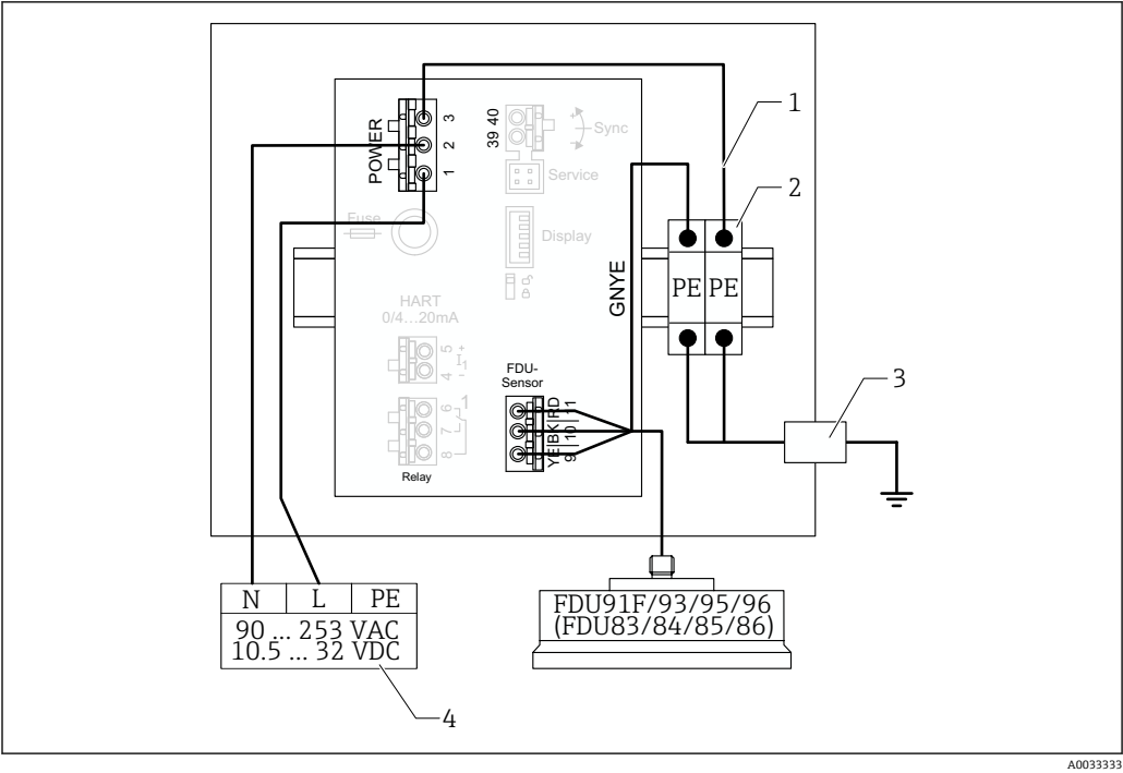
27 铝现场型外壳内金属探头的等电势 1 现场型外壳中的等电势；交付时已接线 2 保护性接地端子接线排（带有与 DIN 导轨接触的触点） 3 现场型外壳外部的保护性接地端 4 电源
