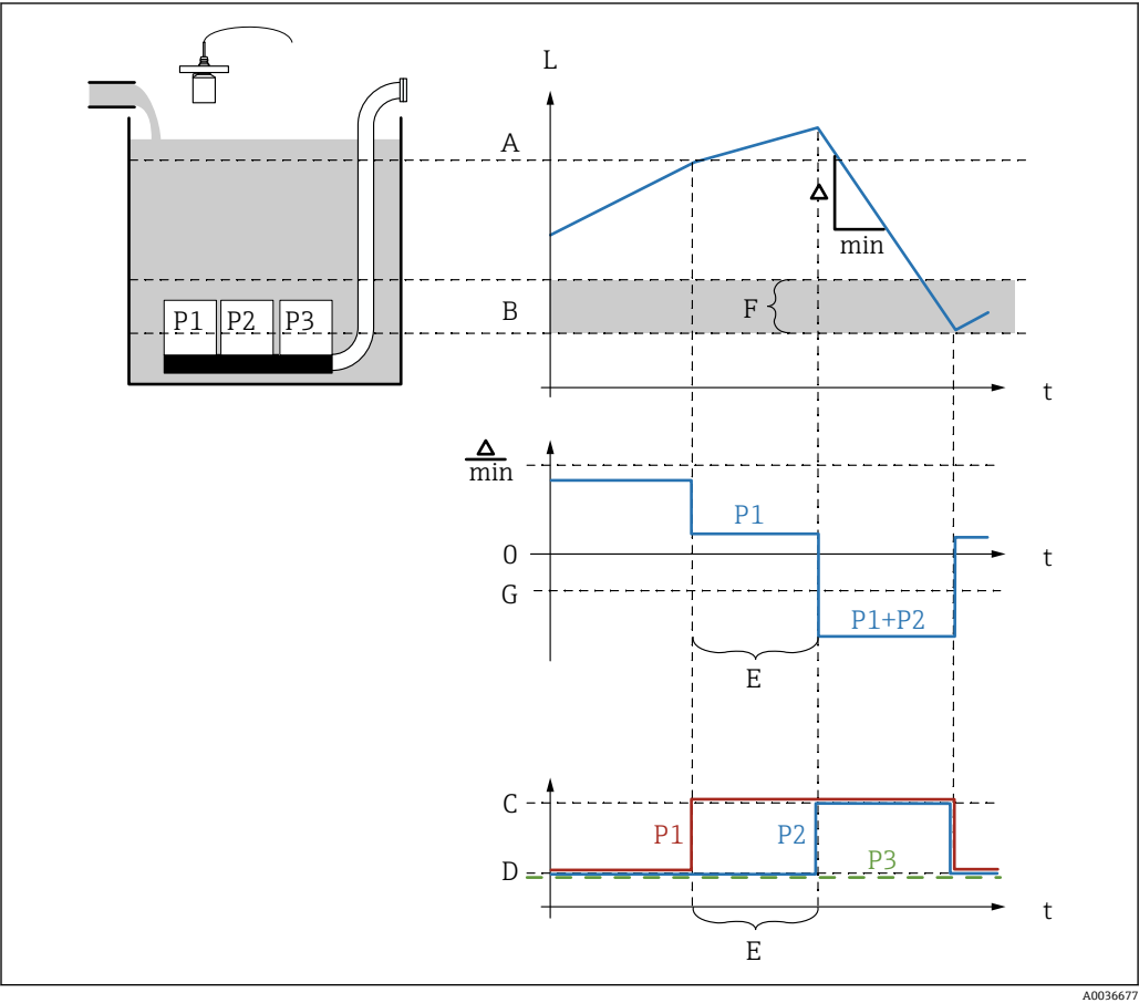
图 59 泵速控制工作原理
