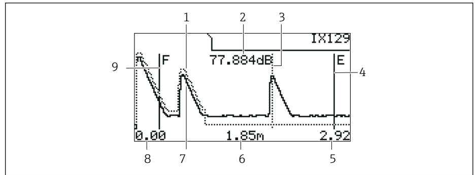
图 67 现场显示单元上的包络线
