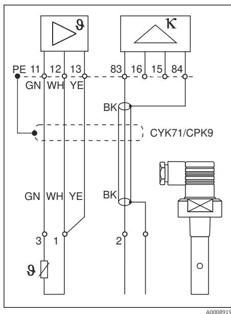
7 Tilslutning af konductive sensorer
