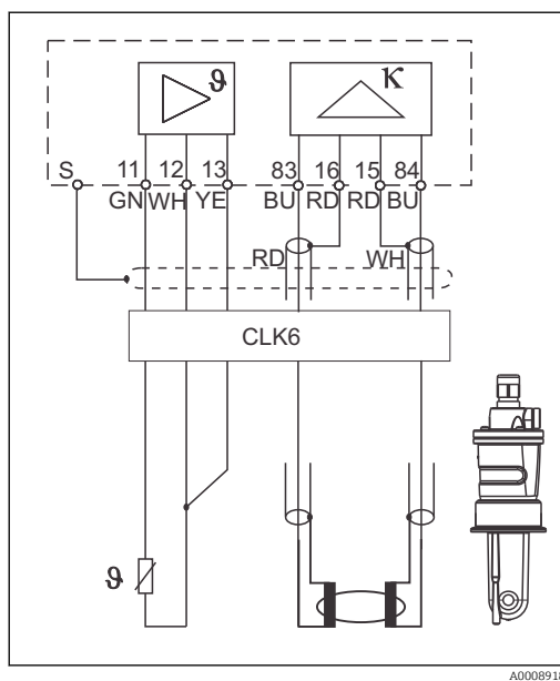
8 Tilslutning af induktive sensorer
