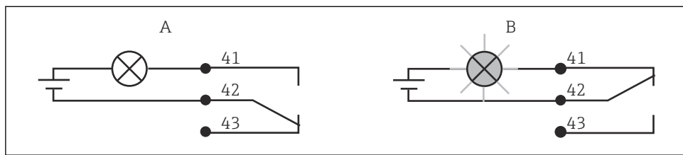
9 Anbefalet fejlsikker afbryder for alarmkontakten
