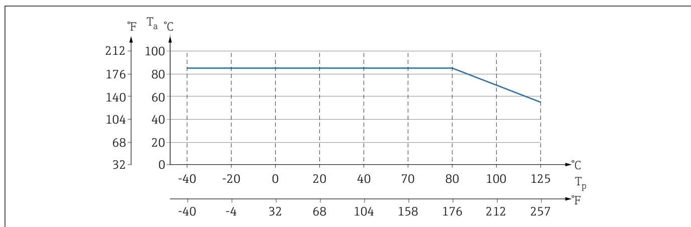
図 12 断熱材を使用しない垂直取付時の値
