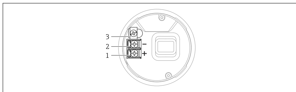
図 6 端子部の接続端子と接地端子
