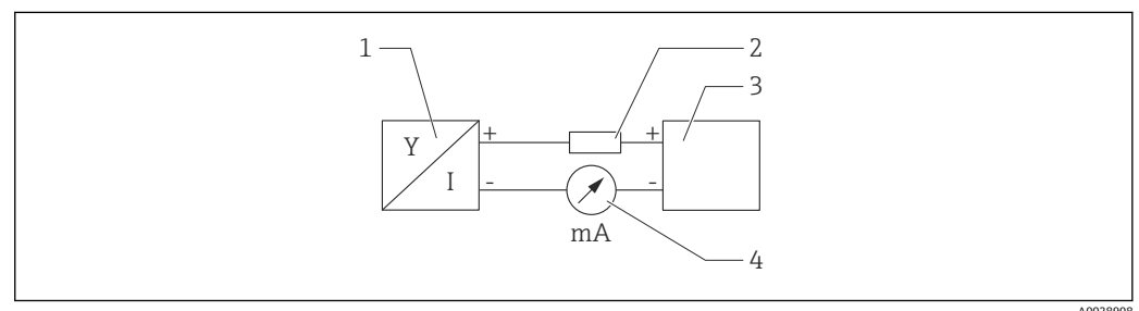
図 5 ブロック図
