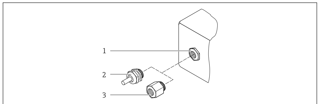
41 允许的电缆入口/缆塞
