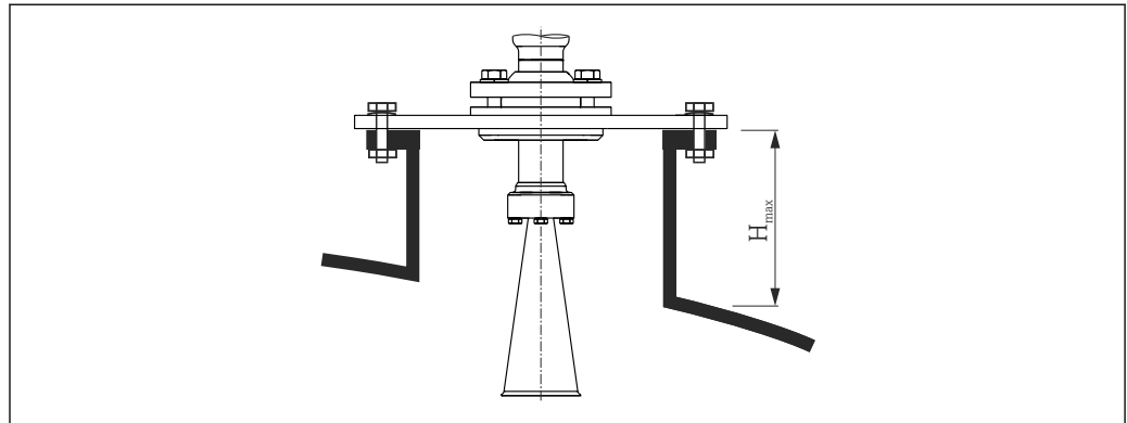
図 8 ホーンアンテナのノズル高 (FMR57)
