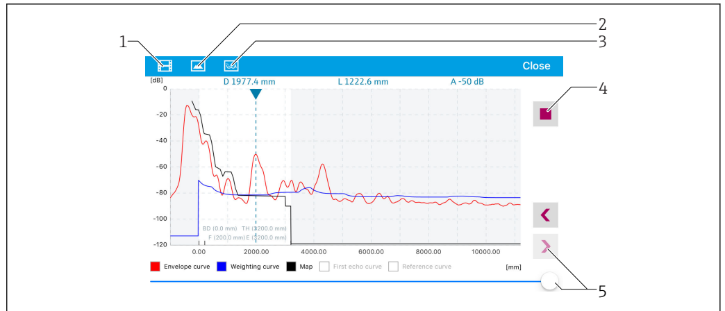
図 39 SmartBlue での反射波形表示 (例) ; iOS の表示
