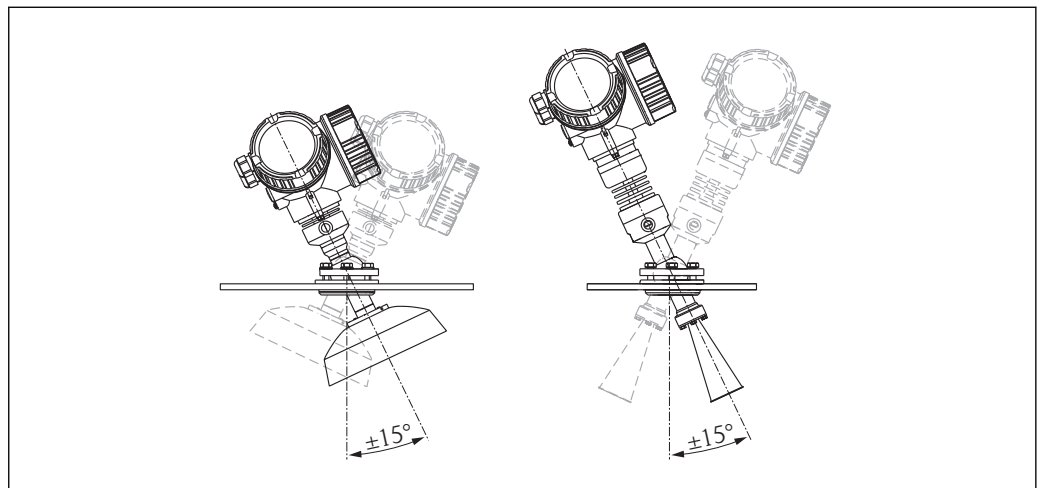
図 10 角度調節器付き Micropilot FMR57
