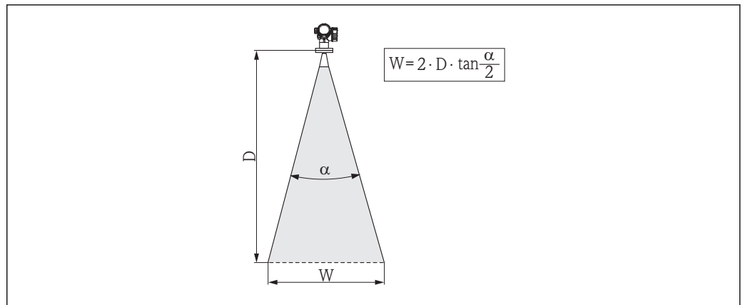
図 5 ビーム放射角 \alpha 、距離 D およびビーム幅 W の関係
