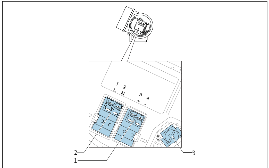
図 20 4 線式、4~20 mA HART の端子割当て (90~253 V AC )
