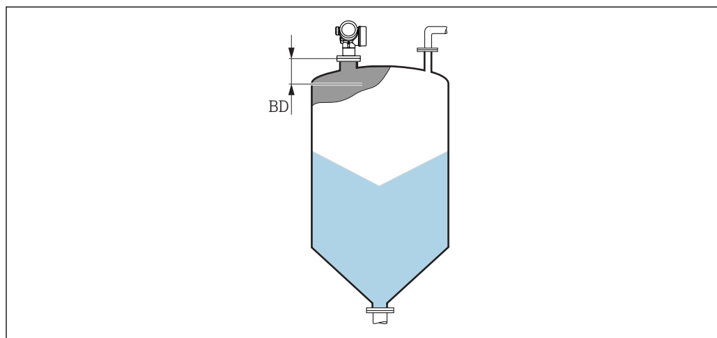
図 55 粉体計測の不感知距離 (BD)
