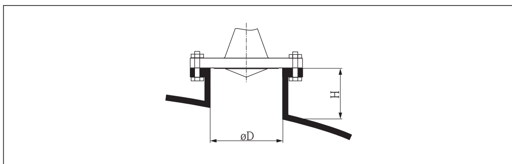
図 6 スリップオンフランジ付きホーンアンテナのノズル高と直径
