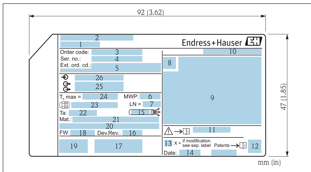
図 4 Micropilot の銘板
