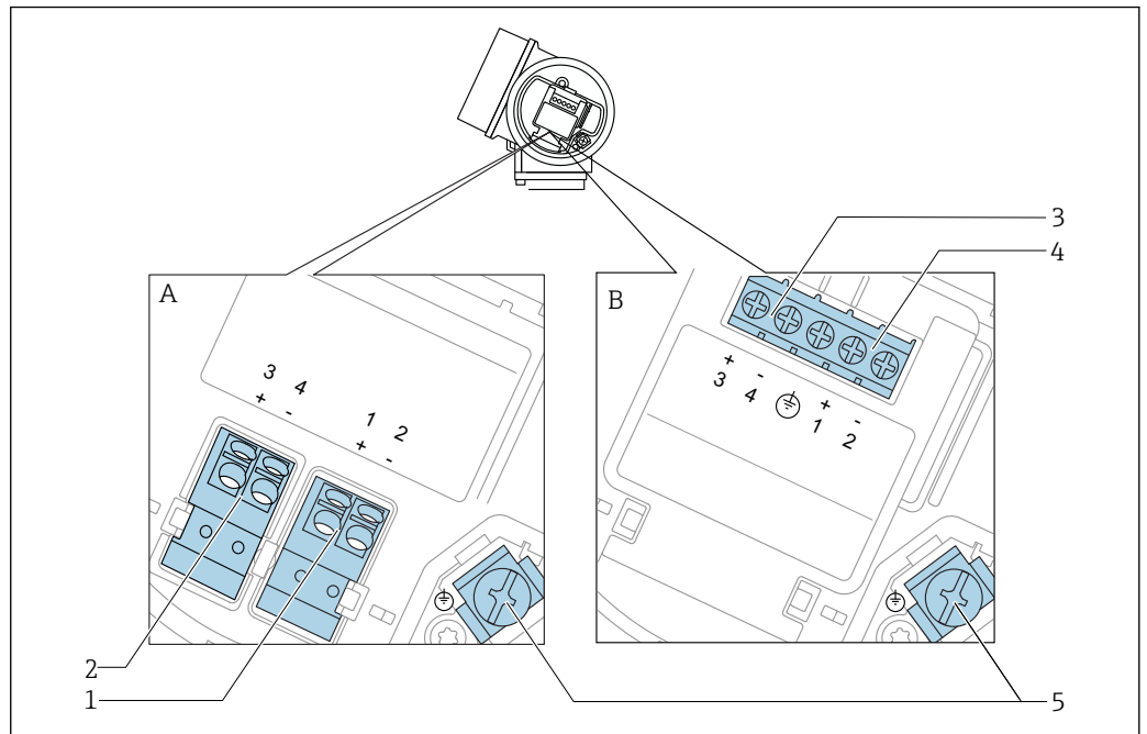
図 16 2線式、4~20 mA HART、4~20 mA の端子割当て
