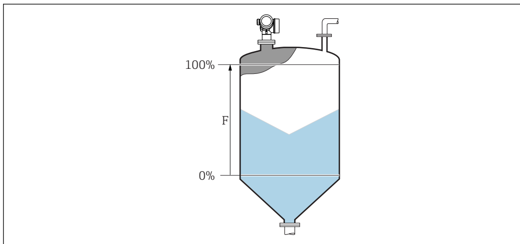
48 粉体レベル測定用の満量校正 (F)
