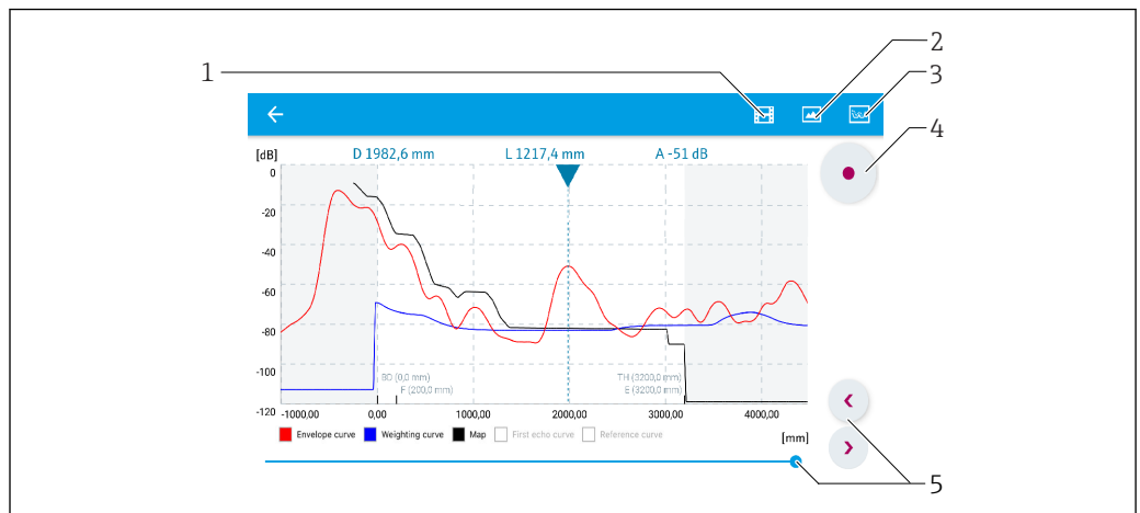
図 38 SmartBlue での反射波形表示 (例) ; Android の表示
