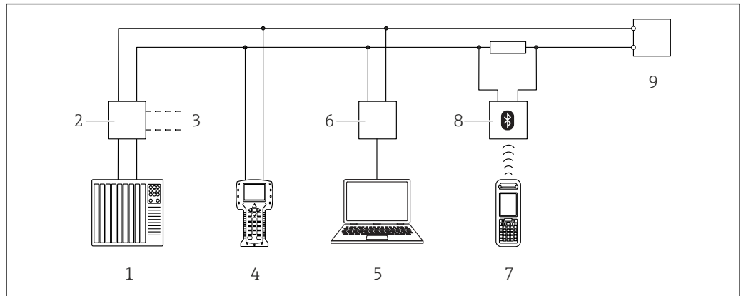
図 29 HART 経由のリモート操作オプション
