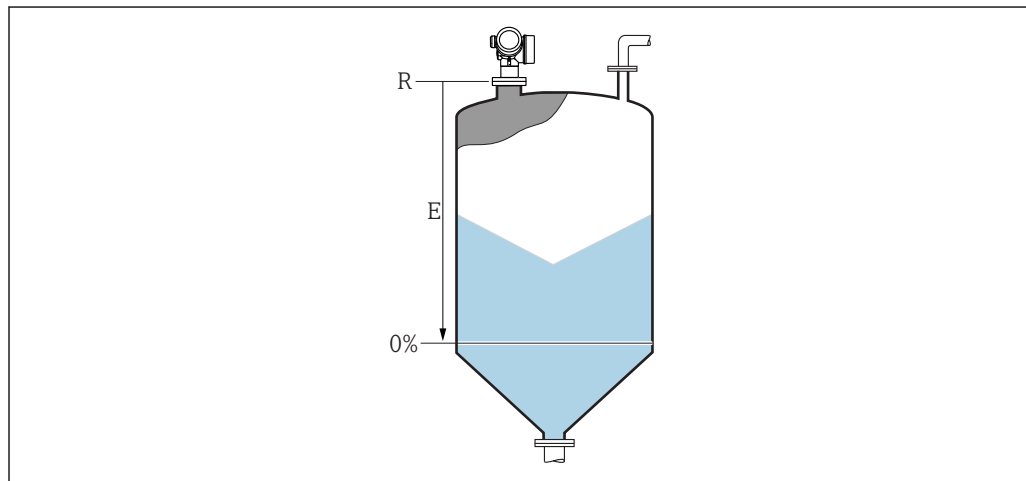
☑ 47 粉体レベル測定用の空校正 (E)
