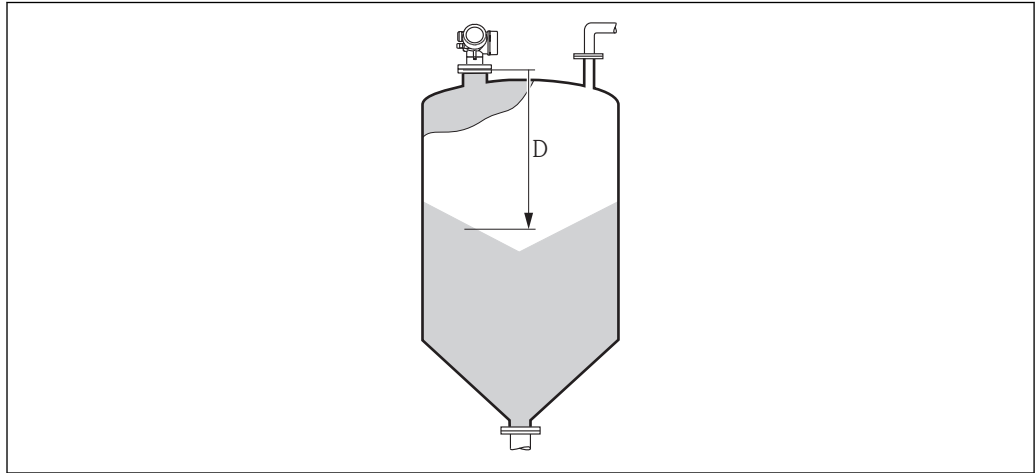
☑ 50 粉体測定の距離
