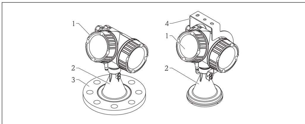
図 1 Micropilot FMR56 (26 GHz) の構成
