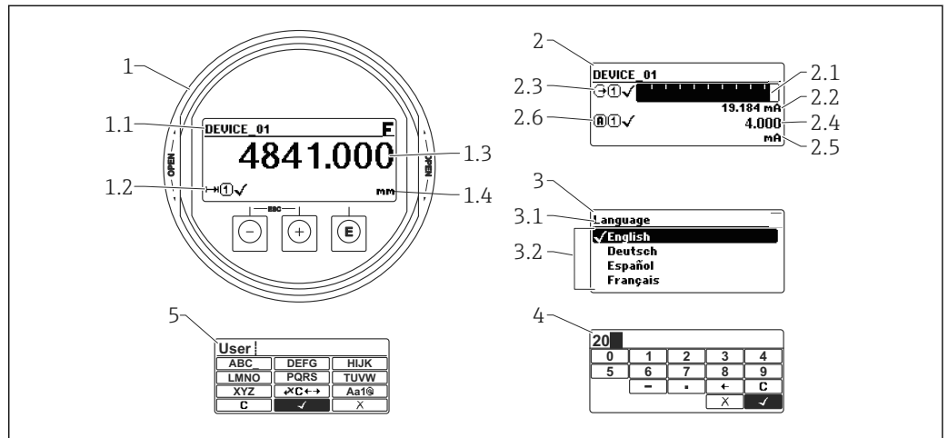
図 31 現場操作用の表示部および操作モジュールの表示
