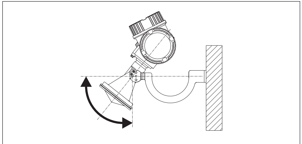
図 7 取付ブラケット付きホーンアンテナの設置
