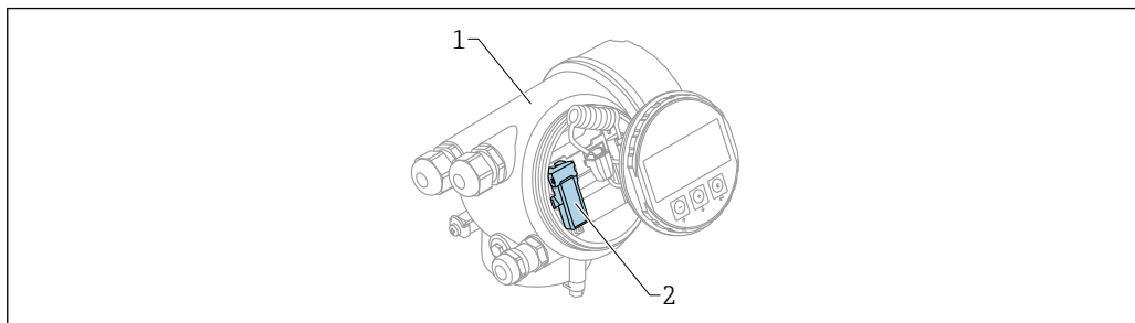
図 27 Bluetooth モジュール搭載の機器
