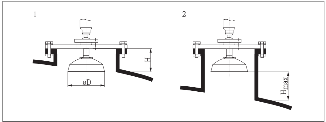
図9 パラボラアンテナ付き Micropilot FMR57 のノズル取付け
