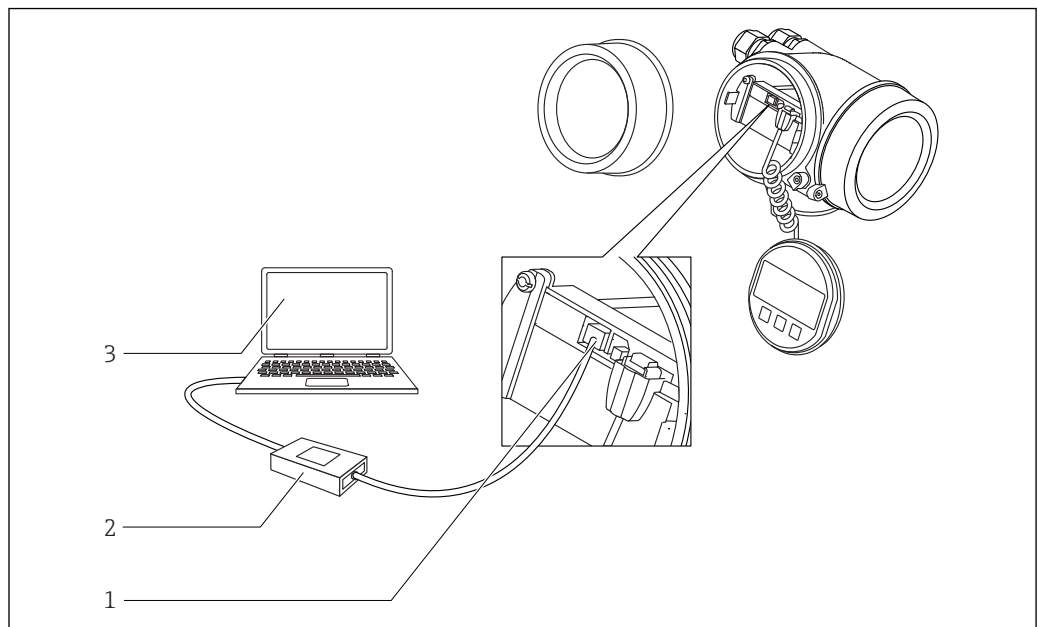
図 30 サービスインターフェイス (CDI) 経由の DeviceCare/FieldCare
