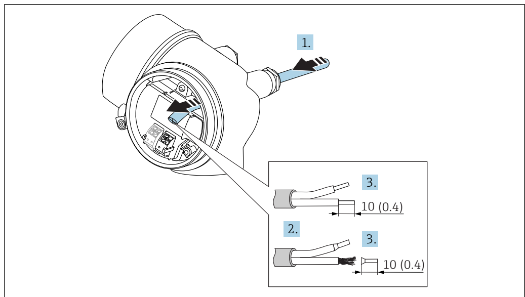
図 24 寸法単位 : mm (in)
