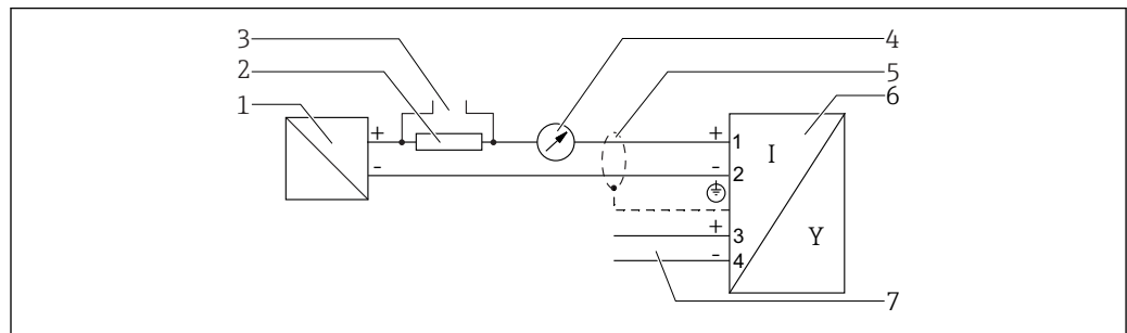
図 15 ブロック図：2線式、4~20 mA HART、スイッチ出力
