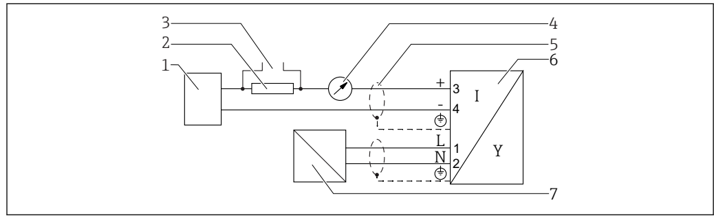
図 21 ブロック図：4線式、4~20 mA HART (90~253 V AC )
