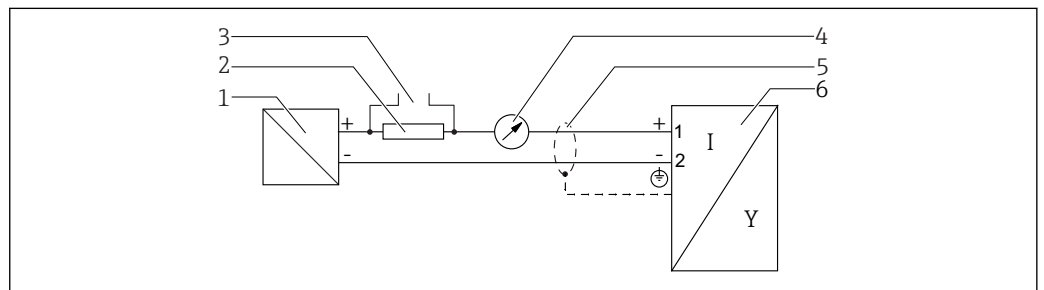
図 13 ブロック図：2 線式、4~20 mA HART
