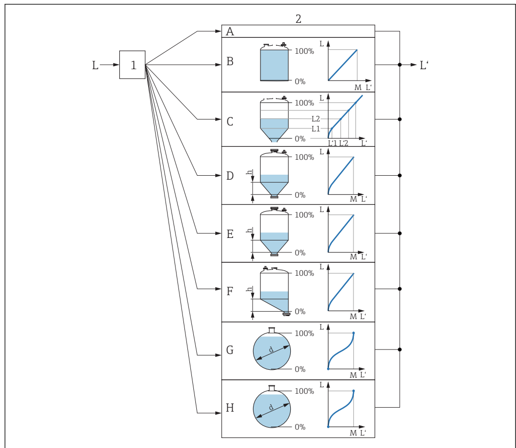
図 53 リニアライゼーション：レベルおよび界面の高さ（該当する場合）を容量または質量に変換します。これは容器の形状に応じて異なります。
