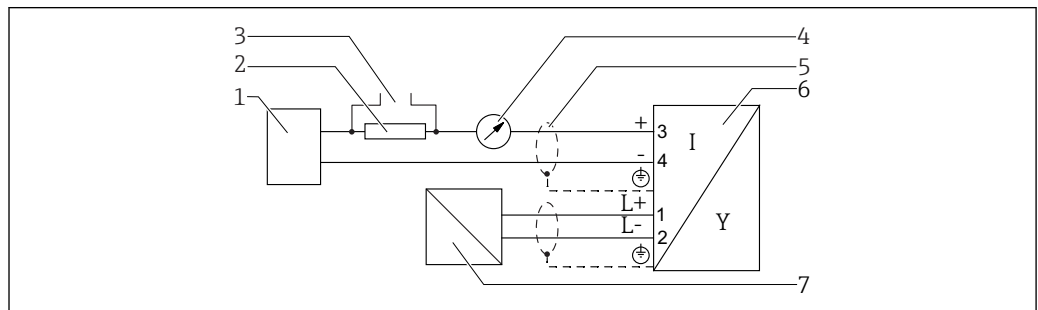
図 19 ブロック図：4線式、4~20 mA HART (10.4~48 V DC )
