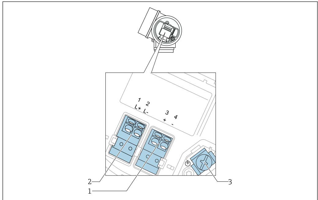
図 18 4線式、4~20 mA HART の端子割当て (10.4~48 V DC )
