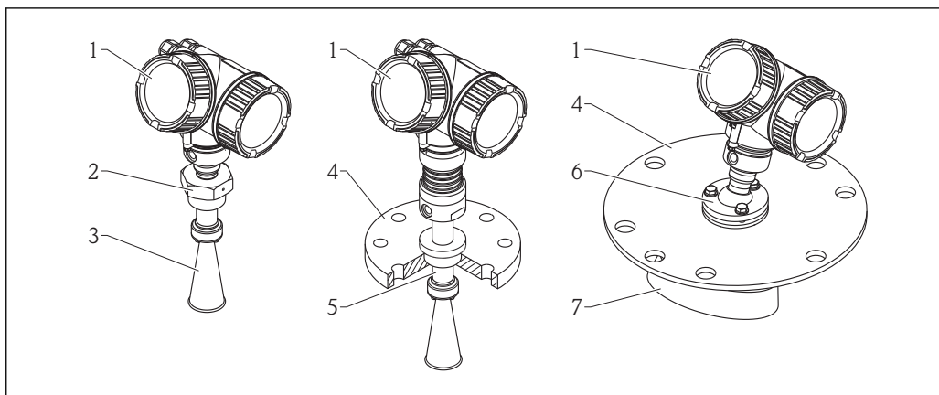
図 2 Micropilot FMR57 (26 GHz) の構成
