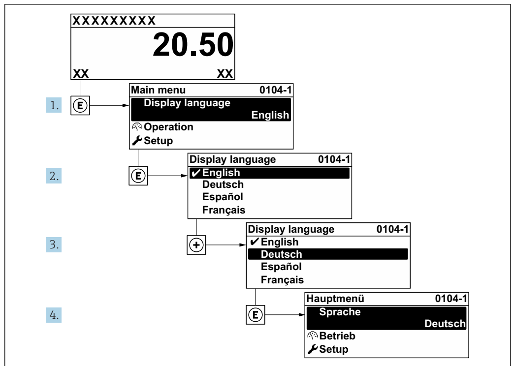
40 現場表示器の言語設定の例
