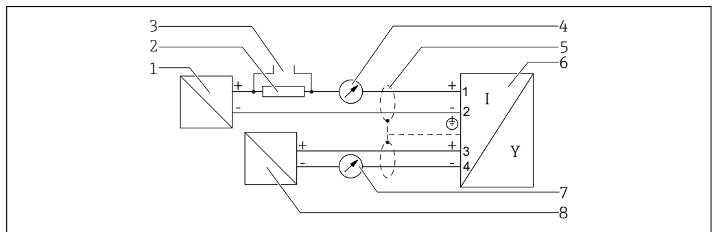
図 17 ブロック図：2線式、4~20 mA HART、4~20 mA
