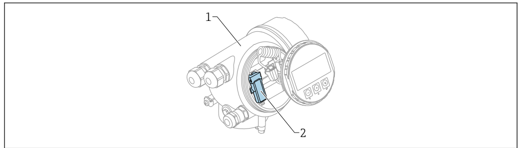
図 32 Bluetooth モジュール搭載の機器
