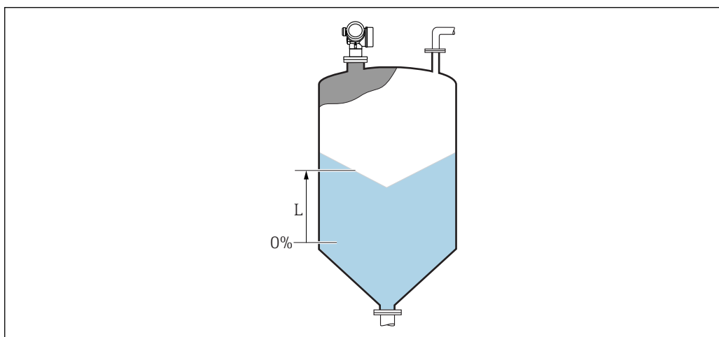
49 粉体計測時のレベル
