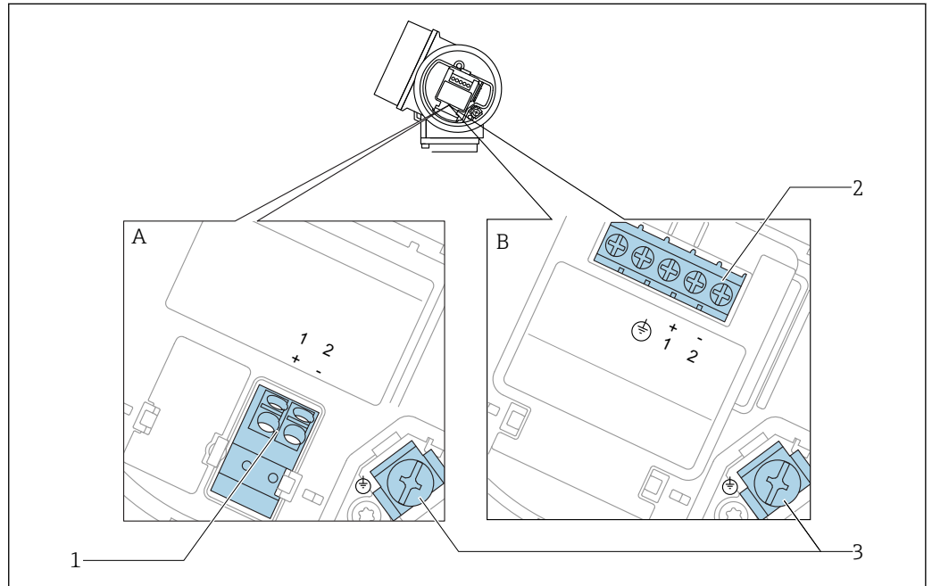
図 12 2 線式、4-20 mA HART の端子割当て
