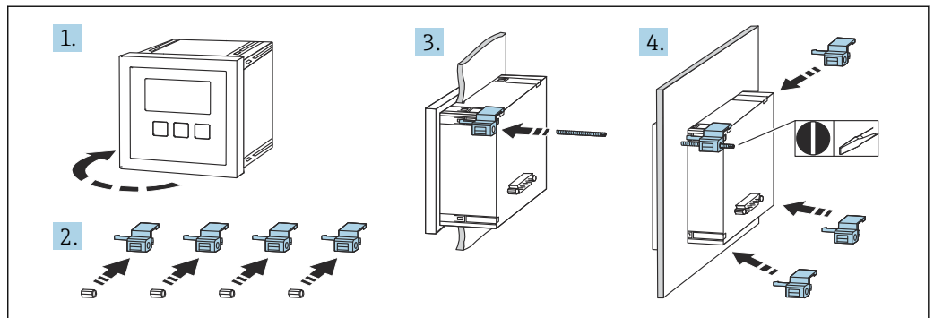
図 15 リモートディスプレイと操作モジュールの取付け
