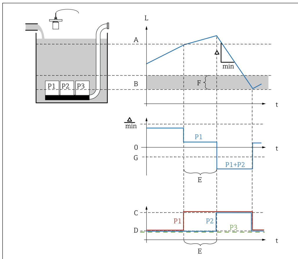
図 59 ポンププレート制御の動作原理
