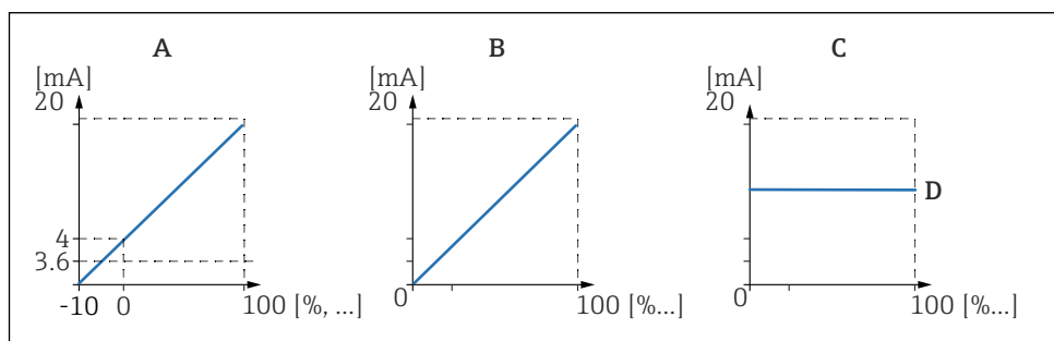
図 66 電流スパン
