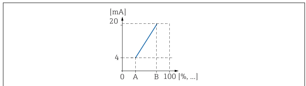
図 69 電流ターンドアンの動作原理
