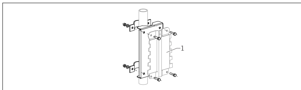
図 73 ポリカーボネート製フィールドハウジング用の取付プレート
