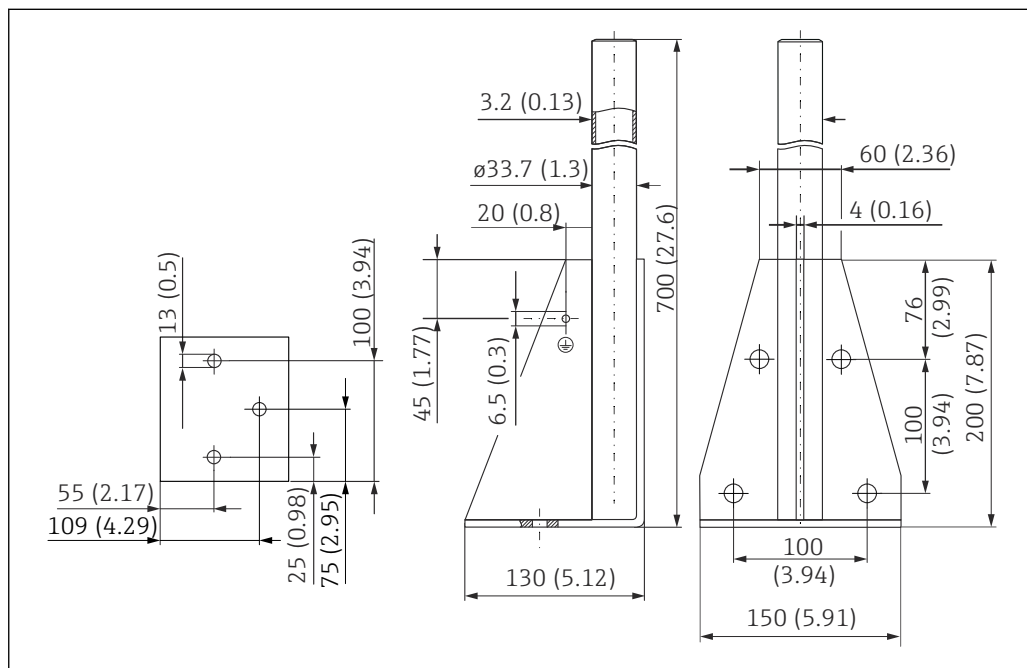
74 寸法。測定単位 mm (in)
