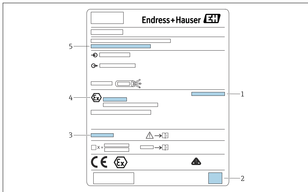
図 5 銘板
