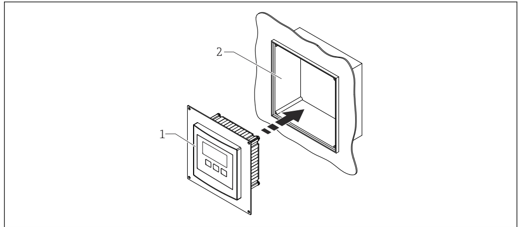
図 14 FMU860/861/862 の分離型ディスプレイの取付け
