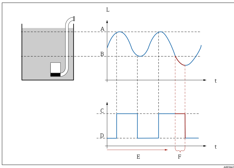
図 60 「反動間隔」および「反動時間」の影響
