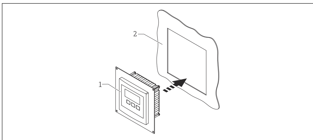
図 76 アダプタプレートを使用
