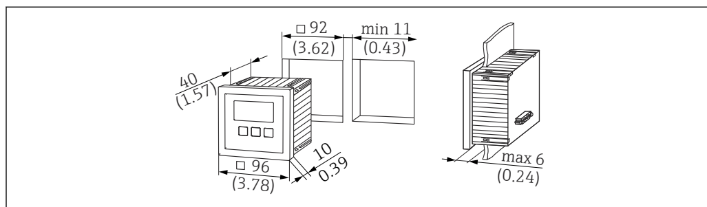
図 13 分離型ディスプレイと操作モジュール用の開口部。測定単位 mm (in)
