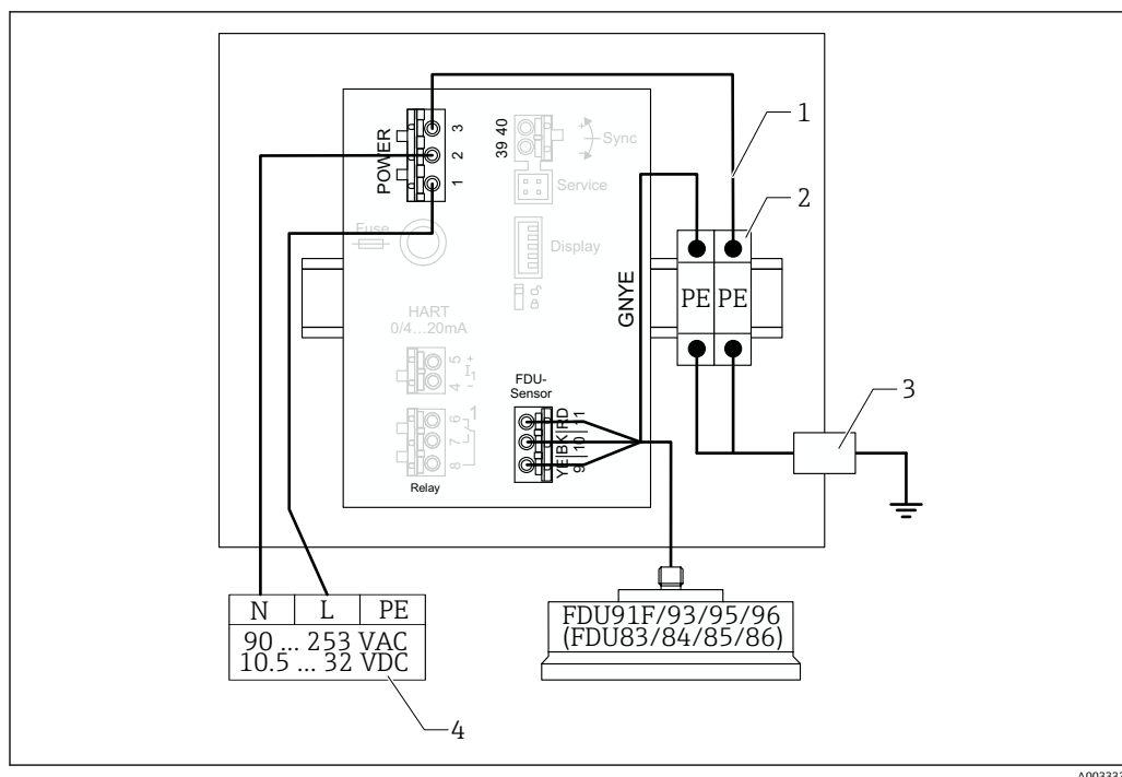
27 アルミニウム製フィールドハウジング内の金属製センサの電位平衡
