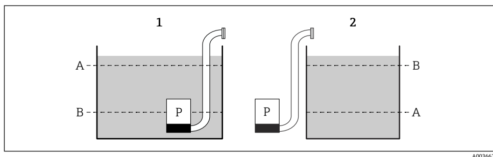
図 61 リミット制御用のスイッチオンポイントとスイッチオフポイント
