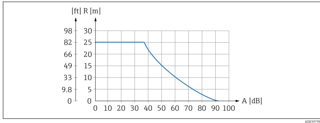
2 Rækkeviddediagram for ultralydssensorer
