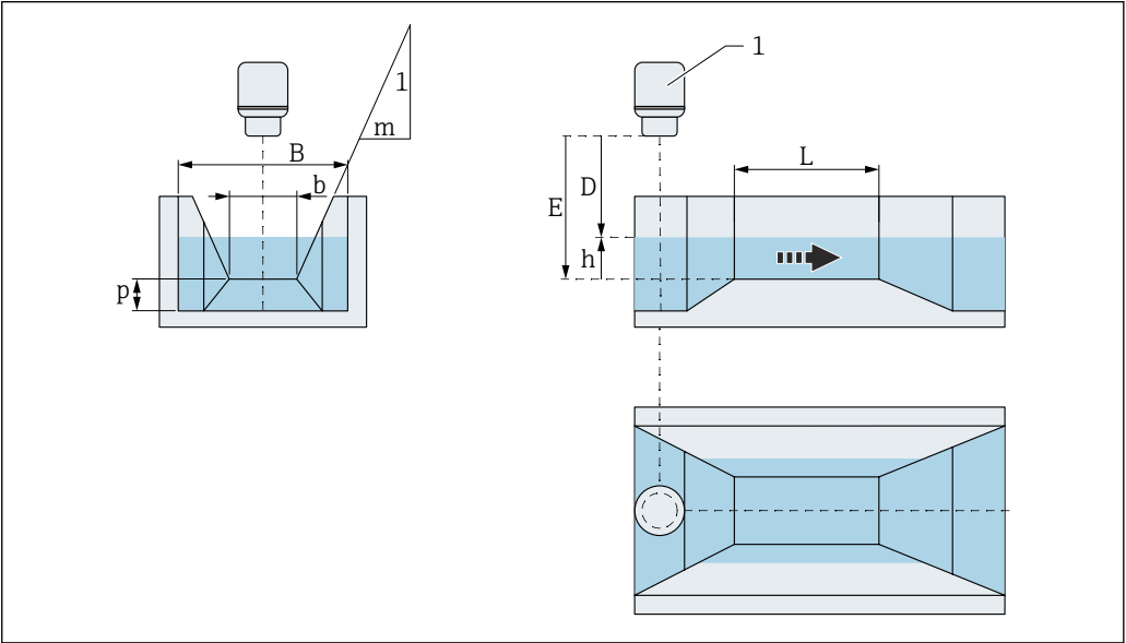
101 Gerinnetyp: Trapezrinne (ISO 4359)
