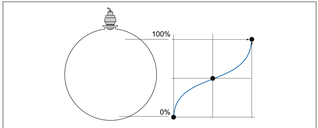
69 Linearisierungsart: Kugeltank
