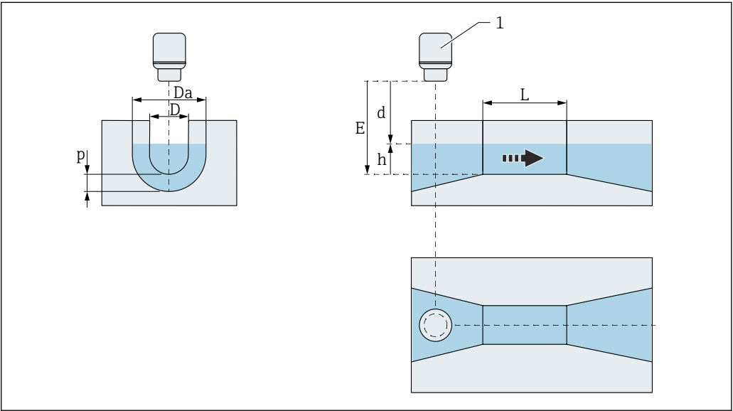
105 Gerinnetyp: U-Form-Rinne (ISO 4359)
