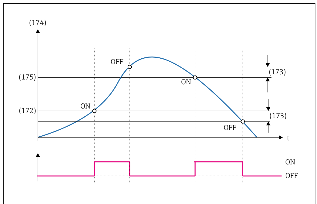
154 Funktion 'Inband'
