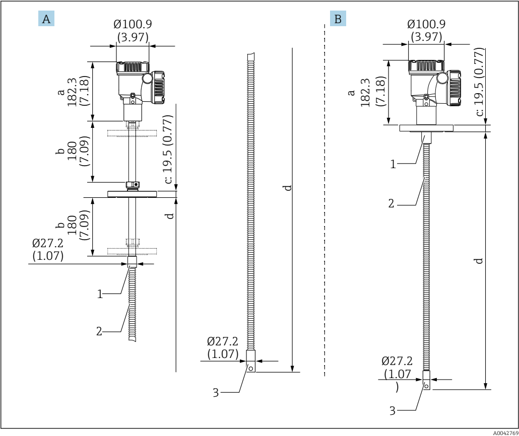
6 Преобразователь с зондом для измерения средней температуры. Единица измерения мм (дюйм) A Регулируемый фланец B Приварной фланец a Высота преобразователя b Регулируемая монтажная высота c Основывается на стандартах изготовления фланцев d Длина температурного зонда (см. ниже) 1 316L 2 316L 3 316L
