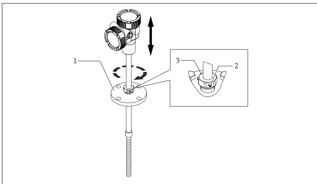
21 Прибор NMT81 с регулятором высоты
