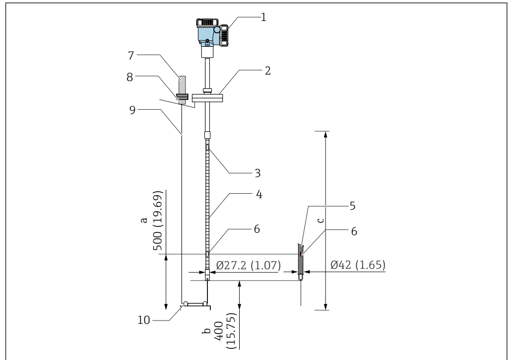
24 Метод с использованием верхнего анкера. Единица измерения мм (дюйм)
