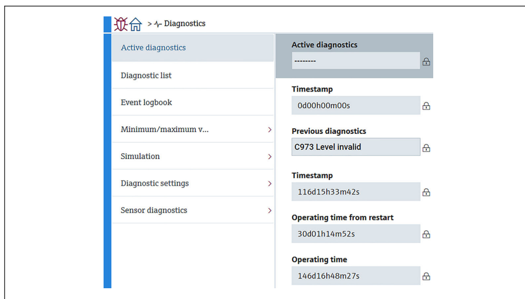
105 Экран Диагностика активна
