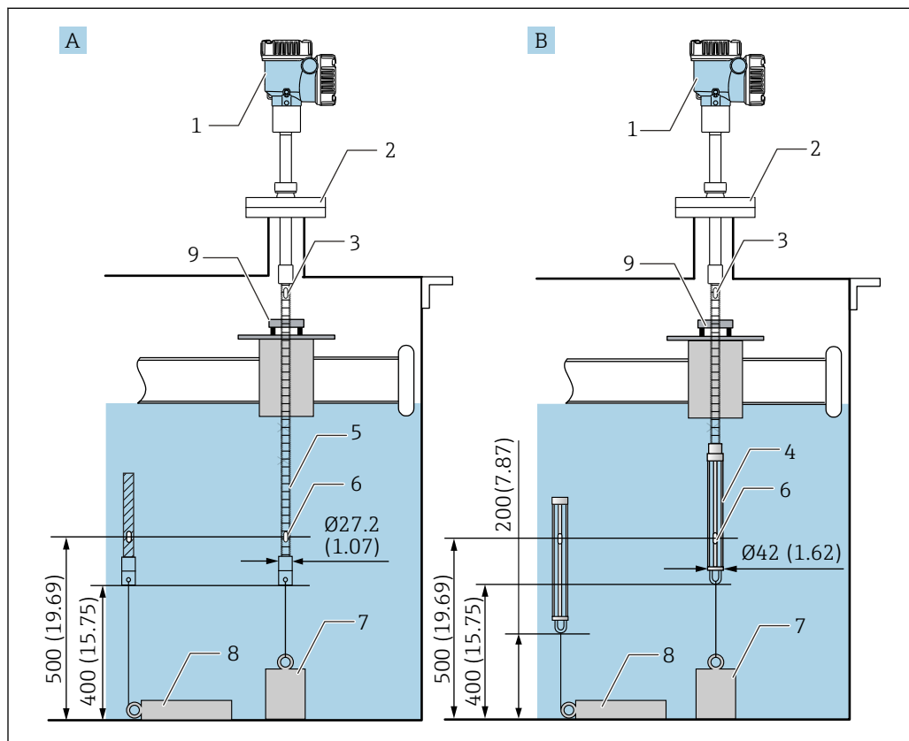
32 Метод с использованием направляющего кольца и якорного груза. Единица измерения мм (дюйм)
