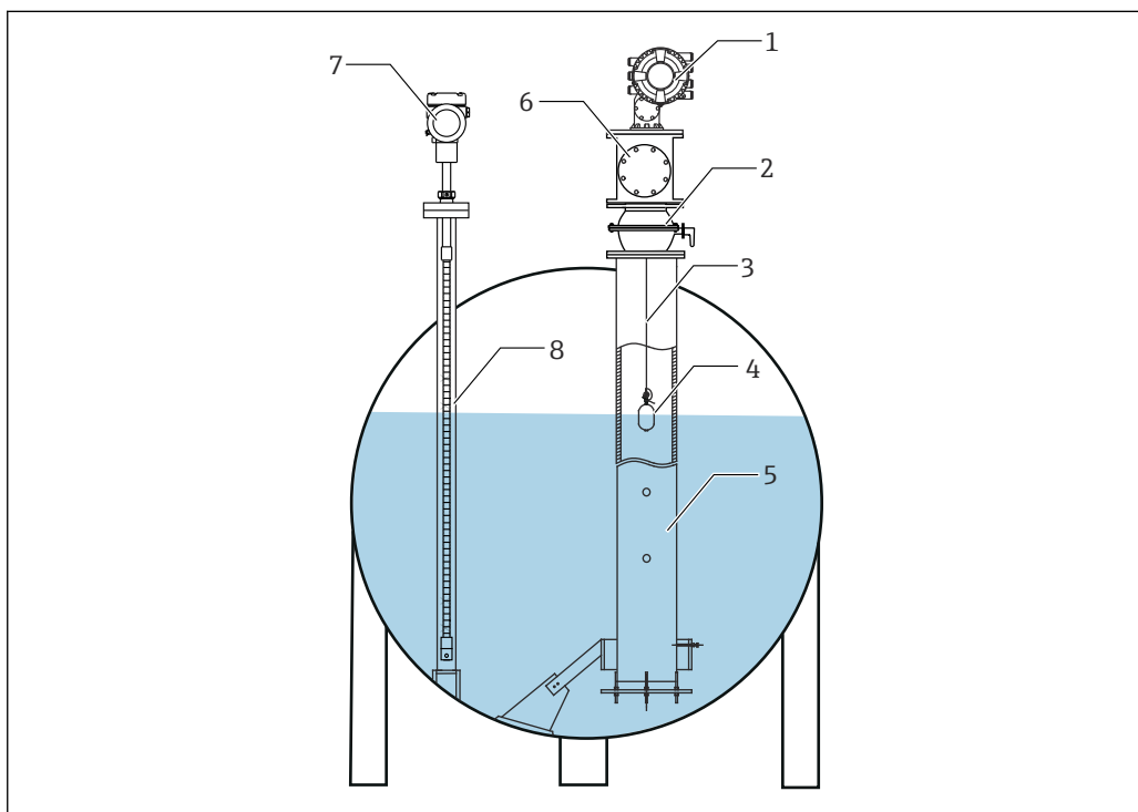
33 Термогильза для резервуара, работающего под давлением
