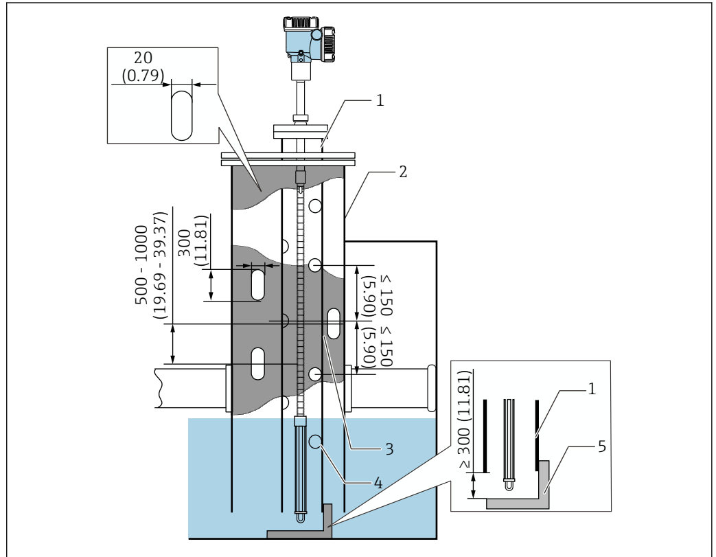
31 Метод с использованием успокоительной трубы. Единица измерения мм (дюйм)
