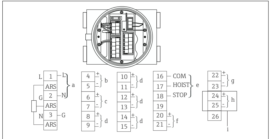
38 Клеммы прибора NMS5
