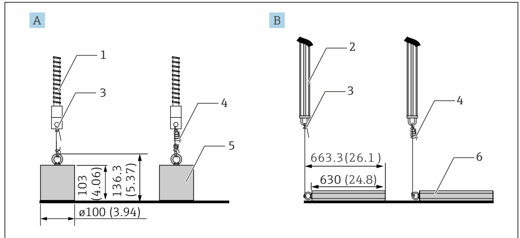
29 Монтаж якорного груза
