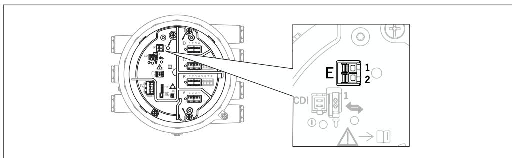
37 Клемма прибора NMS8x для преобразователя NMT81
