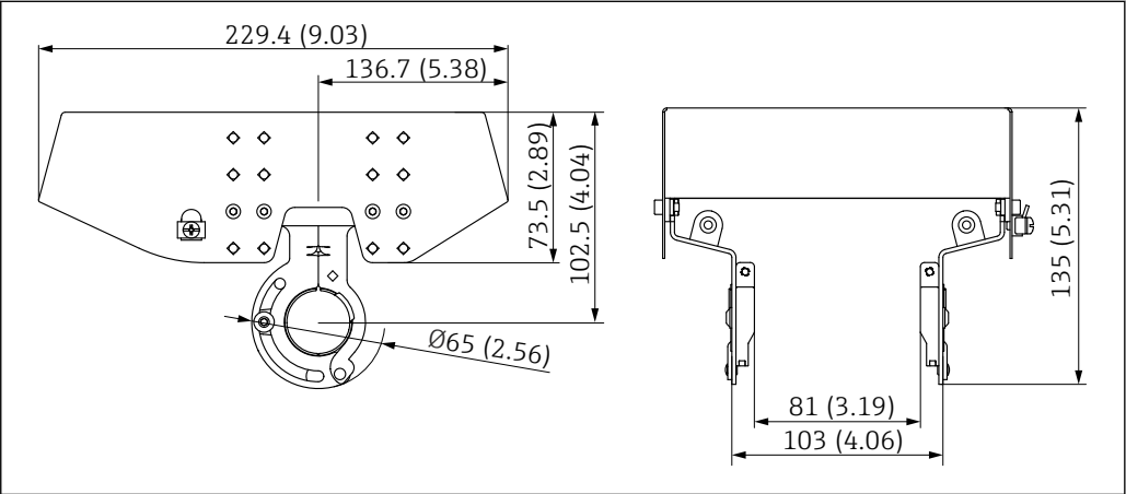
114 Защитный козырек от атмосферных явлений. Единица измерения мм (дюйм)
