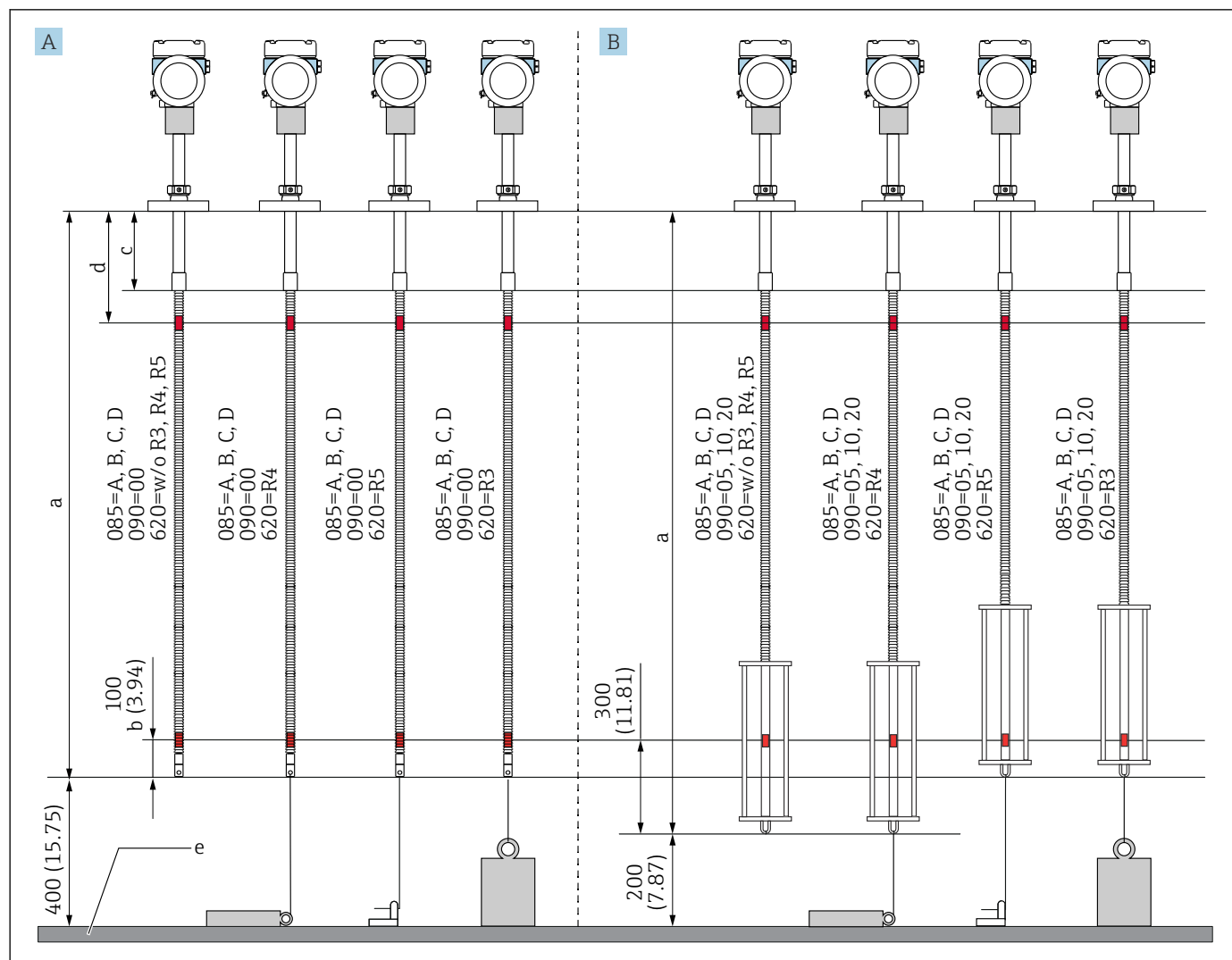
10 Положение чувствительного элемента № 1 прибора NMT81 в зависимости от метода монтажа. Единицы измерения мм (дюйм)
