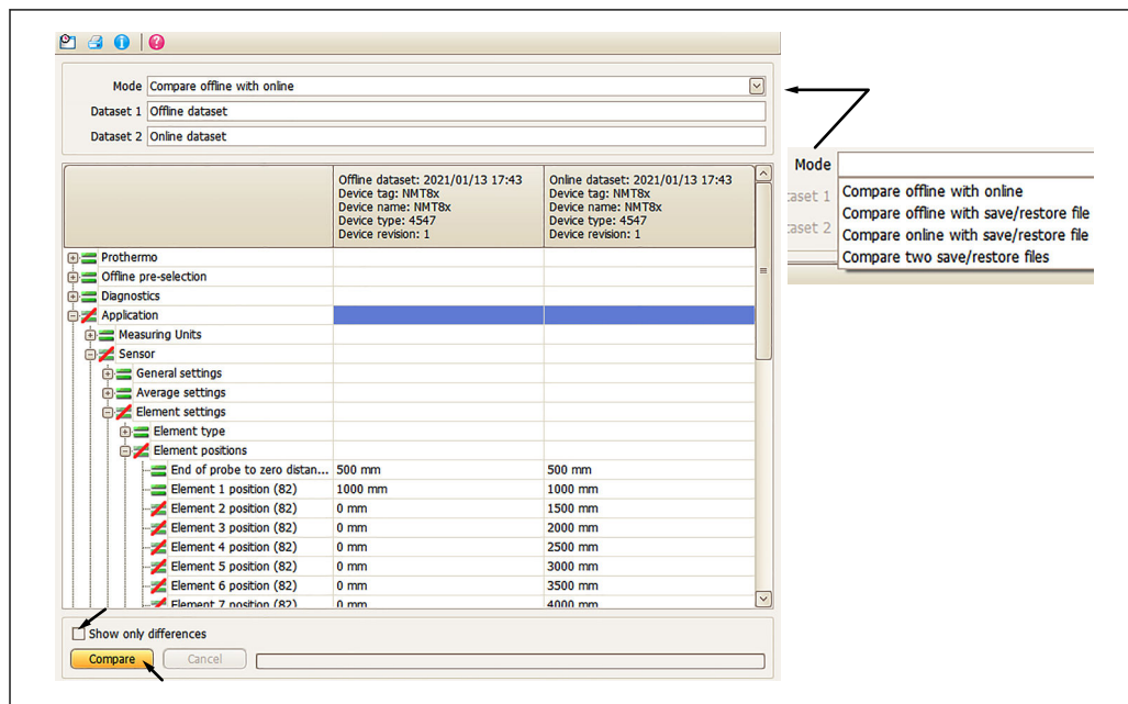
69 Экран сравнения наборов данных
