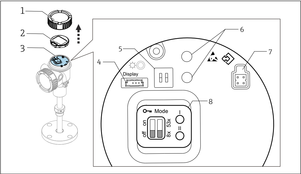
47 Электрический модуль
