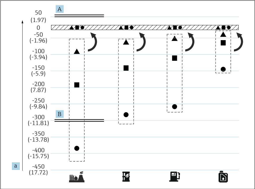
14 Влияние компенсации при наличии трех слоев A С компенсацией B Без компенсации a Максимальная погрешность уровня воды, мм (дюйм)
