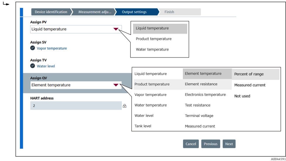
63 Экран настройки выхода
