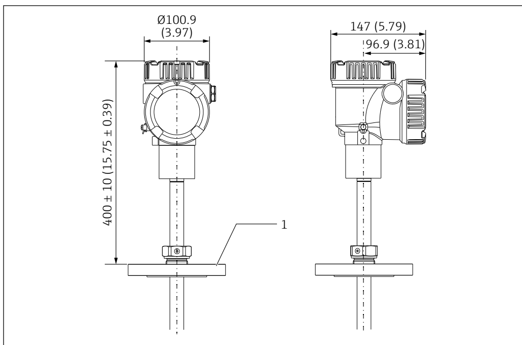
9 Регулируемый фланец. Единица измерения мм (дюйм)
