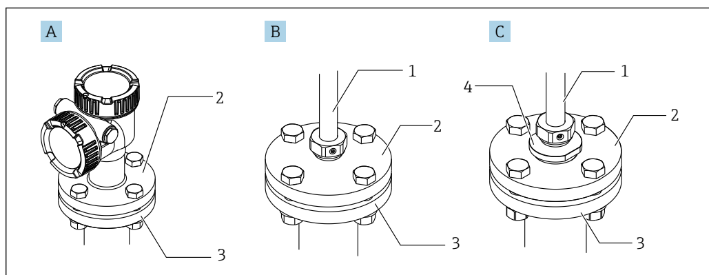
19 Фланцы
