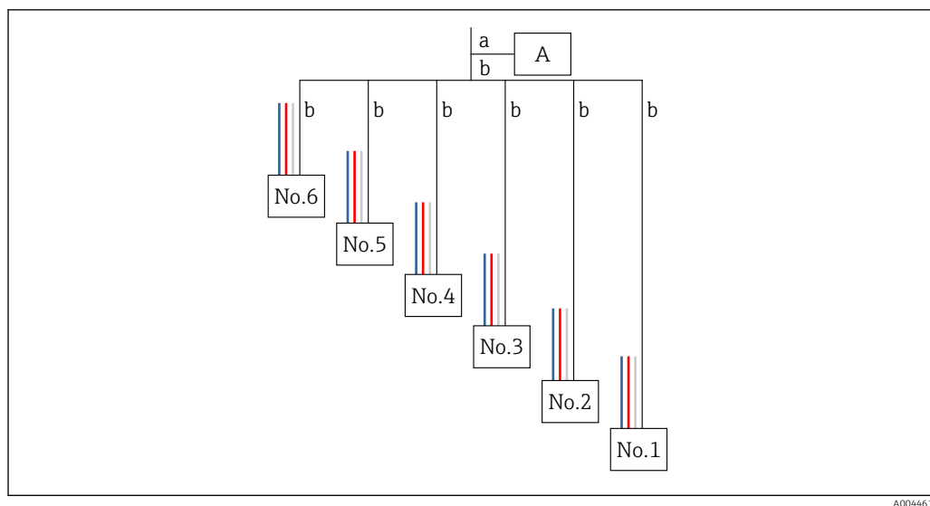
43 Структура четырехпроводного подключения
