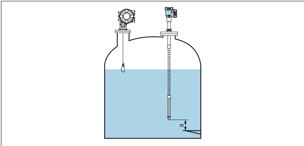
52 Положение температурно-чувствительного элемента в нижней точке
