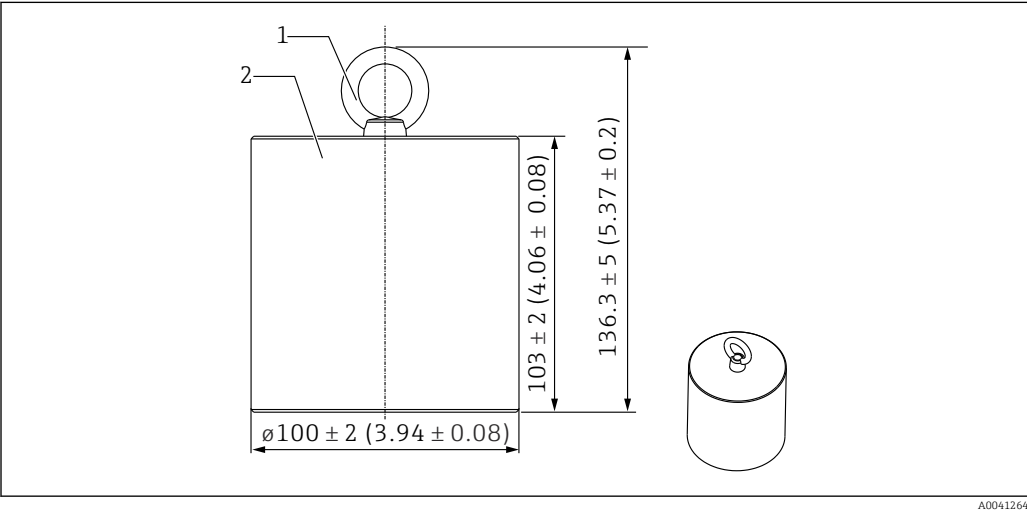
115 Монтажное приспособление. Единица измерения мм (дюйм)
