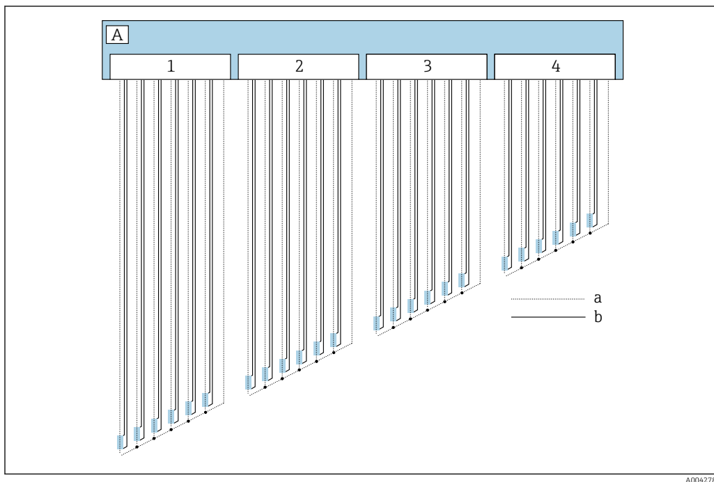
36 Схема четырехпроводного подключения
