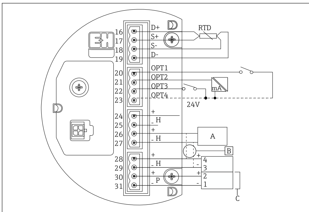
39 Искробезопасные клеммы прибора NRF590
