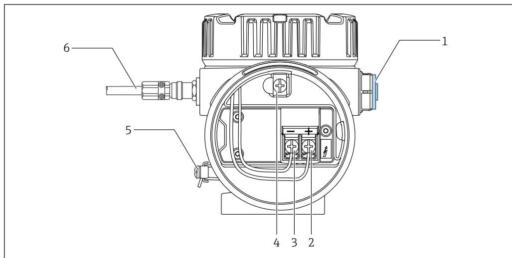
35 Клеммы прибора NMT81 (ATEX Ex ia)
