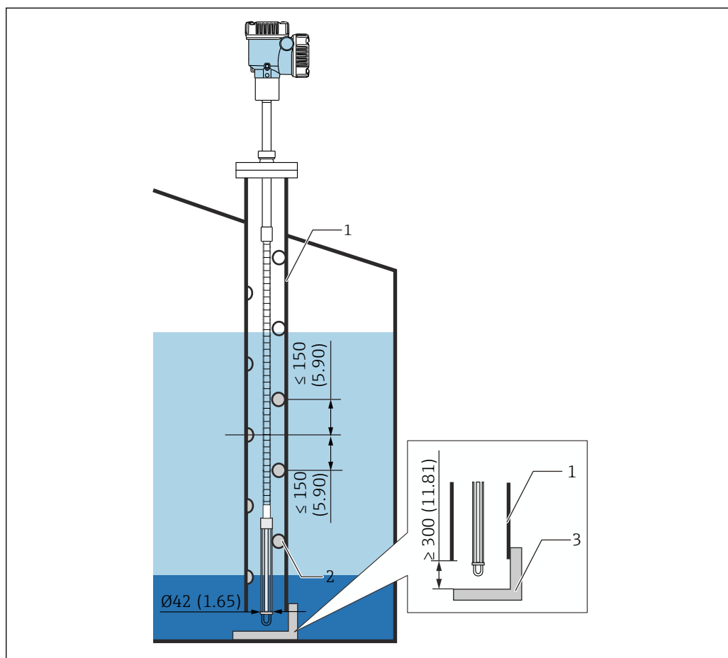
27 Успокоительная труба. Единица измерения мм (дюйм)
