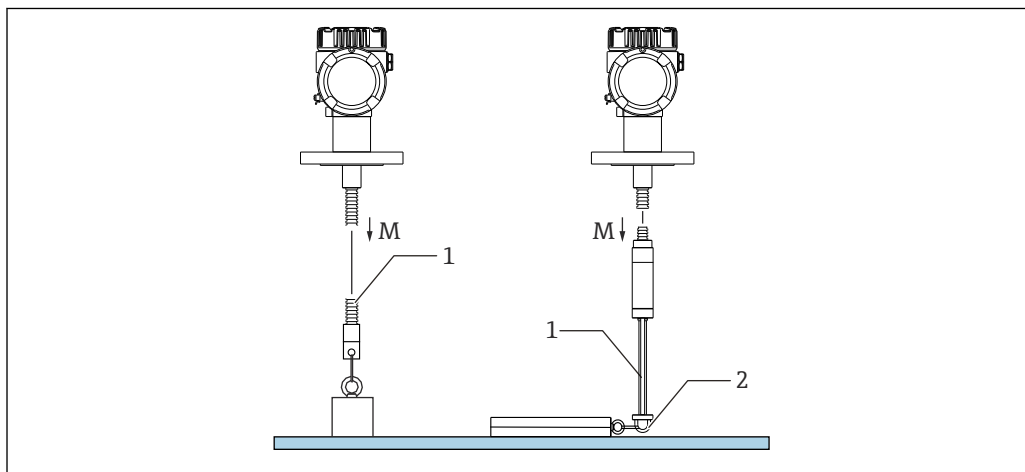
23 Монтаж якорного груза
