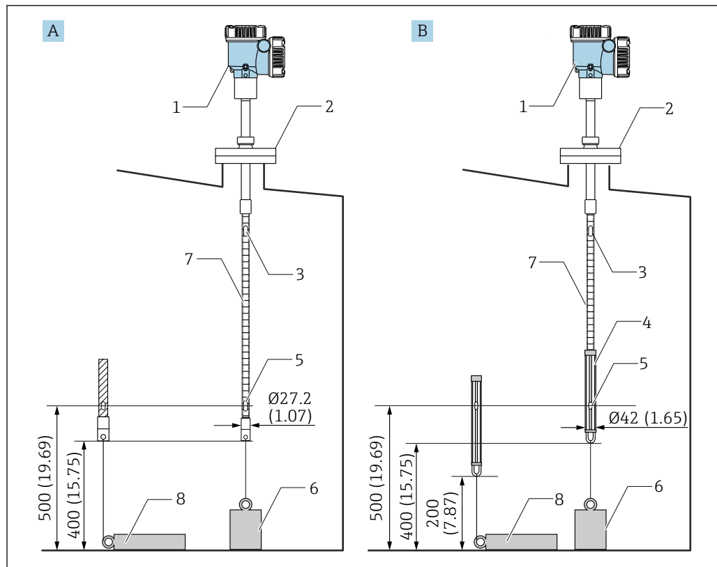
■ 28 Метод с использованием якорного груза. Единица измерения мм (дюйм)
