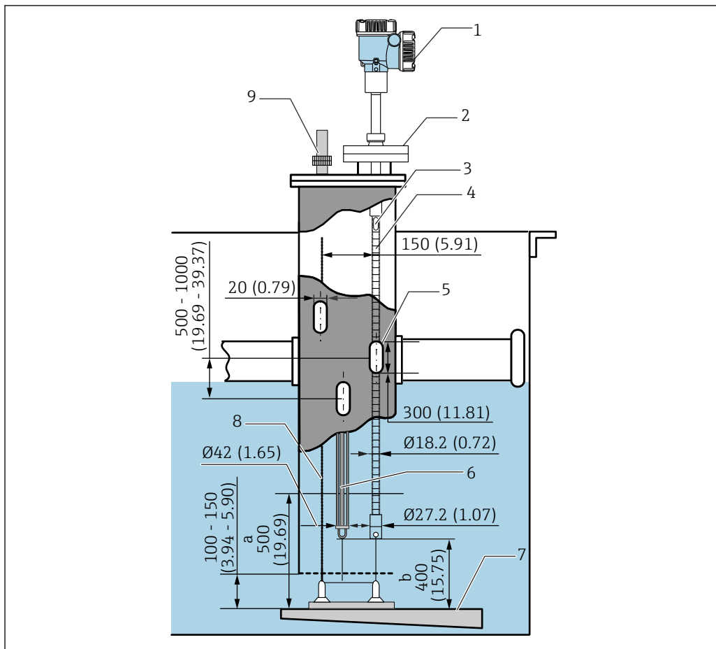
30 Метод с использованием верхнего анкера. Единица измерения мм (дюйм)
