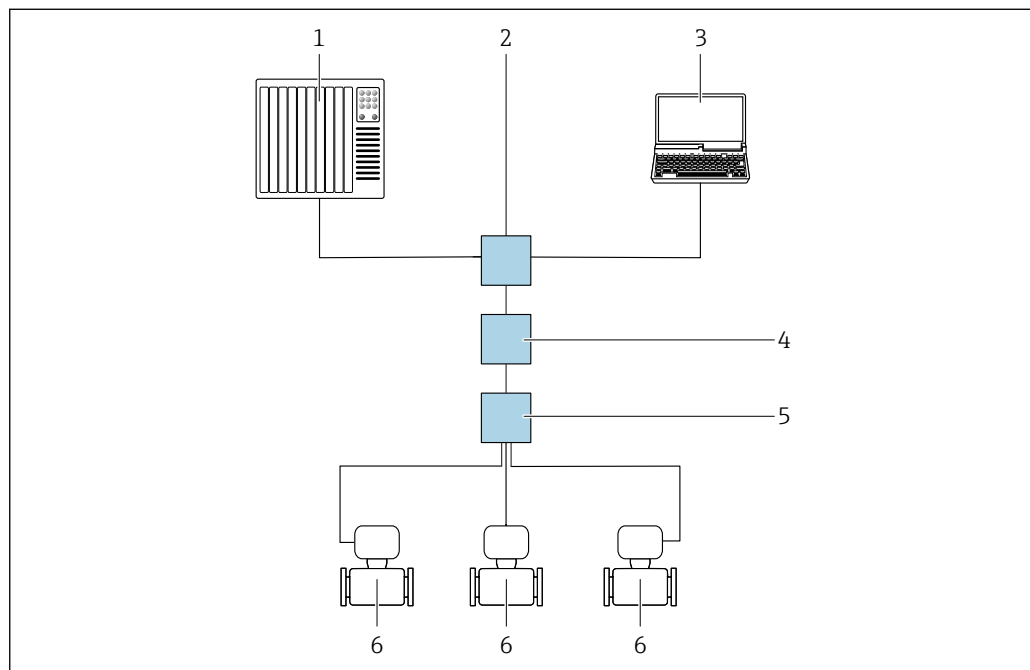
図 25 Modbus TCP over Ethernet-APL プロトコル経由のリモート操作オプション（アクティブ）
