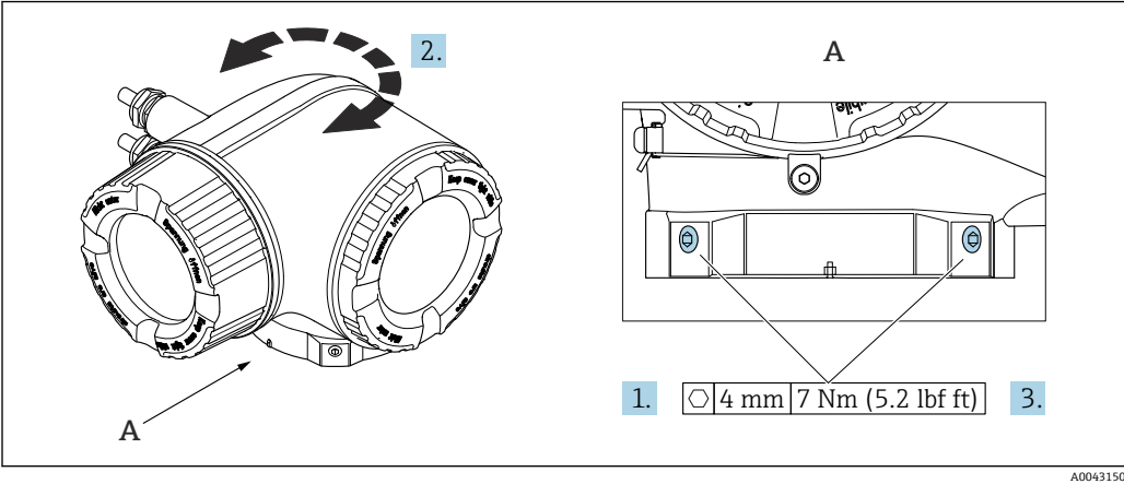
図 11 防爆ハウジング
