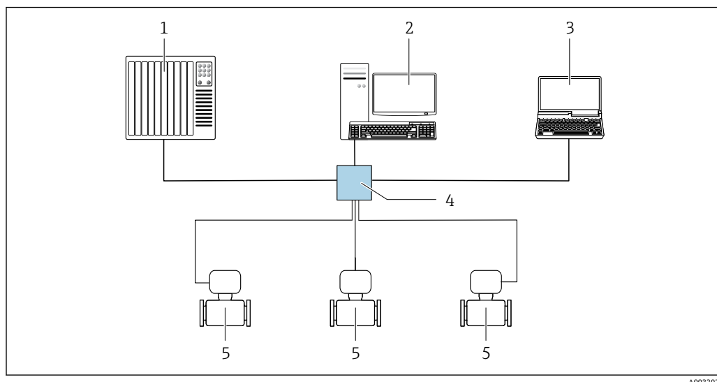
図 26 Modbus TCP over Ethernet - 100 Mbit/s 経由のリモート操作用オプション：スター型トポロジー
