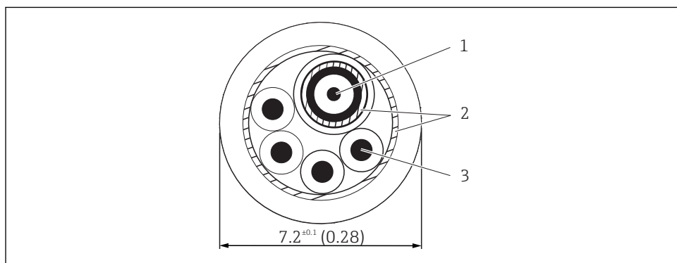
8 Structura cablului de măsurare CYK71, specificații în mm (in)
