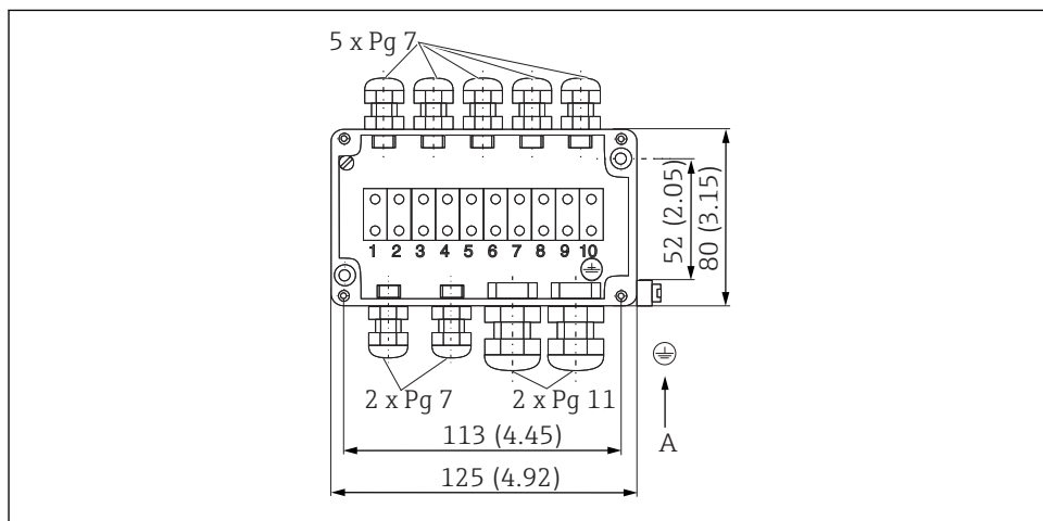
7 Cutie de distribuție VBC cu opțiune de împământare, specificații în mm (in)
