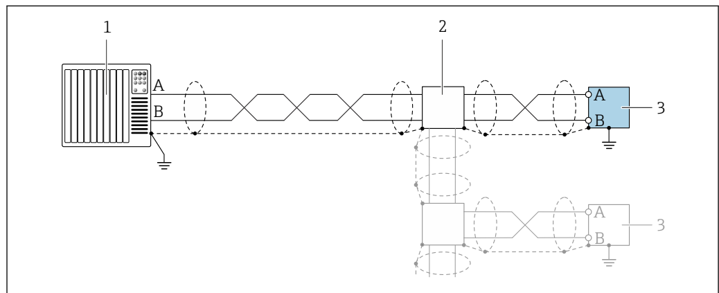
25 Ejemplo de conexión para Modbus RS485
